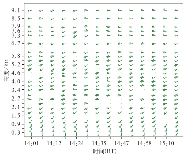
图5 2021年5月10日14:01—15:16吉安雷达风廓线
