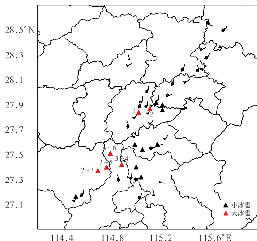
注:红色三角形附近数字为冰雹直径,单位:cm。
