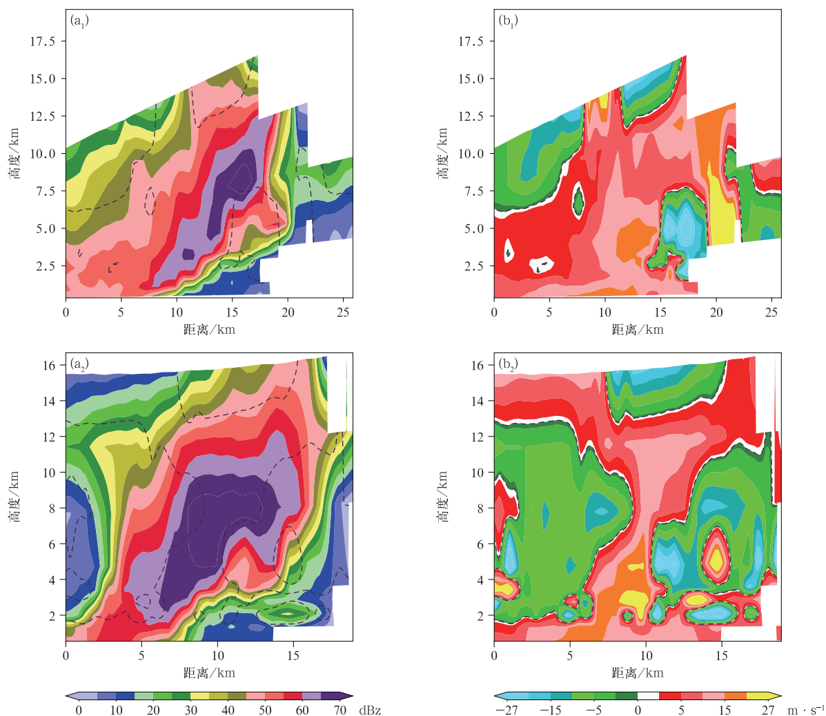
图 9 2021 年 5 月 10 日 15:16 吉安雷达(a)反射率因子和(b)径向速度沿图 8a_1 线段 (a_1, b_1) AB 、 (a_2, b_2) CD 的垂直剖面 Fig. 9 Vertical cross-sections of (a) reflectivity factor and (b) radial velocity along the line (a_1, b_1) AB and (a_2, b_2) CD in Fig. 8a_1 at Ji'an Radar at 15:16 BT 10 May 2021
