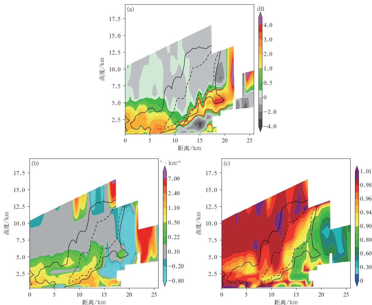
图 11 2021 年 5 月 10 日 15:16 吉安雷达(a) Z_{DR} , (b) K_{DP} , (c)CC 沿图 8a 1 线段 AB 的垂直剖面
