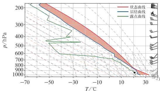
图3 对2021年5月10日08:00南昌站探空进行订正后的14:00探空
