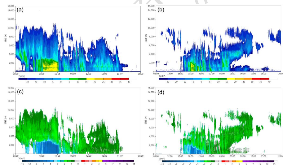
图 9 (a, c)2023 年 11 月 5 日 08:00 至 7 日 08:00 和(b, d)2024 年 2 月 18 日 08:00 至 19 日 20:00 沈阳苏家屯站云雷达(a, b)反射率因子和(c, d)径向速度垂直分布的时间演变
