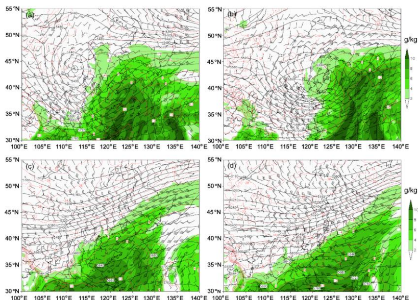
图 3 2023 年 11 月(a)5 日 20:00、(b)6 日 08:00 和 2024 年 2 月(c)18 日 20:00、(d)19 日 08:00 500 hPa 高度场（黑色等值线，单位：gpm），850 hPa 温度场（红色等值线，单位：℃）、风场（风羽）和相对湿度（填色）
