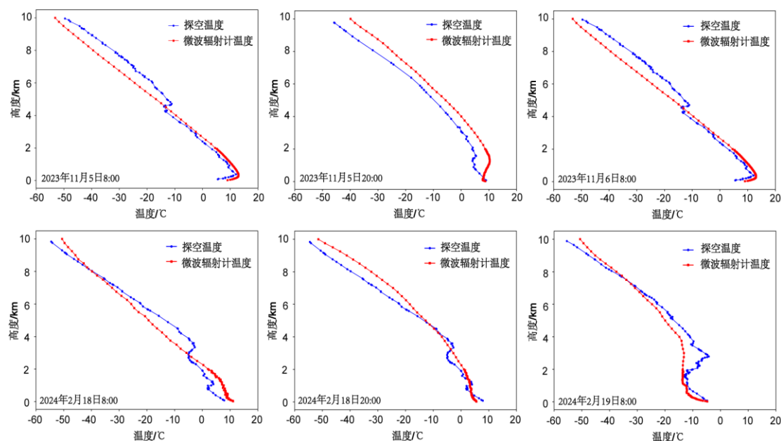
图 7 2023 年 11 月(a)5 日 08:00、(b)5 日 20:00、(c)6 日 08:00 和 2024 年 2 月(d)18 日 08:00、(e)18 日 20:00、(f)19 日 08:00 微波辐射计与探空的温度廓线对比
