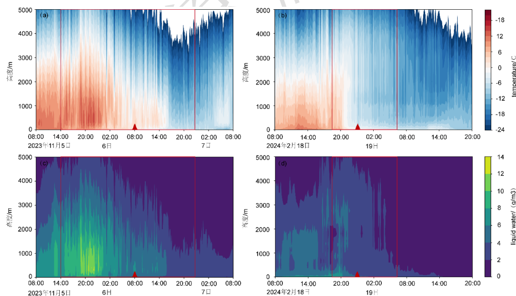
图 8 (a, c)2023 年 11 月 5 日 08:00 至 7 日 08:00 和 (b, d) 2024 年 2 月 18 日 08:00 至 19 日 20:00 苏家屯站微波辐射计反演的 (a, b) 温度和 (c, d) 液态水含量垂直分布的时间演变
