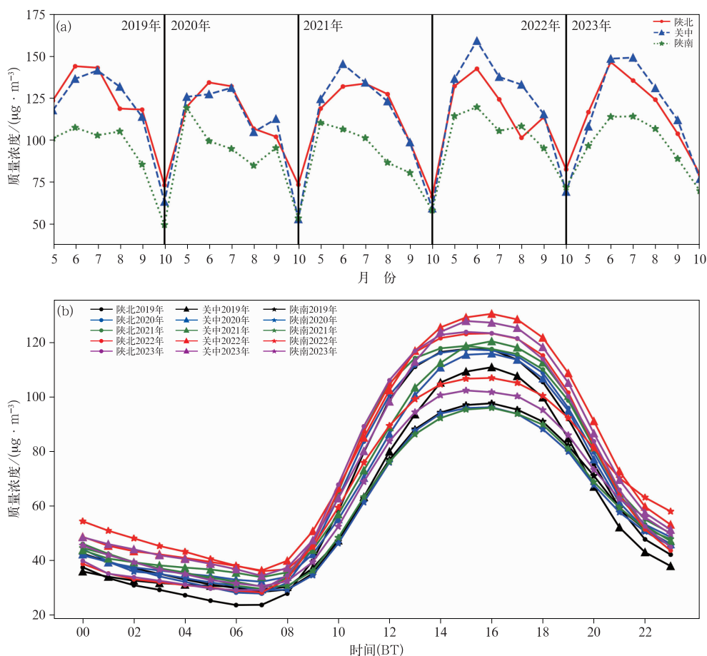
图 2 2019—2023 年暖季陕西近地面 O_3 浓度 (a) 月变化和 (b) 日变化
