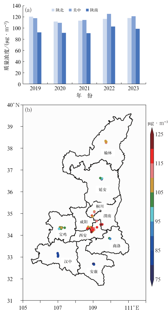
图1 2019—2023年暖季陕西近地面O 3 浓度 (a)逐年变化和(b)年均空间分布
