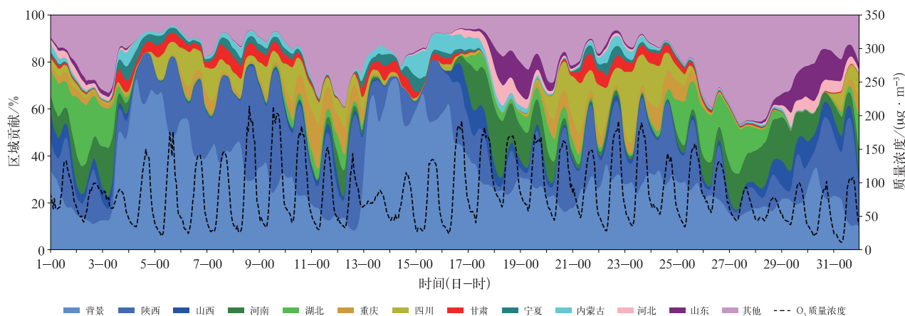
图 7 2023 年 7 月陕西 O 3 来源逐时解析
