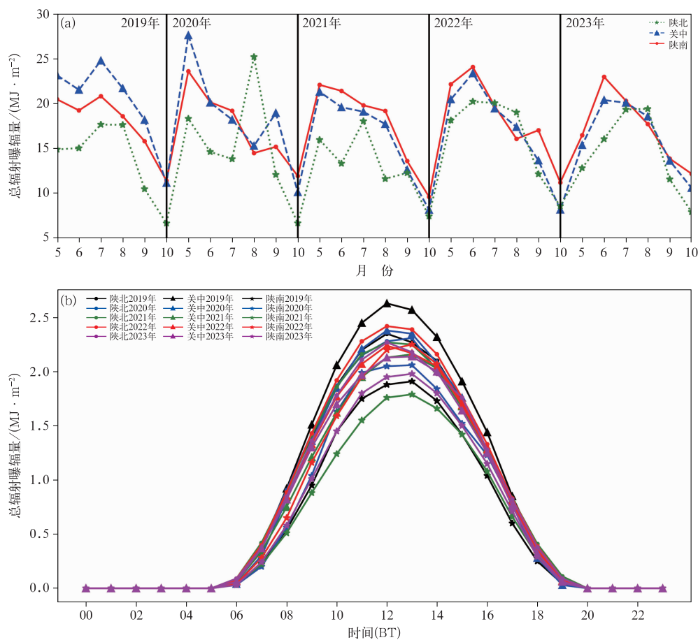
图 4 2019—2023 年暖季陕西总辐射曝辐量(a)月变化和(b)日变化
