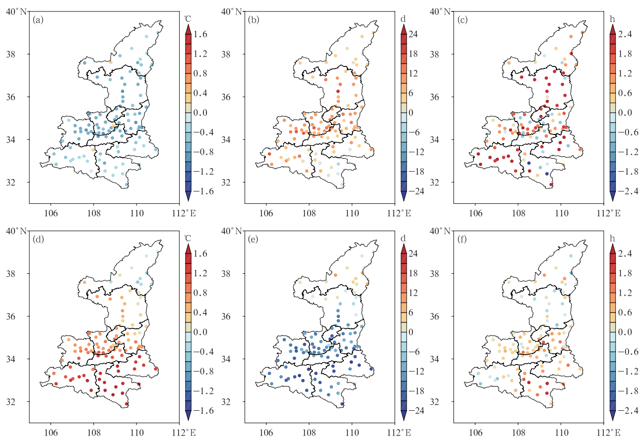
图5 (a~c)2020年和(d~f)2022年暖季陕西(a,d)日最高气温,(b,e)降水日数以及(c,f)日照时数较2019—2023年同期多年平均的差值的空间分布
