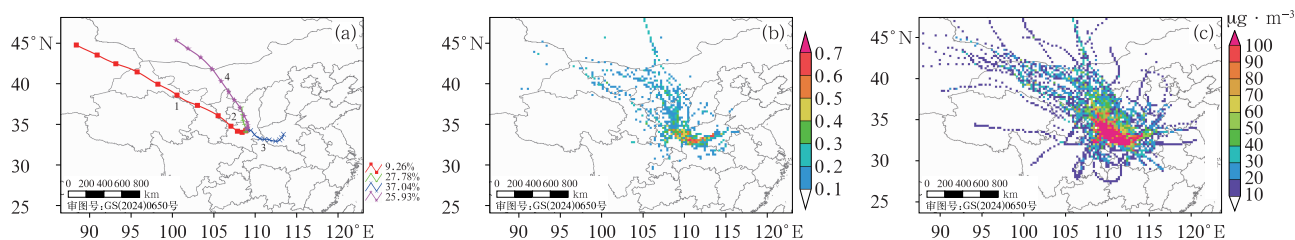
图 8 2023 年暖季西安污染日 O 3 (a)后向轨迹聚类, (b)权重潜在源贡献因子和 (c)加权浓度权重轨迹分布
