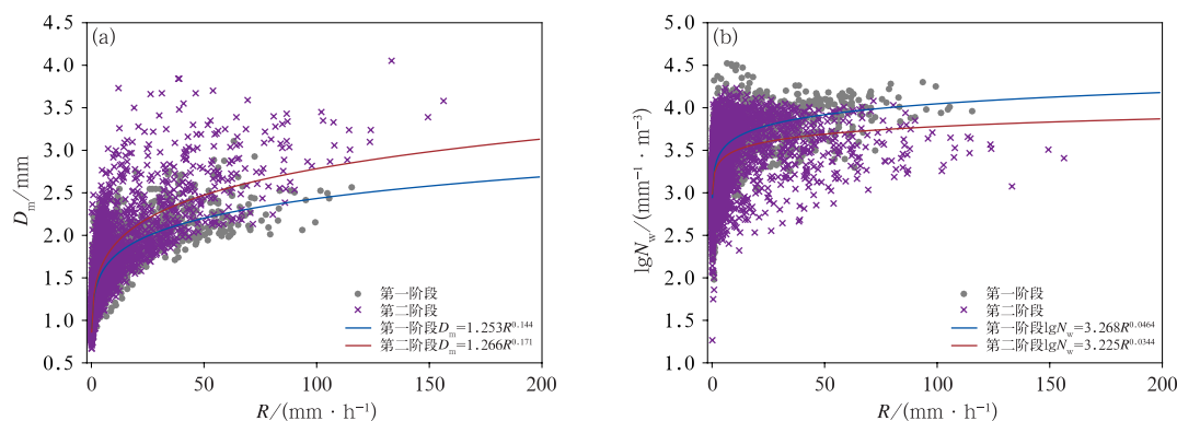
图 10 2023 年 9 月“海葵”残涡影响珠三角过程第一阶段和第二阶段对流降水的 (a) D_m - R 和(b) \lg N_w - R 散点分布及拟合曲线
