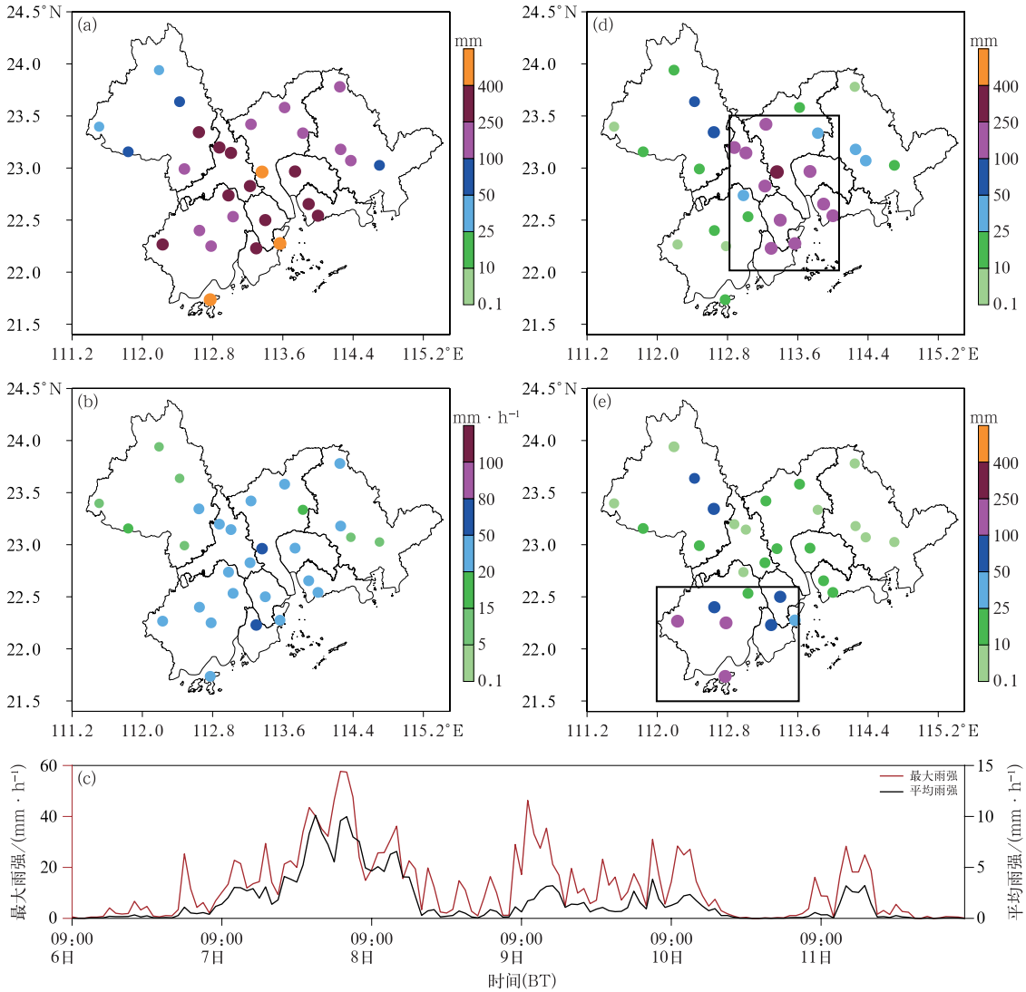
图 2 2023 年 9 月珠三角(a~c)6 日 08:00 至 12 日 08:00(a)累计降雨量和(b)最大雨强的空间分布,
