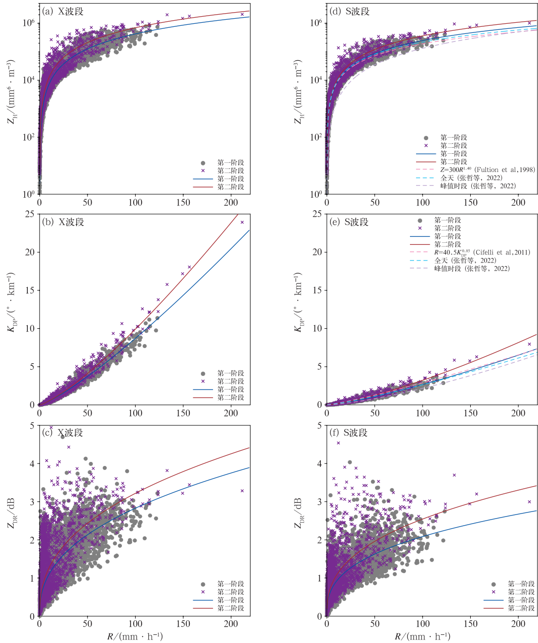
图 11 2023 年 9 月“海葵”残涡影响珠三角过程基于雨滴谱仪的 S/X 波段雷达双偏振参量与雨强的散点图和拟合曲线
