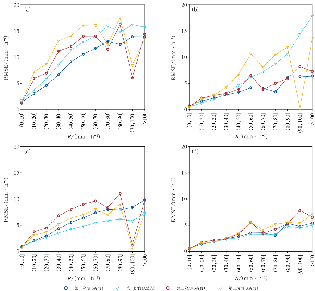
图 12 2023 年 9 月“海葵”残涡影响珠三角过程基于雨滴谱仪的 S/X 波段不同 QPE 算法的 RMSE 随雨强的变化
