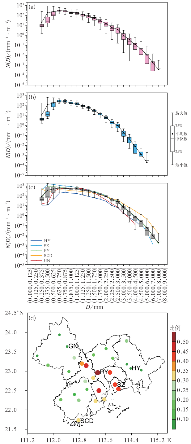
图 6 2023 年 9 月 7 日 08:00 至 11 日 08:00(a~c)不同类型降水平均雨滴谱的箱线分布及其中(d)对流云降水出现频次占总样本(对流云+层状云降水)的比例分布 (a)全部样本,(b)层状云,(c)对流云 Fig. 6 (a~c) Boxplots of average raindrop spectra of different rainfall types and (d) distribution of the proportion of convective cloud rainfall frequency to the total samples (convective cloud + stratiform cloud) from 08:00 BT 7 to 08:00 BT 11 September 2023 (a) all samples, (b) stratiform cloud, (c) convective cloud
