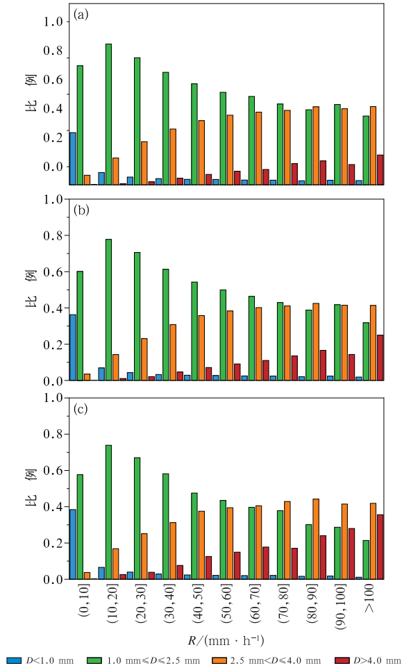
图 8 2023 年 9 月“海葵”残涡影响珠三角过程不同尺度雨滴粒径( D )对雨强( R )的贡献比例 (a)所有样本,(b)第一阶段,(c)第二阶段
