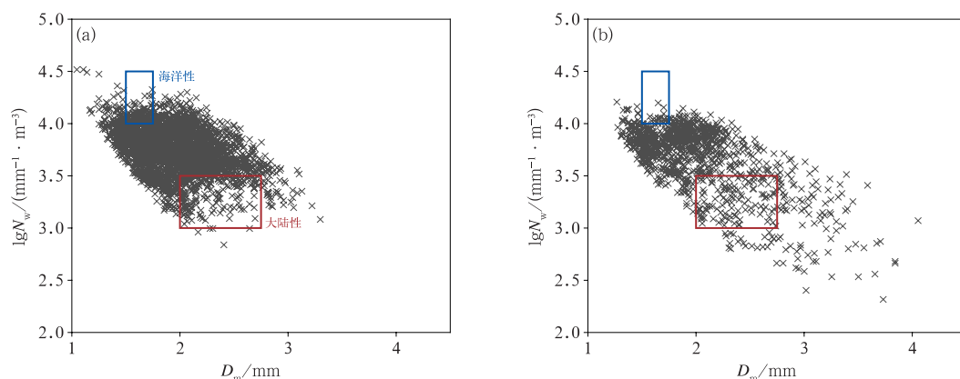
图 9 2023 年 9 月“海葵”残涡影响珠三角过程(a)第一阶段、 (b)第二阶段关键区域对流降水的 D_m - \lg N_w 散点分布
