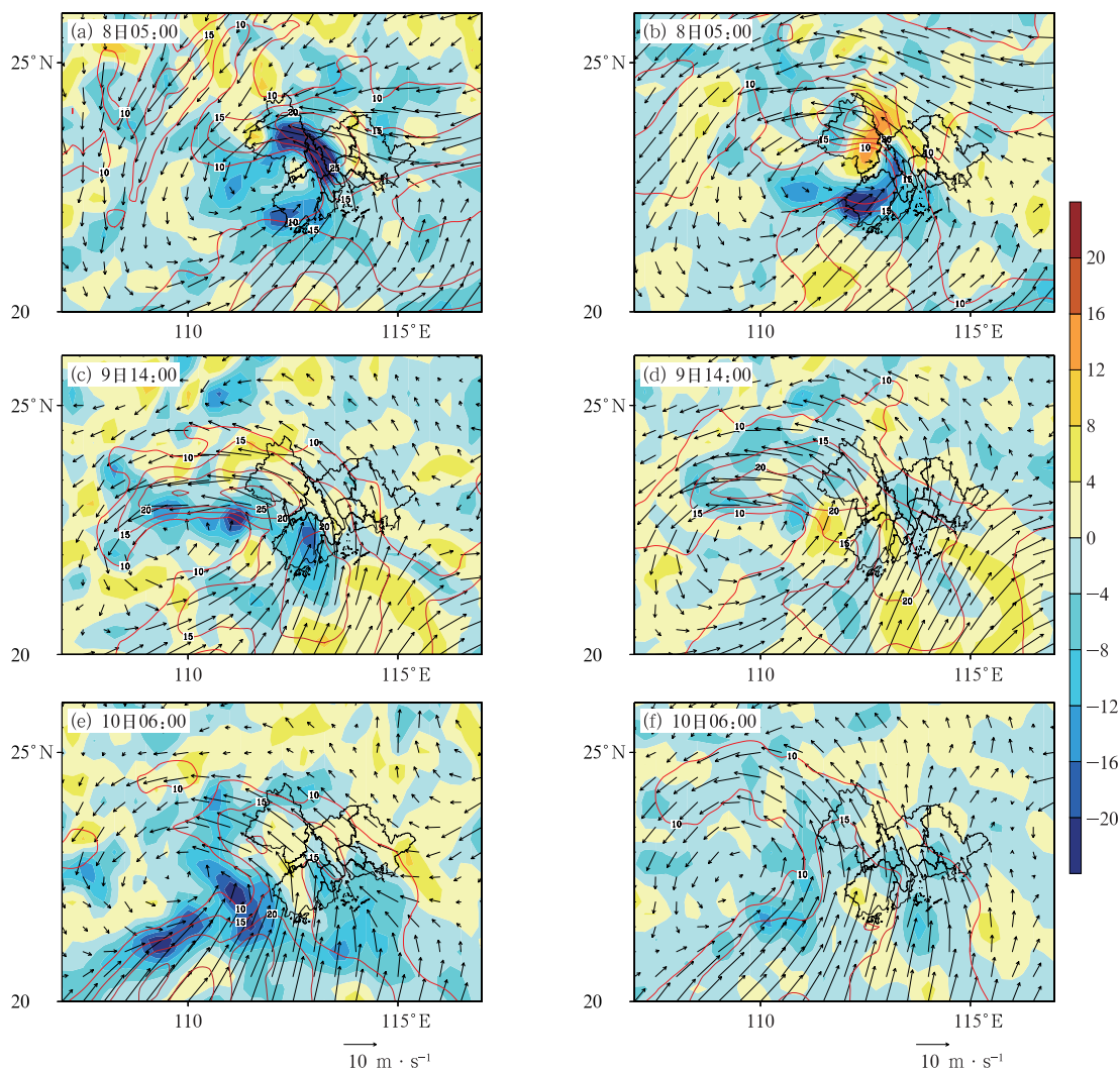
图 4 2023 年 9 月“海葵”残涡影响珠三角过程(a,b)第一阶段,(c~f)第二阶段风场(风矢)、水汽通量(等值线,单位: \text{g} \cdot \text{cm}^{-1} \cdot \text{hPa}^{-1} \cdot \text{s}^{-1} )和水汽通量散度(填色,单位: 10^{-7} \text{g} \cdot \text{cm}^{-2} \cdot \text{hPa}^{-1} \cdot \text{s}^{-1} ) (a,c,e)925 hPa,(b,d,f)850 hPa
