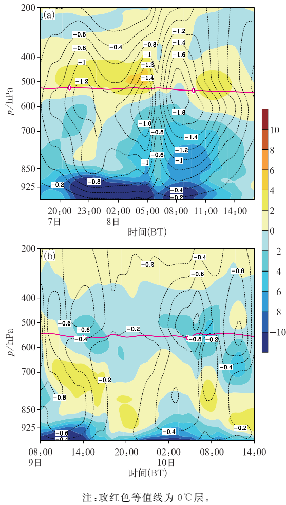
图 5 2023 年 9 月“海葵”残涡影响珠三角过程 (a)第一阶段,(b)第二阶段关键区域的 垂直速度(等值线,单位: \text{Pa} \cdot \text{s}^{-1} )和 水汽通量散度(填色,单位: 10^{-7} \text{g} \cdot \text{cm}^{-2} \cdot \text{hPa}^{-1} \cdot \text{s}^{-1} ) 垂直分布随时间的变化
