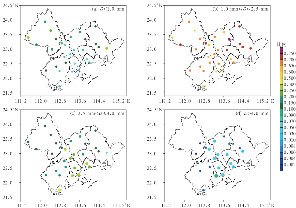
图 7 2023 年 9 月“海葵”残涡影响珠三角过程不同尺度雨滴粒径( D )对总降雨量贡献比例的空间分布
