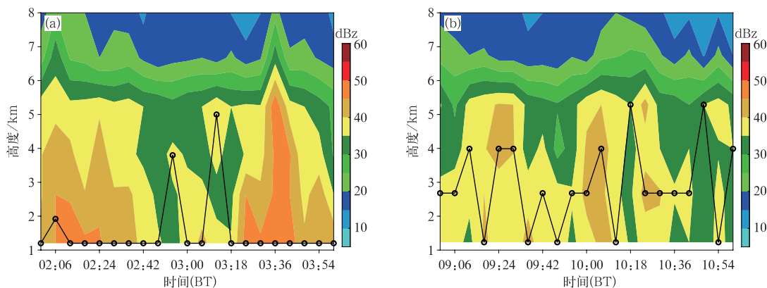
图 3 2023 年 9 月“海葵”残涡影响珠三角过程的单站反射率因子垂直分布(填色)
