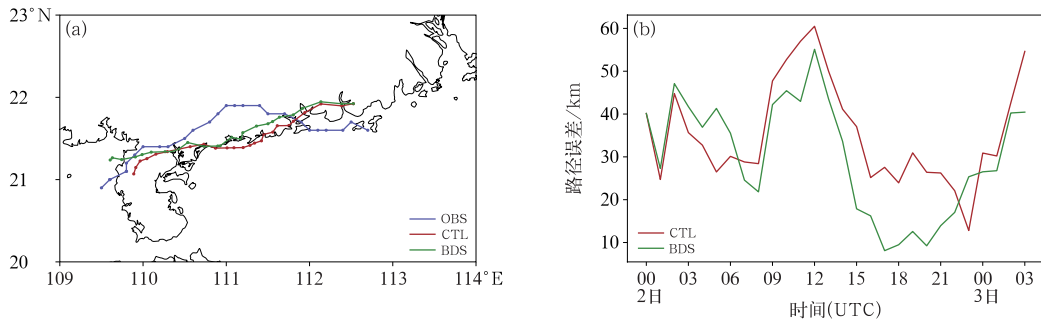
图 6 2023 年台风“苏拉”(a)观测和模拟的台风路径,(b)9月2日00时起报的两组同化试验的台风路径预报误差
