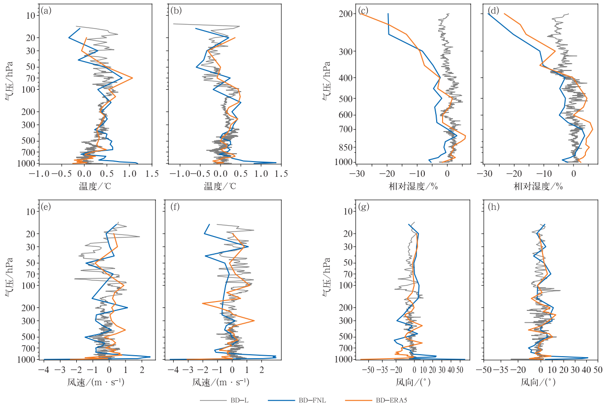
图 3 2023 年 8 月 31 日 00 时至 9 月 6 日 00 时(a,c,e,g)00 时和(b,d,f,h)12 时北斗探空上升段与 L 波段探空、
