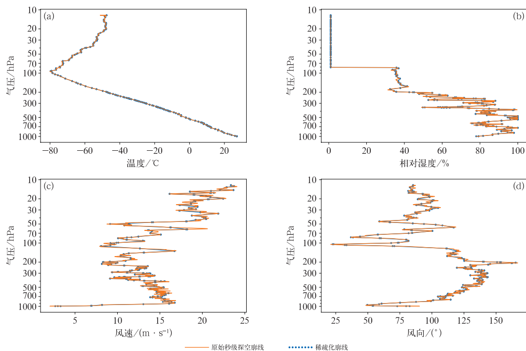
图 5 2023 年 9 月 2 日 00 时河源站上升段(a)温度,(b)相对湿度,(c)风速,(d)风向的原始秒级探空廓线及稀疏化廓线
