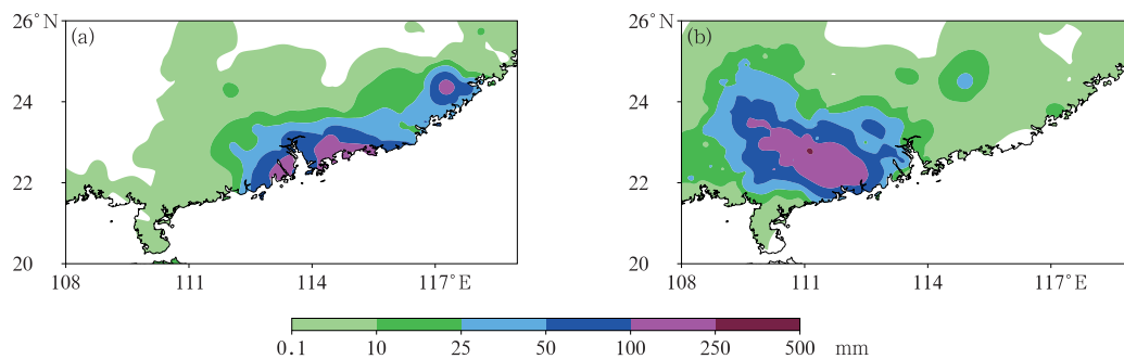
图1 2023年9月(a)1日00时至2日00时,(b)2日00时至3日00时台风“苏拉”(2309号)24 h累计降水量
