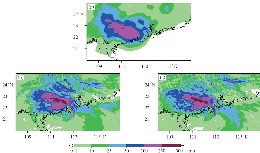
图 8 2023 年 9 月 2 日 00 时至 3 日 00 时台风“苏拉”(a)观测,以及(b)CTL 和(c)BDS 预报的 24 h 累计降水量
