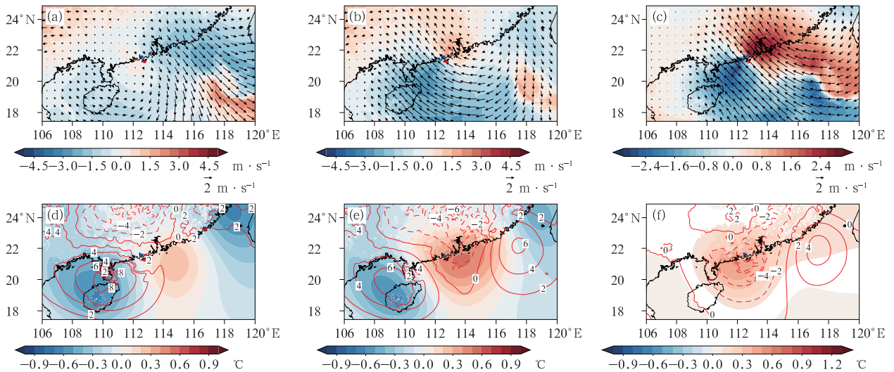
注: 蓝色圆点为 CTL 台风位置, 红色圆点为观测台风位置; 图 a 和 b 中的风矢表示纬向风与经向风分析增量的合成风场, 填色表示风速大小的分析增量。
