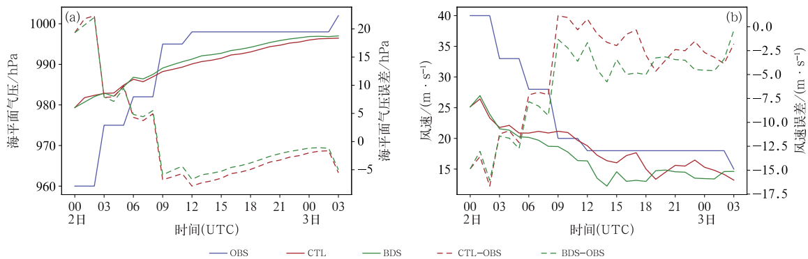
图 7 2023 年台风“苏拉”观测及 9 月 2 日 00 时起报的两组同化试验的 (a)台风中心附近海平面最低气压及其预报误差,(b)最大风速及其预报误差
