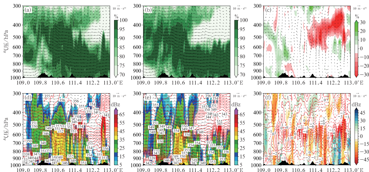
图 13 2023 年 9 月 2 日 12 时沿 23.75^{\circ}\text{N} 的(a~c)相对湿度(填色)和风场(风矢),以及(d~f)雷达反射率因子(填色)、相当位温(红色等值线,单位:K)和风场(风矢)的垂直剖面 (a,d)CTL, (b,e)BDS, (c,f)BDS 与 CTL 之差
