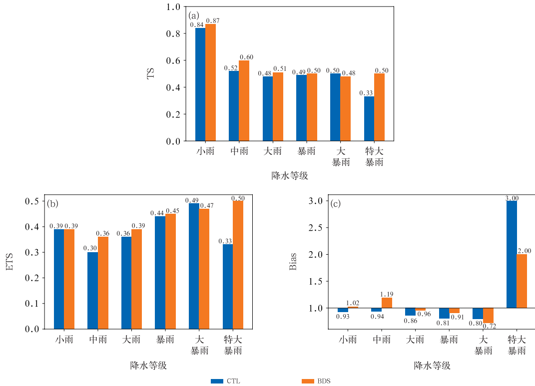
图 9 2023 年 9 月 2 日 00 时至 3 日 00 时台风“苏拉”两组同化试验预报的 24 h
