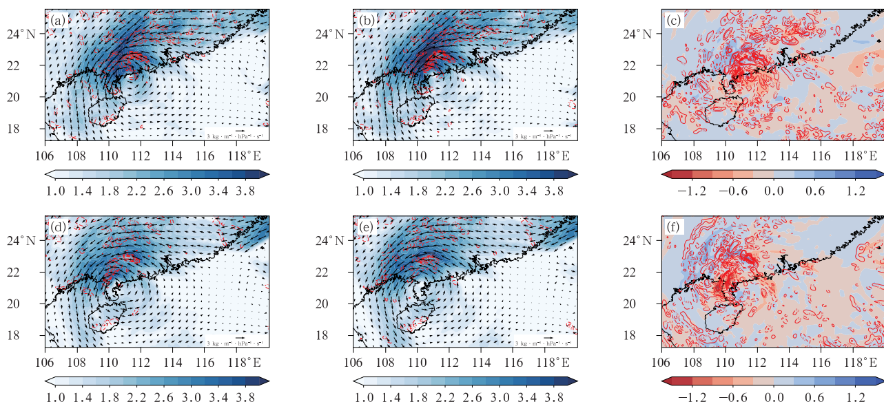
图 11 2023 年 9 月 2 日(a~c)12 时和(d~f)18 时 850 hPa 水汽通量(矢量和填色,单位: \text{kg} \cdot \text{m}^{-1} \cdot \text{hPa}^{-1} \cdot \text{s}^{-1} )及水汽通量散度(红色等值线,单位: 10^{-5} \text{ kg} \cdot \text{m}^{-2} \cdot \text{hPa}^{-1} \cdot \text{s}^{-1} )
