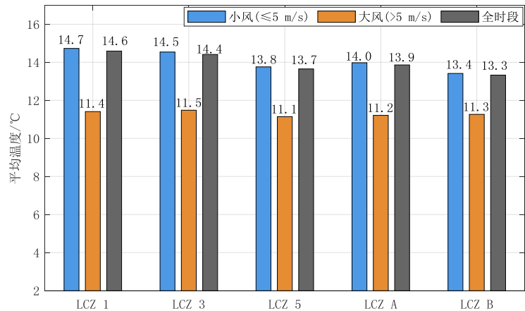
图 9 2010—2021 年北京五环内不同风速条件下各局地气候类型平均气温对比
