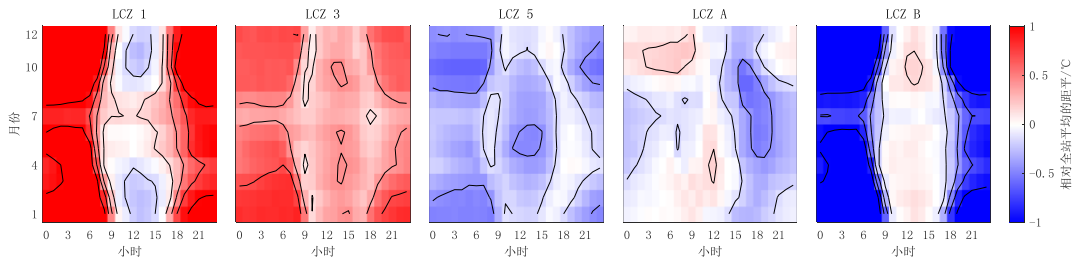
图 6 2010—2021 年北京五环内不同局地气候类型相对 37 个站平均的气温月-时距平分布
