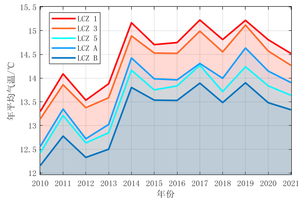
图 3 2010—2021 年北京五环内不同局地气候类型年平均气温的年际变化
