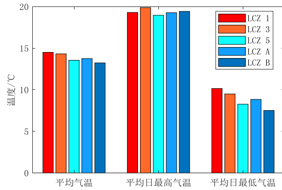
图 2 2010—2021 年北京五环内不同局地气候类型的气温特征对比
