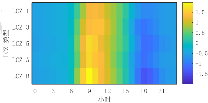
图 7 2010—2021 年北京五环内不同局地气候类型气温逐小时变化率
