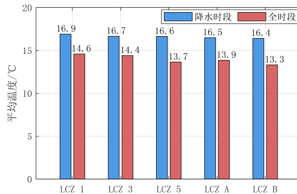
图 8 2010—2021 年北京五环内不同局地气候类型降水时段与全时段的平均气温对比
