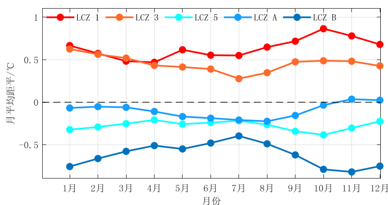
图 4 2010—2021 年北京五环内不同局地气候类型的月平均气温距平
