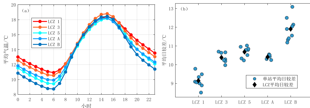
图 5 2010—2021 年北京五环内不同局地气候类型的 (a) 平均气温日变化与 (b) 日较差特征
