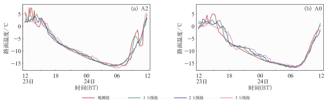
图 5 2023 年 1 月 23—24 日(a)A2 和(b)A0 交通气象站极端低温个例的路面温度观测值与模型预报值
