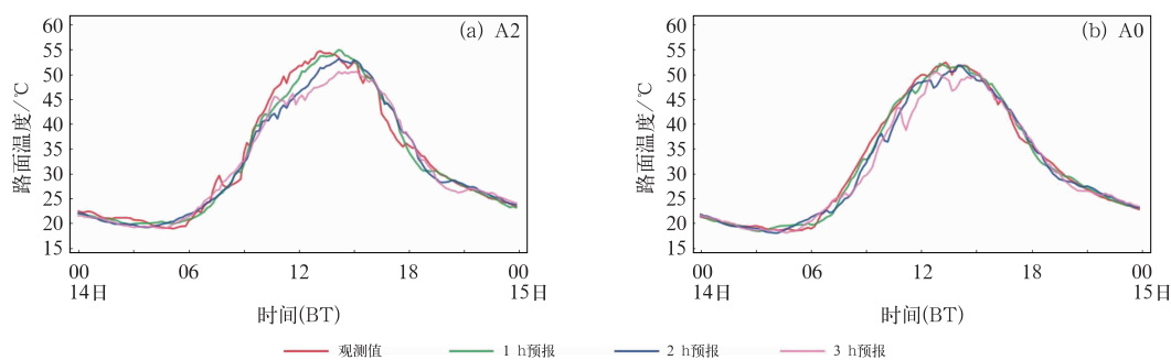
图 6 2023 年 5 月 14—15 日(a)A2 和(b)A0 交通气象站极端高温个例的路面温度观测值与模型预报值
