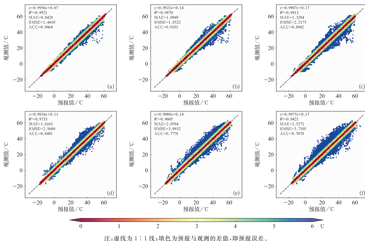
图 4 2023 年交通气象站(a~c)A1 和(d~f)A8 模型预报值与观测值散点分布 (a,d)1 h 预报,(b,e)2 h 预报,(c,f)3 h 预报
