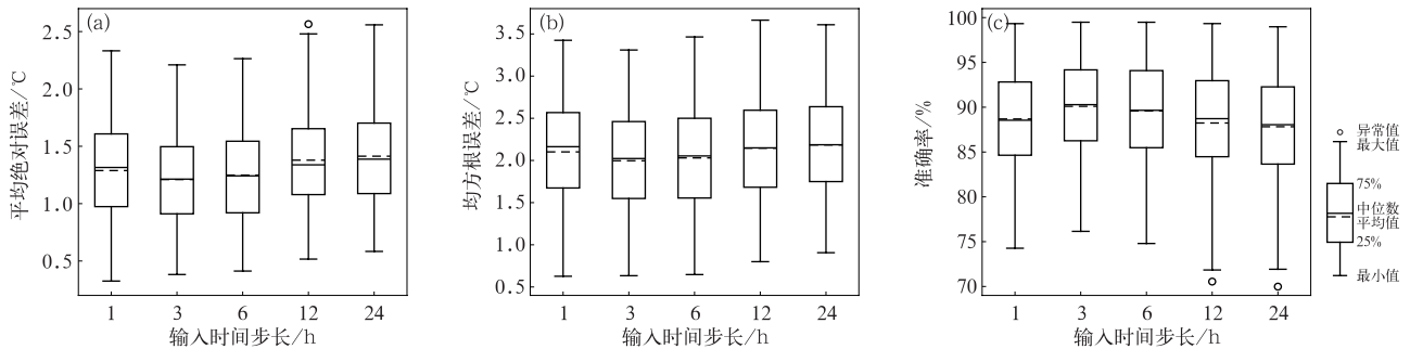
图 2 不同输入时间步长模型对 2023 年路面温度的预报能力评估
