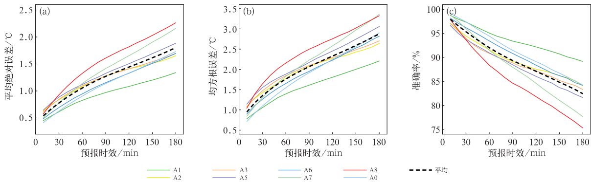
图 3 2023 年 8 个交通气象站模型预报能力评估
