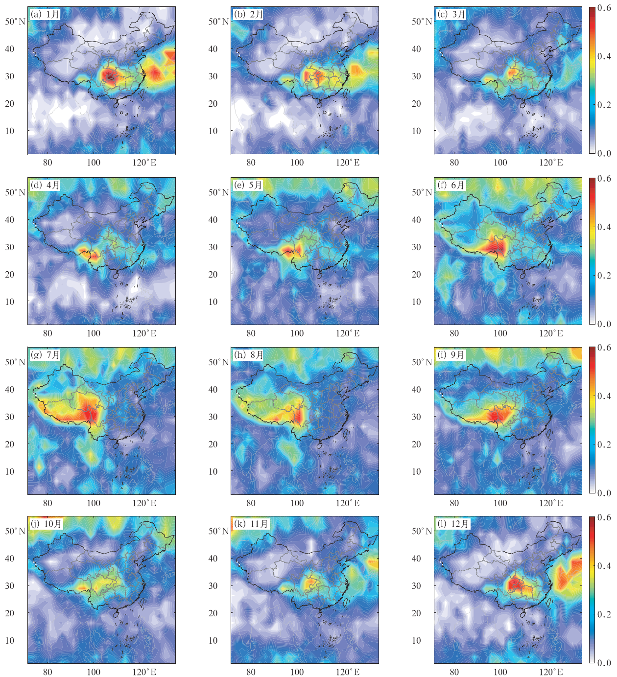
图 4 2006—2019 年过冷积状云月平均出现频率的空间分布
