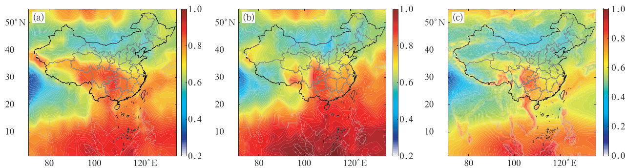
图 1 (a,b)由 CloudSat-CALIPSO 统计计算的 2006—2019 年(a)白天和(b)夜间平均总云出现频率, (c)由 ERA5 统计得到的 2006—2019 年白天平均总云量对比
