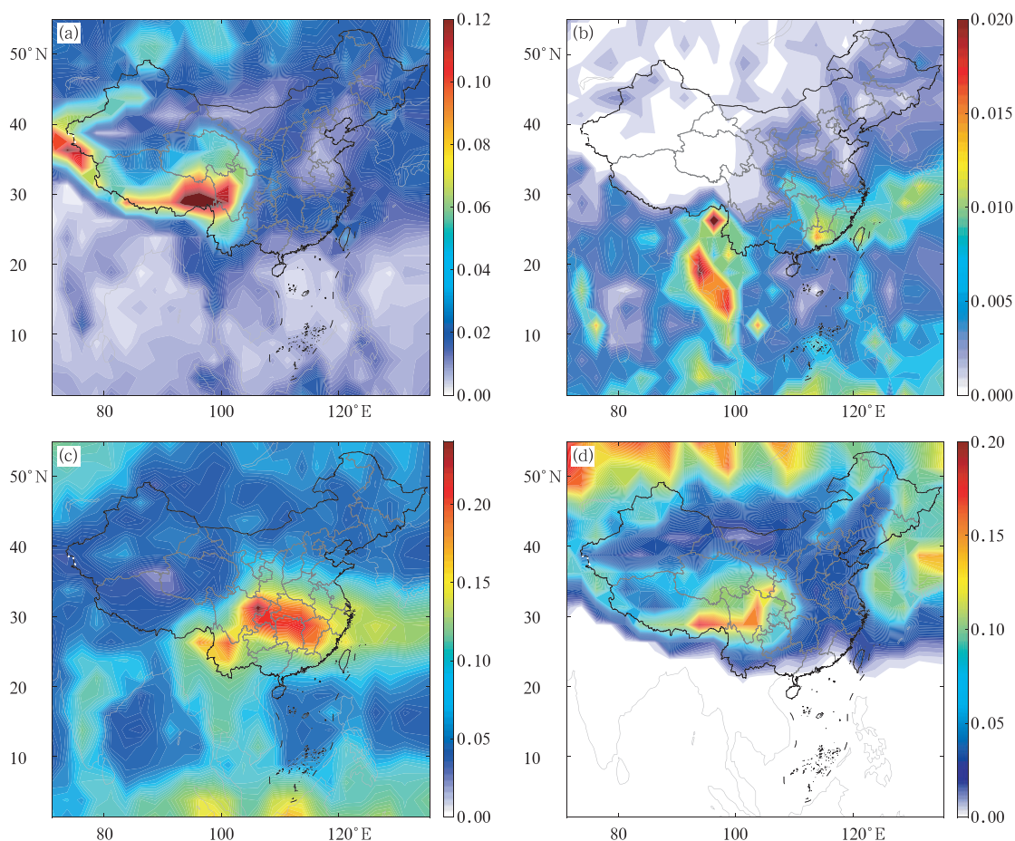
图 3 2006—2019 年(a)过冷积云,(b)过冷深对流,(c)过冷高积云及 (d)过冷层积云平均出现频率的空间分布
