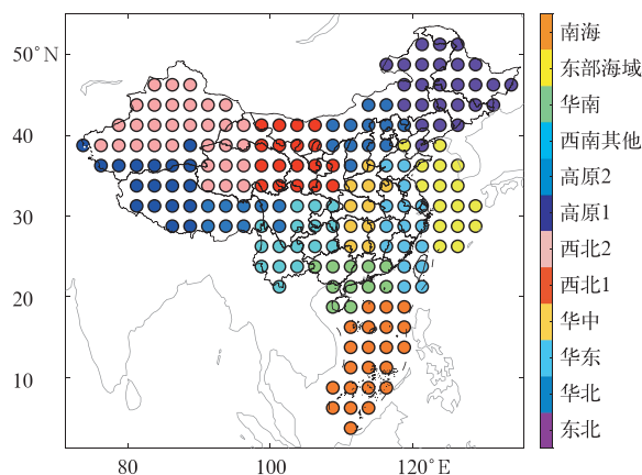
图 5 用于统计不同区域云出现频率年际变化趋势的格点划分
