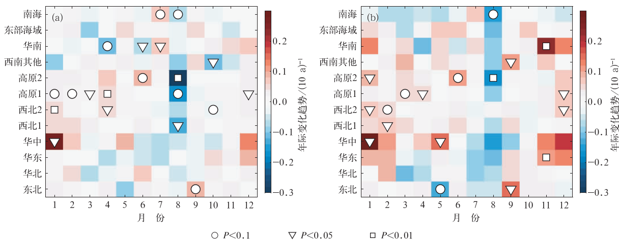
图 6 2006—2019 年不同区域(a)过冷积状云和(b)积状云出现频率的年际变化趋势及显著性水平检验结果
