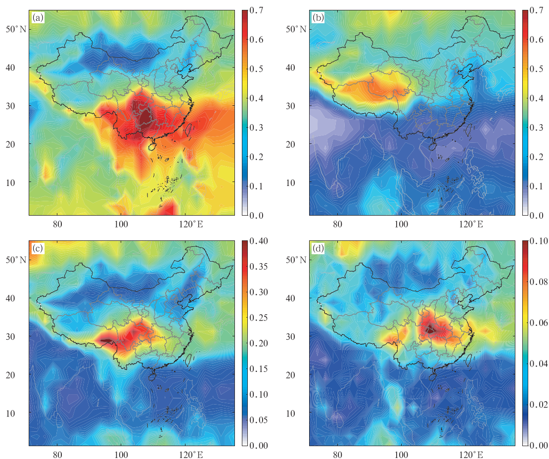
图 2 2006—2019 年(a)积状云,(b)层状云,(c)过冷积状云及(d)过冷层状云平均出现频率的空间分布
