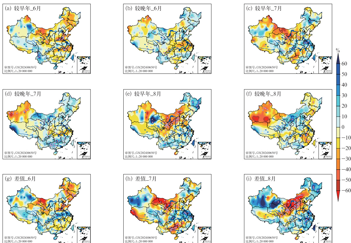
图 3 1961—2023 年厄尔尼诺年 6 月、7 月和 8 月降水量距平百分率合成
