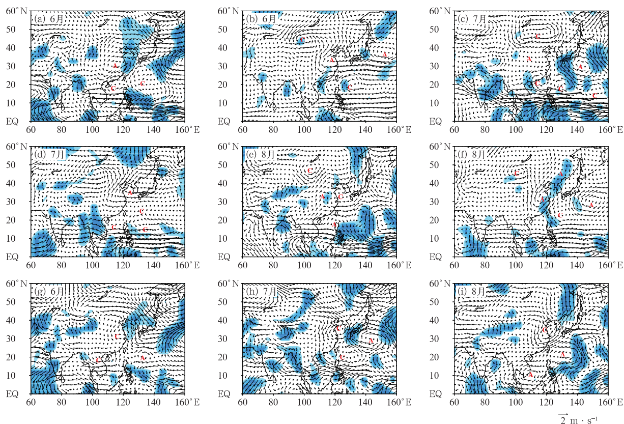
图 5 1961—2023 年厄尔尼诺年 6 月、7 月和 8 月 850 hPa 风场距平合成 (a, c, e) 开始较早年, (b, d, f) 开始较晚年, (g~i) 早晚年差值
