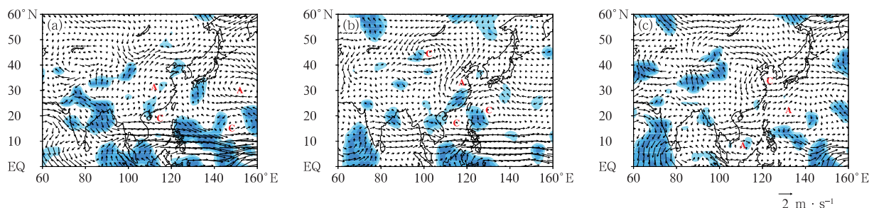
图 4 1961—2023 年厄尔尼诺年夏季 850 hPa 风场距平合成
