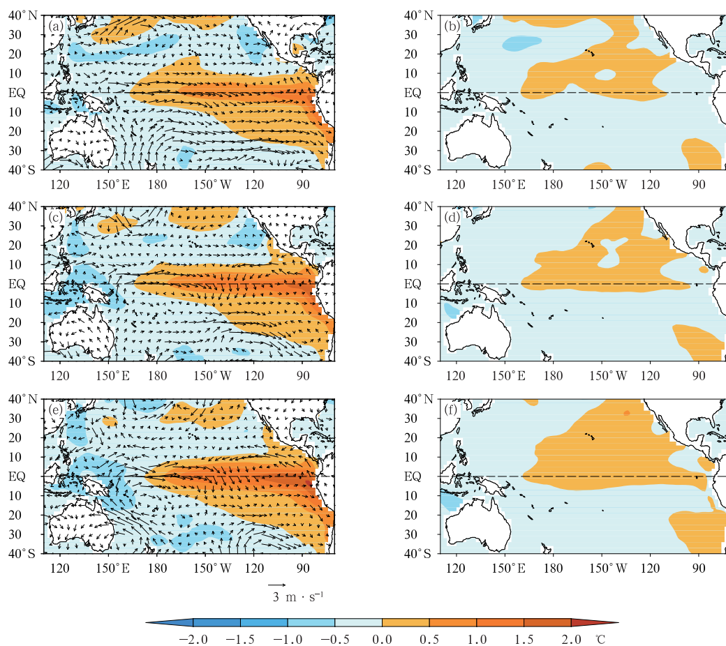
图1 1961—2023年厄尔尼诺开始(a,c,e)较早年和(b,d,f)较晚年对应的(a,b)6月、(c,d)7月、(e,f)8月SSTA(填色)和(a,c,e)850 hPa风场差值(风矢)
