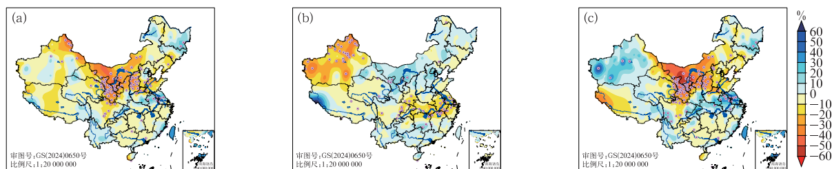
图 2 1961—2023 年厄尔尼诺年夏季降水量距平百分率合成
