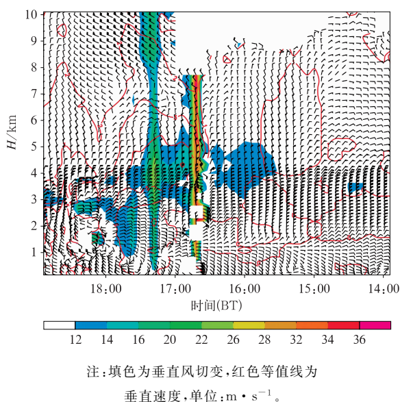
图 5 2020 年 8 月 27 日延庆垂直风廓线(风羽)时间-高度变化
