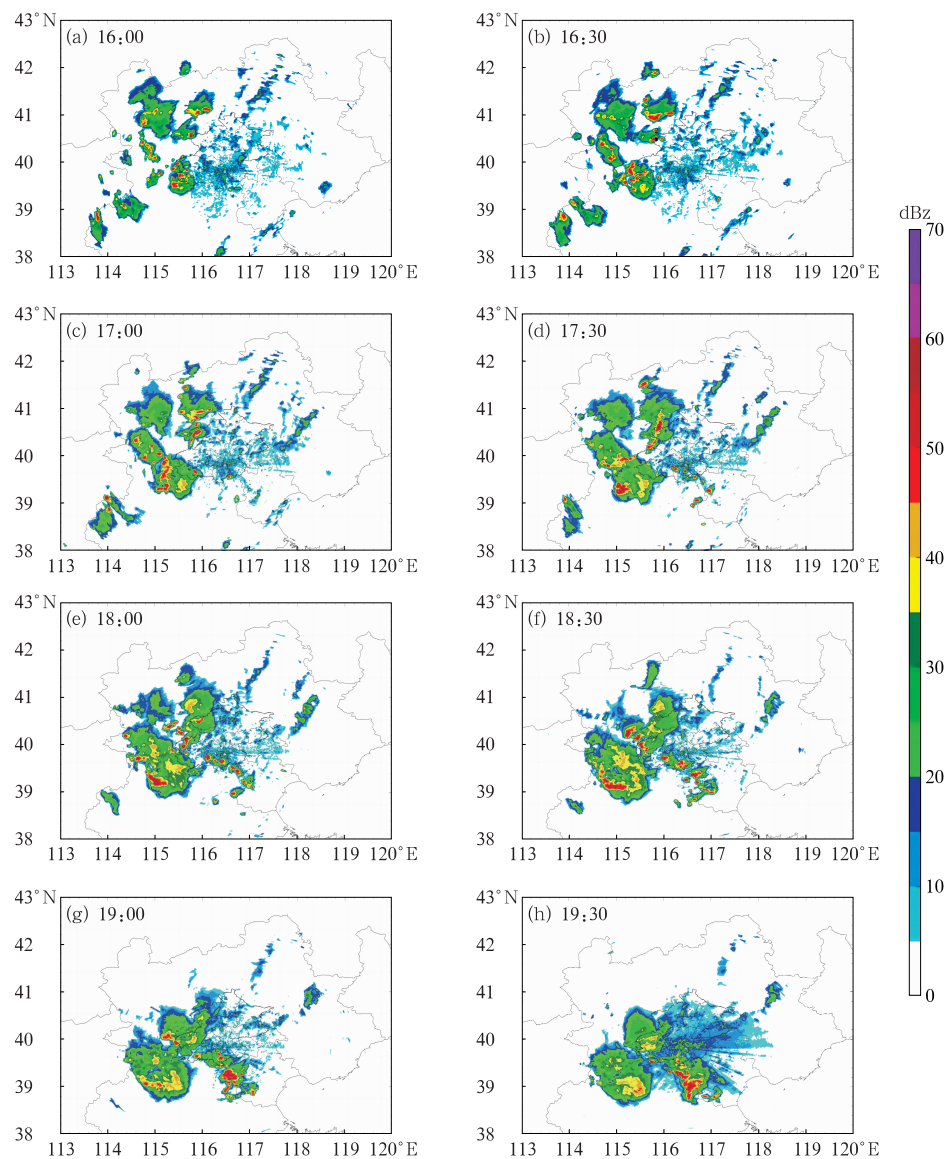
图 3 2020 年 8 月 27 日 16:00—19:30 逐 30 min 的雷达回波演变 Fig. 3 Evolution of radar echoes every 30 min from 16:00 BT to 19:30 BT 27 August 2020
