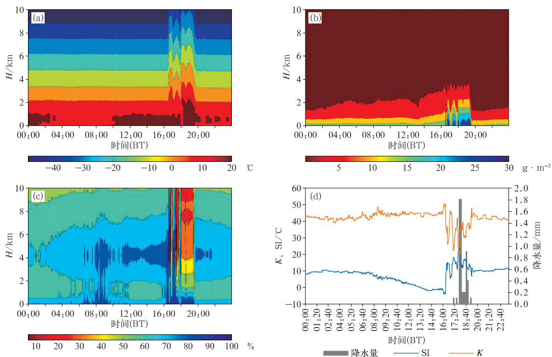
图 4 2020 年 8 月 27 日延庆微波辐射计的(a)温度,(b)水汽密度, (c)相对湿度的时间-高度变化;(d)K 指数、SI 指数、降水量随时间的变化
