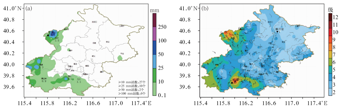
图 2 2020 年 8 月 27 日 15:00—21:00 北京地区(a)累计降水量,(b)地面极大风(风羽)和风力(填色)
