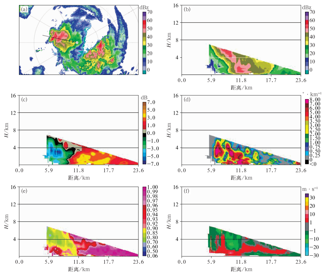
图 8 2020 年 8 月 27 日 18:30 北京房山 X 波段雷达(a)组合反射率因子,(b~f)沿图 a 中黑线的
