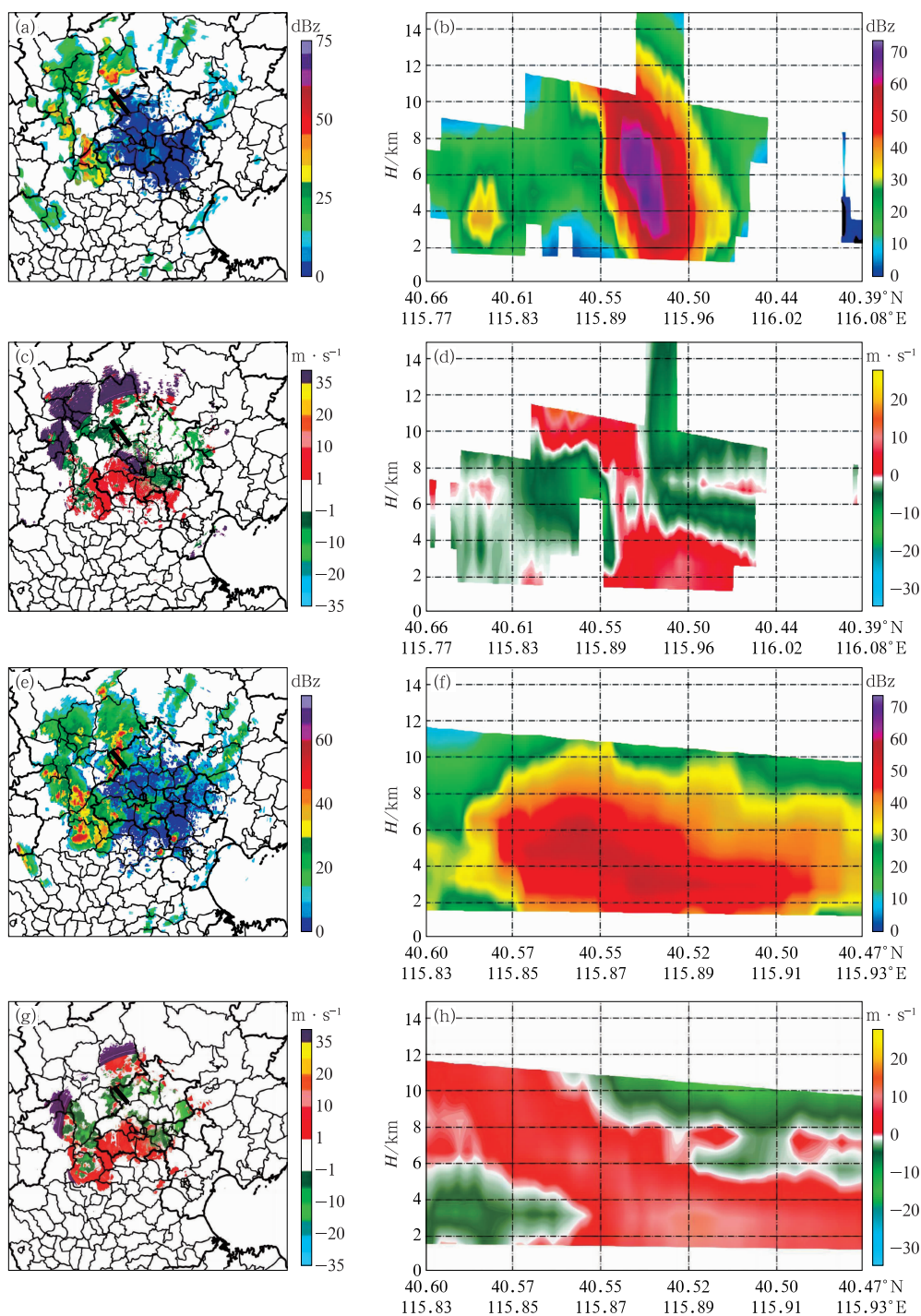
图 6 2020 年 8 月 27 日 (a~d) 16:48, (e~h) 17:18 北京 S 波段雷达 (a, e) 组合反射率因子, (b, f) 分别沿图 6a, 6e 中延庆强回波中心 (黑色实线) 的反射率因子剖面, (c, g) 2.4° 仰角径向速度, (d, h) 分别沿图 6c, 6g 中延庆强回波中心 (黑色实线) 的径向速度剖面 Fig. 6 (a, e) Composite reflectivity factor, (b, f) reflectivity factor cross-section along the strong echo center (black solid line) in Yanqing in Fig. 6a and Fig. 6e, (c, g) radial velocity at 2.4° elevation, (d, h) radial velocity cross-section along the strong echo center (black solid line) in Yanqing in Fig. 6c and Fig. 6g of S-band radar in Beijing at (a—d) 16:48 BT and (e—h) 17:18 BT 27 August 2020
