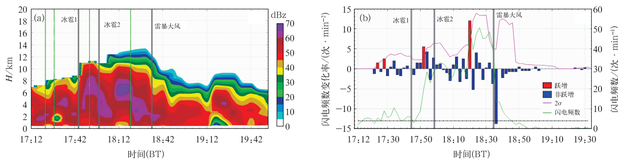
图 9 2020 年 8 月 27 日房山追踪的强雷暴(a)沿雷暴中心的反射率因子(填色)
