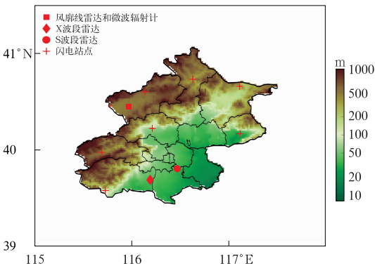
图 1 北京多源高频次探测设备分布和地形(填色)
