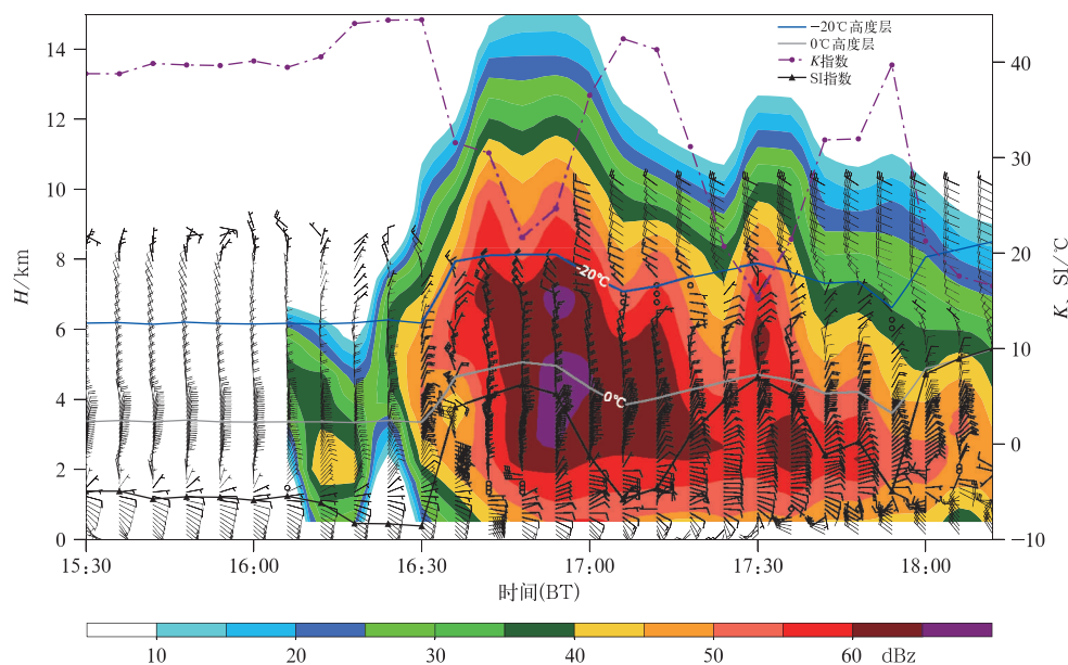
图 10 2020 年 8 月 27 日 15:30—18:10 沿延庆追踪的强雷暴中心的反射率因子(填色)、 -20^{\circ}\text{C} 和 0^{\circ}\text{C} 高度层、延庆风廓线雷达观测的风场(风羽)以及 K 指数和 SI 指数随时间的变化
