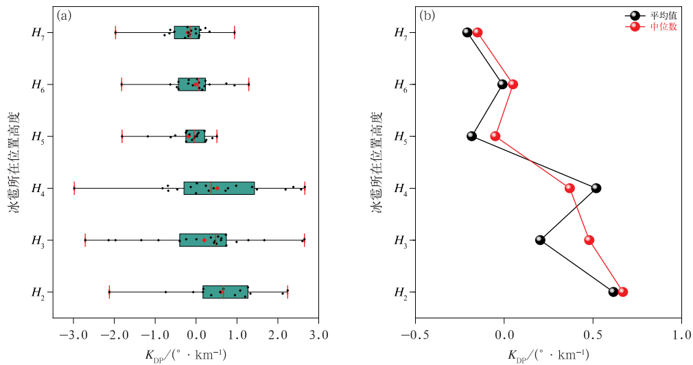
图 2 K_{DP} (a) 在各个高度的分布和 (b) 平均值、中位数随高度变化趋势 Fig. 2 (a) Distribution of K_{DP} at different heights and (b) trend of K_{DP} 's mean and median values with altitude
