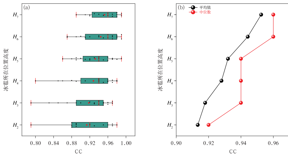
图 3 CC (a) 在各个高度的分布和 (b) 平均值、中位数随高度变化趋势 Fig. 3 (a) Distribution of CC at different heights and (b) trend of CC's mean and median values with altitude
