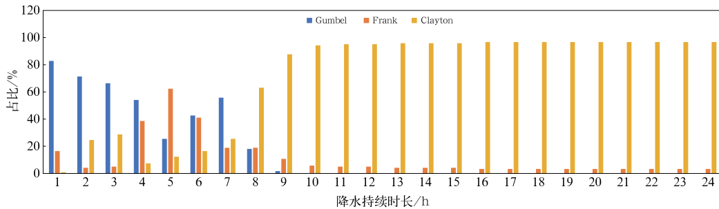
图 7 1966—2023 年山东强降水不同降水持续时长的最优拟合 Copula 联合分布函数类型占比
