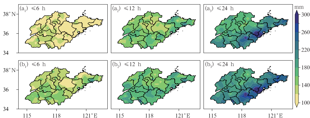
图 11 山东不同降水持续时长在(a)30 年一遇和(b)60 年一遇联合重现期下的降水量阈值
