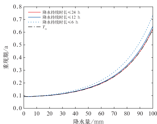
图 9 1966—2023 年崂山站强降水不同降水持续时长的联合重现期与单变量重现期对比
