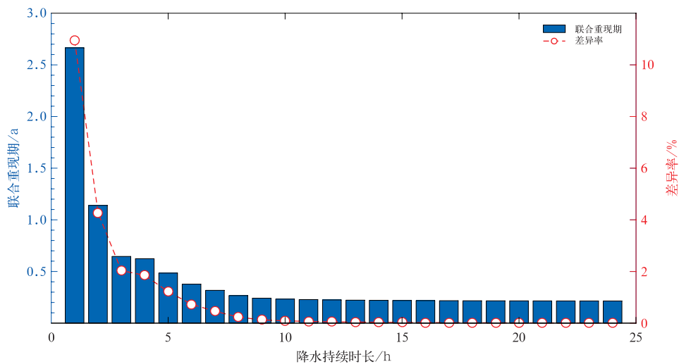
图 8 1966—2023 年山东强降水不同降水持续时长的联合重现期及差异率
