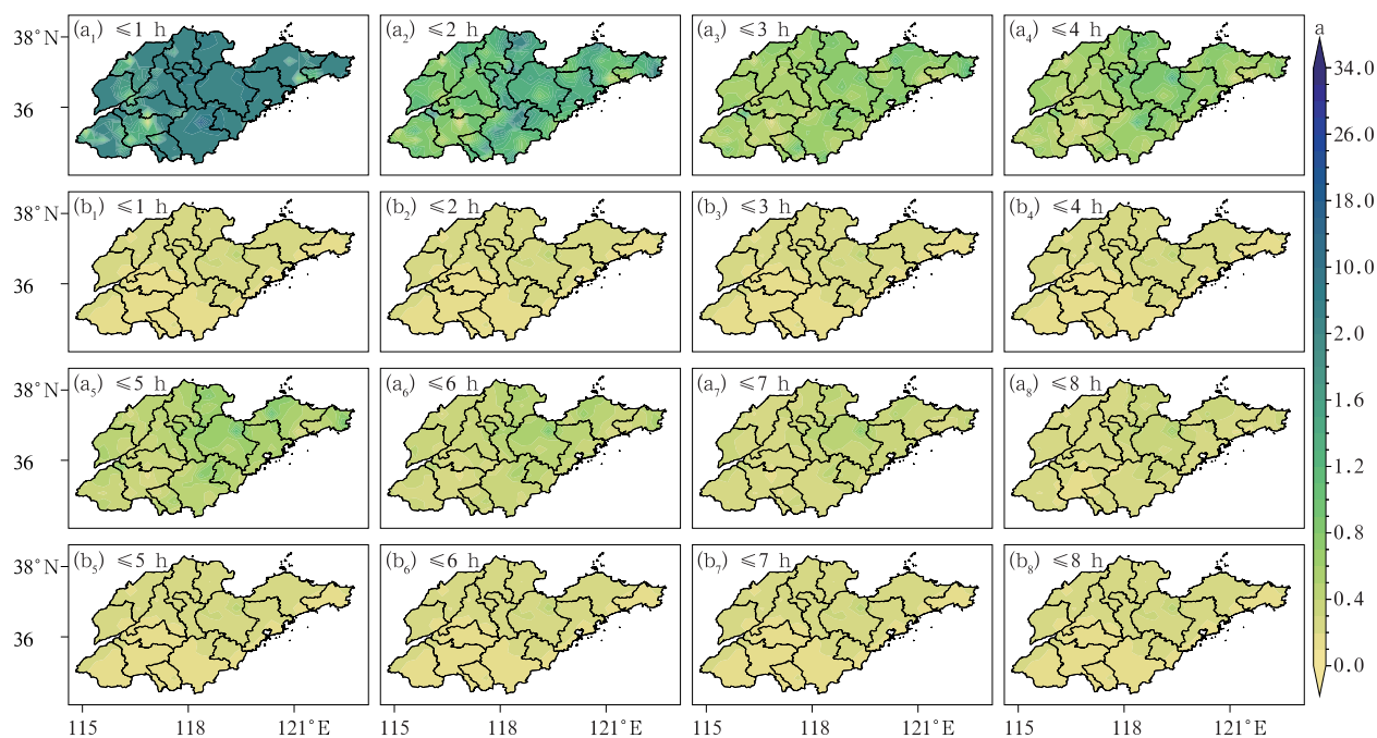
图 10 1966—2023 年山东强降水(降水量 \geq 50 mm)在不同降水持续时长阈值下的
