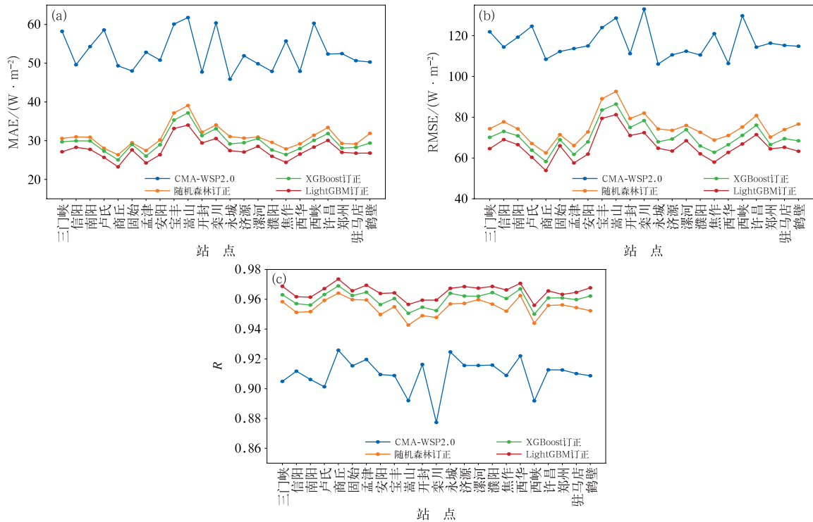
图 3 2022 年河南省各站点测试集中 CMA-WSP2.0 预报, 随机森林、XGBoost、LightGBM 订正的总辐照度 (a)MAE, (b)RMSE, (c)R
