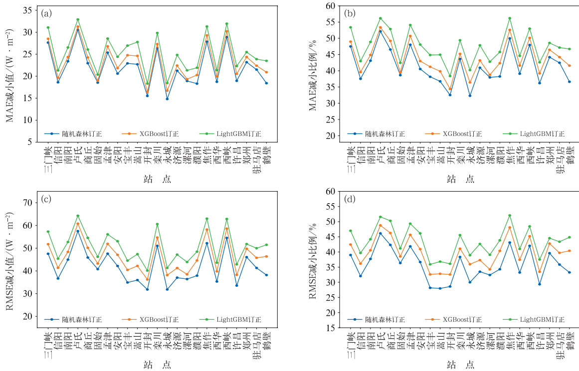
图 4 2022 年河南省各站点测试集中随机森林、XGBoost、LightGBM 订正的总辐照度
