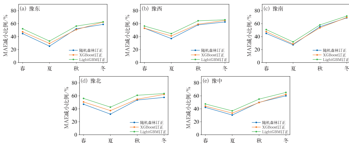
图 7 2022 年不同季节河南省 5 个区域测试集中随机森林、XGBoost、LightGBM 订正的总辐照度 MAE 减小比例
