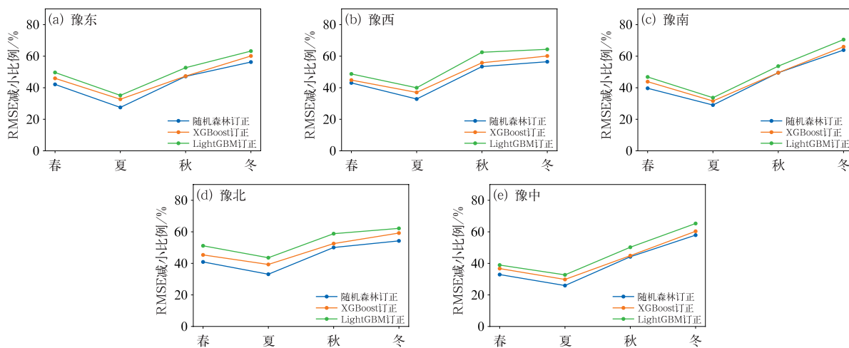
图 8 2022 年不同季节河南省 5 个区域测试集中随机森林、XGBoost、LightGBM 订正的总辐照度 RMSE 减小比例
