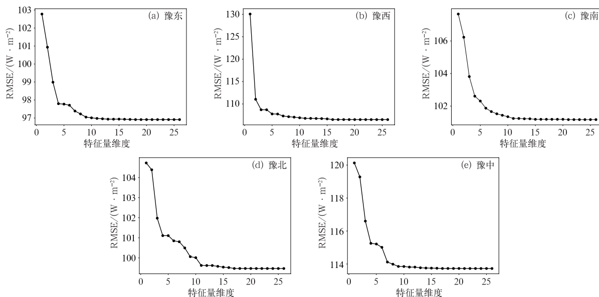
图 2 2022 年原始测试集中河南省 5 个区域基于 LASSO 回归预测总辐照度 RMSE 随特征量维度的变化
