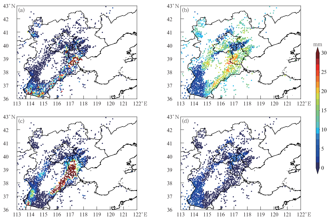
图 10 2019 年 8 月 9 日 20—23 时累计降水量分布
