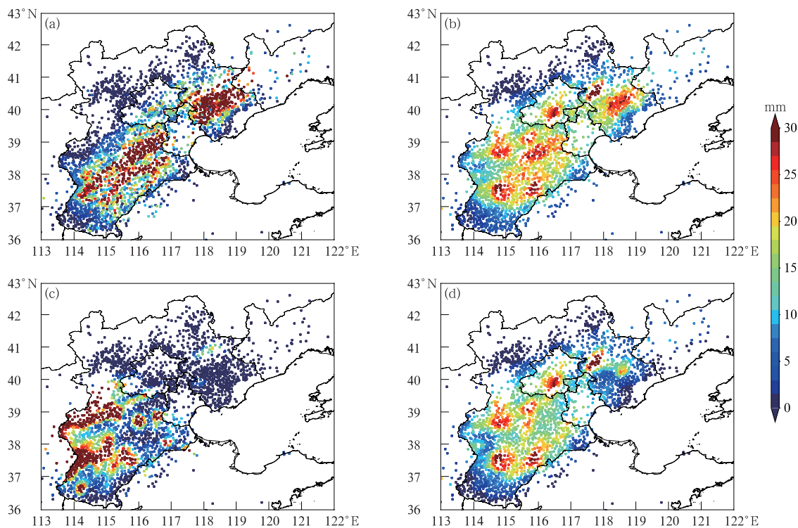
图 9 2019 年 7 月 29 日 14—17 时累计降水量分布
