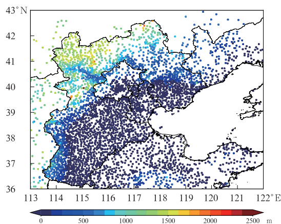
图 1 研究区域海拔高度(填色)及观测站点(圆点)分布
