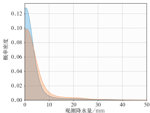
图 4 < 2 mm 降水 50% 下采样前(蓝色区域)和下采样后(橙色区域)降水样本的概率密度分布
