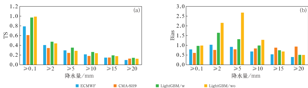
图 11 采用(LightGBM/w)和去除(LightGBM/wo)四类输入特征的 LightGBM、ECMWF、CMA-SH9 降水预报在测试集的(a)TS 和(b)Bias 评分
