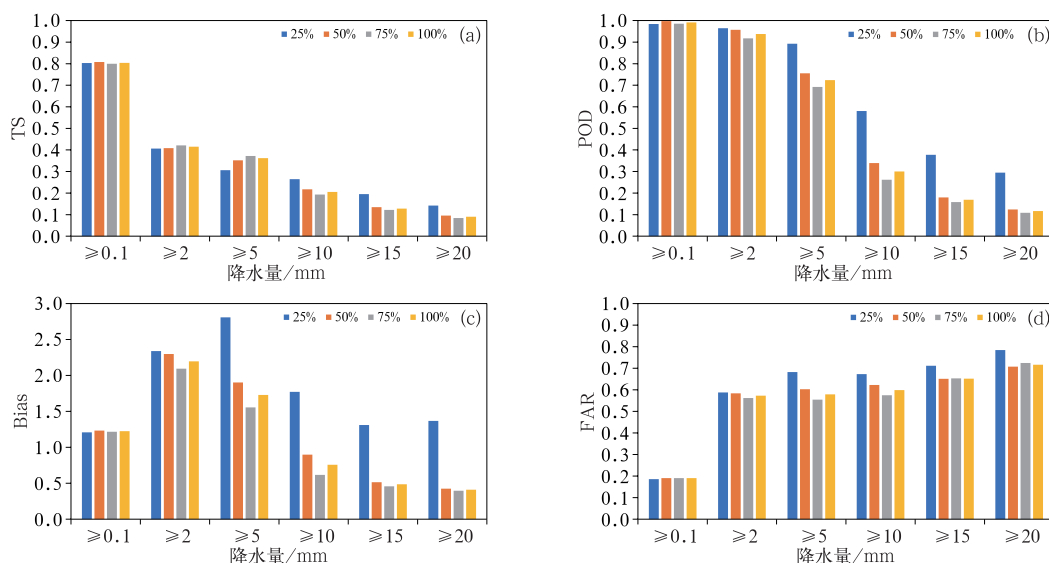
图3 <2 mm降水不同下采样比例测试集在不同降水量级的评分结果
