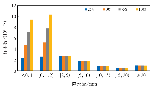
图2 <2 mm降水样本不同比例下采样后不同降水量区间的样本数分布
