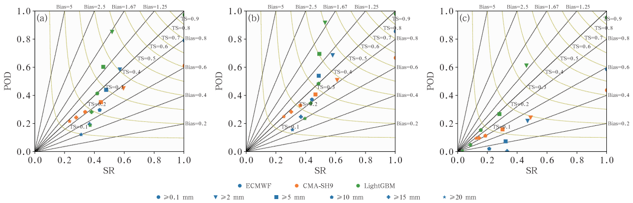
图 6 LightGBM、ECMWF 和 CMA-SH9 降水预报的综合评分
