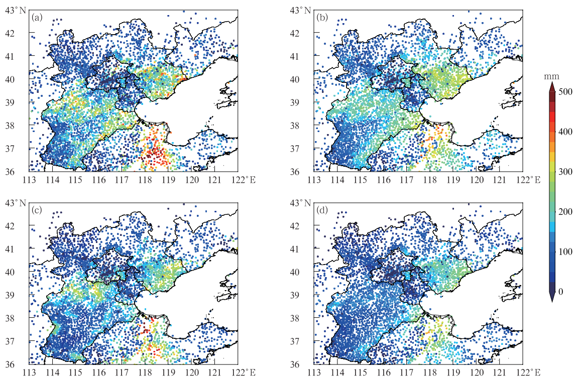
图 8 测试集(2019 年 7 月 21 日至 9 月 1 日)总降水量分布
