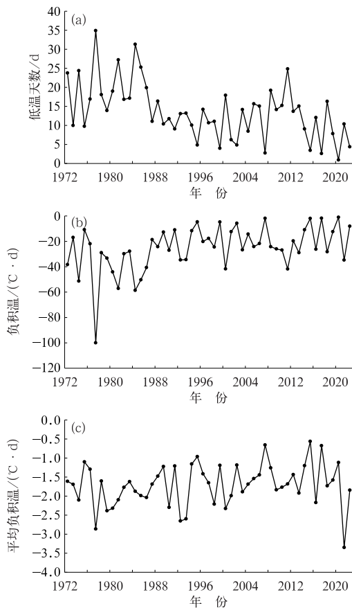
图 1 1972—2022 年江苏省(a)低温天数, (b)负积温, (c)平均负积温年际变化
