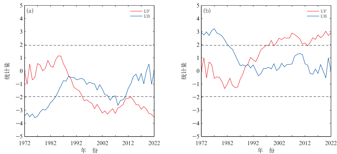
图 2 1972—2022 年江苏省(a)低温天数与(b)负积温的 Mann-Kendall 突变检验
