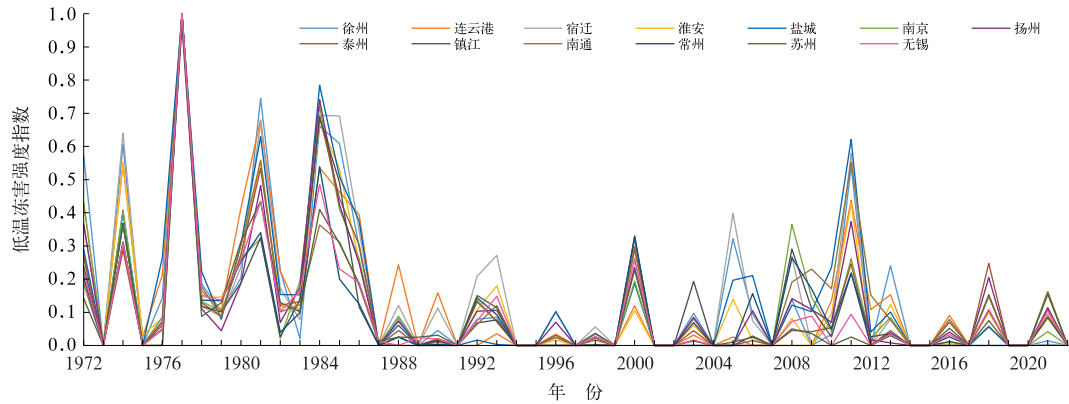
图 3 1972—2022 年江苏省各地冬小麦低温冻害强度指数年变化
