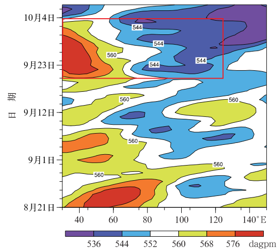
图 9 2017 年 8 月 21 日至 10 月 10 日 50^{\circ} \sim 70^{\circ}N 范围 500 hPa 平均位势高度(填色和等值线)的经度-时间演变
