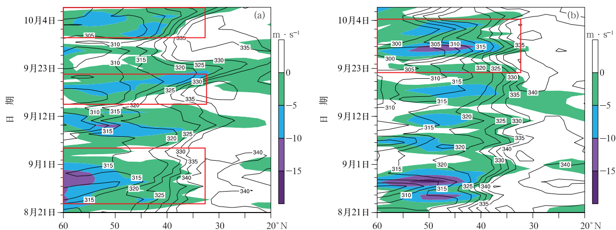
图 10 (a)2003 年和(b)2017 年 8 月 21 日至 10 月 10 日 100^{\circ}\sim 120^{\circ}\text{E} 范围 500 hPa 平均假相当位温(实线,单位:K)和平均经向北风(填色)的纬度-时间演变
