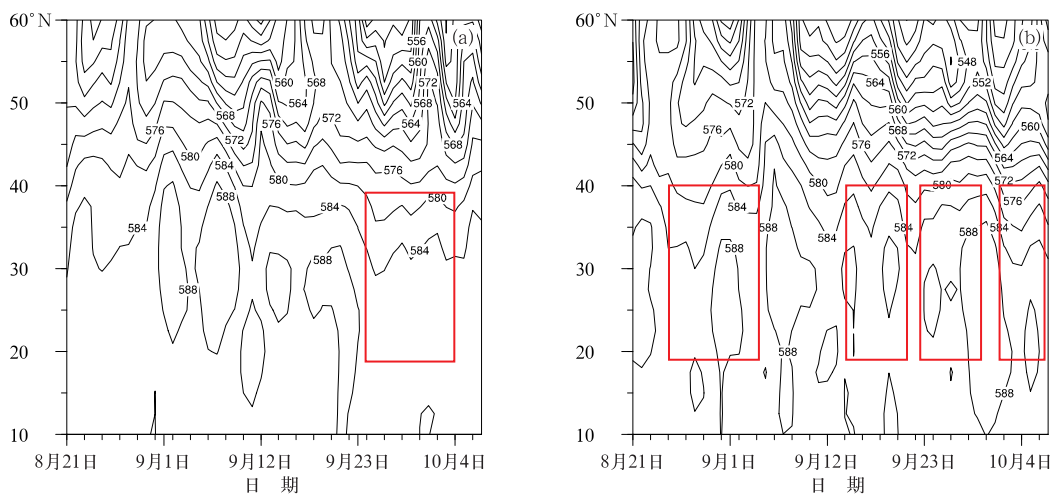
图 11 (a)2005 和(b)2021 年 8 月 21 日至 10 月 10 日 85^{\circ}\sim 95^{\circ}\text{E} 范围 500 hPa 平均位势高度(单位:dagpm)的纬度-时间演变
