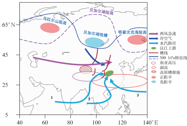
图 13 秋汛期汉江上游致洪降水 大尺度环流背景概念模型
