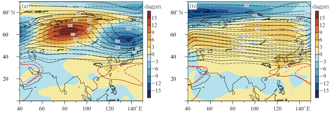
图 6 (a)中阻低压型 2003 年 8 月 21—31 日和(b)平直环流型 2005 年 9 月 1—30 日 500 hPa 位势高度距平(填色)
