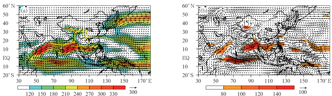
图 12 2023 年 8 月 21 日至 10 月 10 日整层积分的(a)水汽输送通量(箭矢和填色,单位: \text{kg}\cdot\text{m}^{-1}\cdot\text{s}^{-1} )和(b)距平(箭矢和填色,单位: \text{kg}\cdot\text{m}^{-1}\cdot\text{s}^{-1} )
