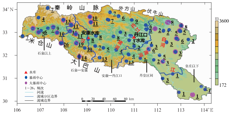
图 3 2000—2023 年秋汛期洪水过程的暴雨、大暴雨中心位置及频次分布
