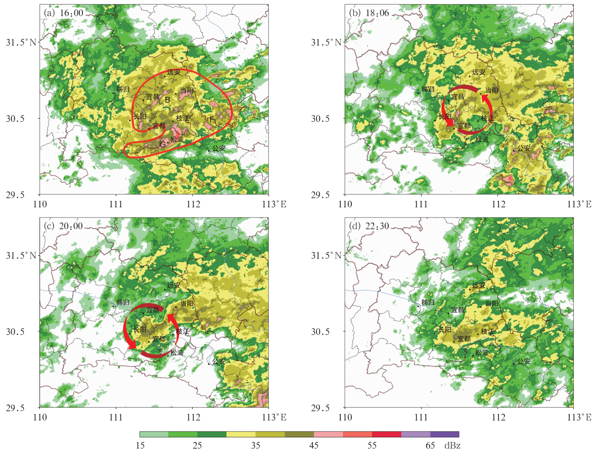
图4 2018年4月22日强降水 MCS 涡旋阶段雷达组合反射率因子
