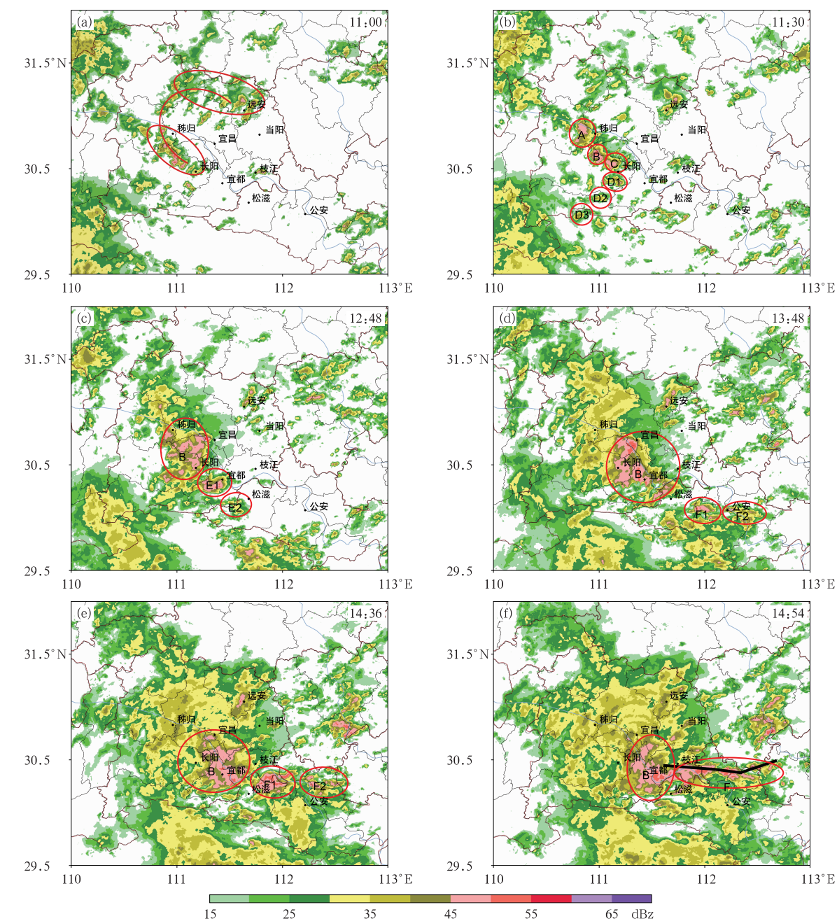
注:红圈表示各回波和 MCS,字母标记其编号;图 a 中红色弧线示意回波的“C”字型形态;图 f 中黑色折线为图 3 剖面。
