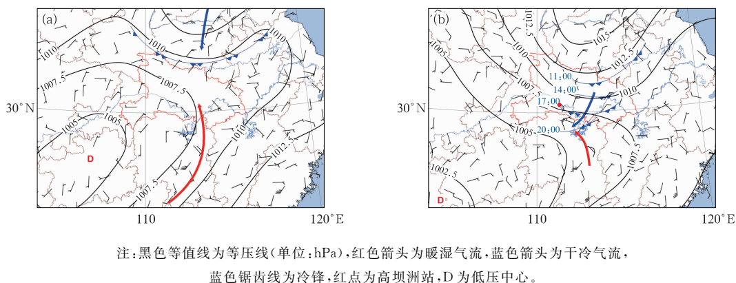
图 7 2018 年 4 月 22 日(a)08:00,(b)20:00 地面环流形势
