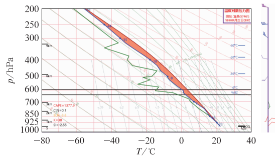
图 6 2018 年 4 月 22 日 08:00 宜昌探空图
