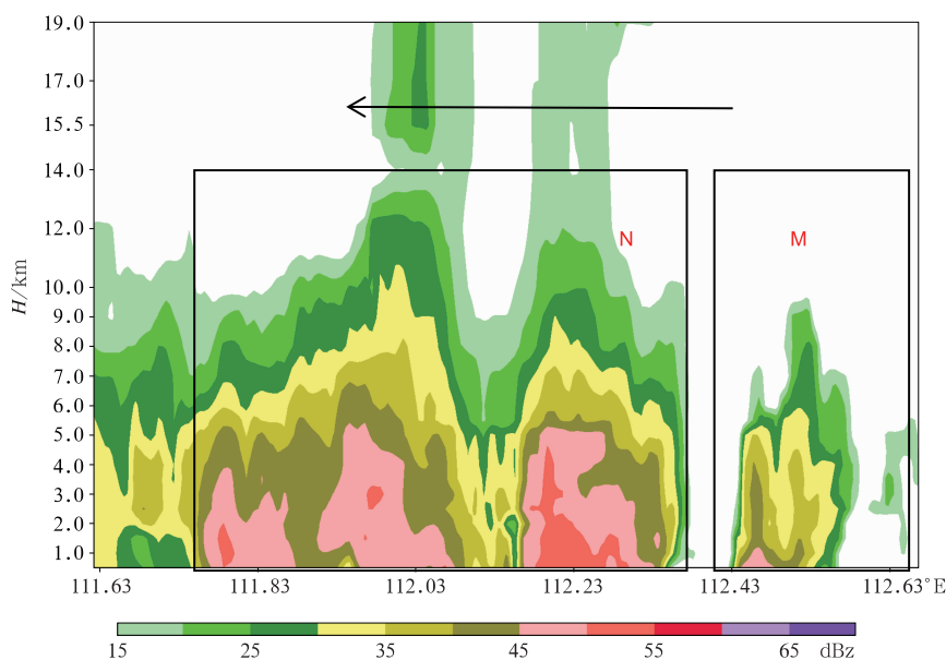
图 3 2018 年 4 月 22 日 14:54 雷达反射率因子沿
