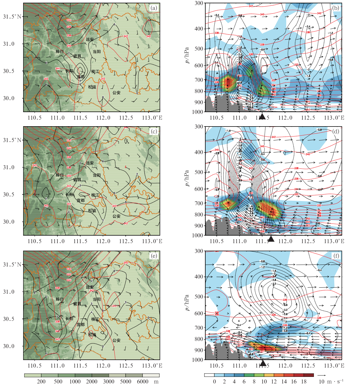
图 8 2018 年 4 月 22 日(a,c,e)850 hPa 锋生函数(黑色等值线,单位: 10^{-9} \text{ K} \cdot \text{m}^{-1} \cdot \text{s}^{-1} )、假相当位温(红色等值线,单位:K)、水平风场(风羽)及地形(填色),(b,d,f)锋生函数(填色,单位: 10^{-9} \text{ K} \cdot \text{m}^{-1} \cdot \text{s}^{-1} )、假相当位温(红色等值线,单位:K)、垂直速度(黑色等值线,单位: \text{Pa} \cdot \text{s}^{-1} )、纬向-垂直速度风矢量(箭头)及地形(灰色阴影)沿 30.5^\circ\text{N} 的垂直剖面 (a)13:00,(b,c)14:00,(d,e)16:00,(f)22:00
