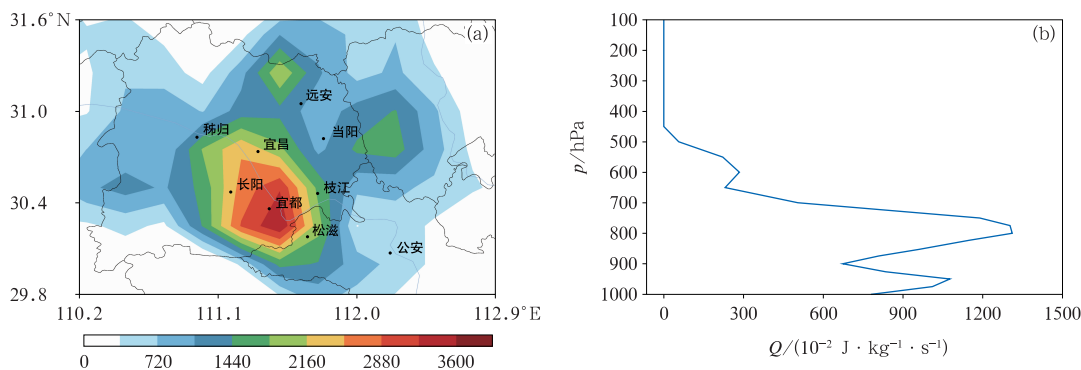
图 10 2018 年 4 月 22 日 16:00(a)800 hPa 凝结潜热加热(单位: 10^{-2} \text{ J} \cdot \text{kg}^{-1} \cdot \text{s}^{-1} ), (b)强降水区域 ( 30^{\circ} \sim 31^{\circ} \text{N} , 110.75^{\circ} \sim 112.25^{\circ} \text{E} ) 平均凝结潜热加热垂直分布
