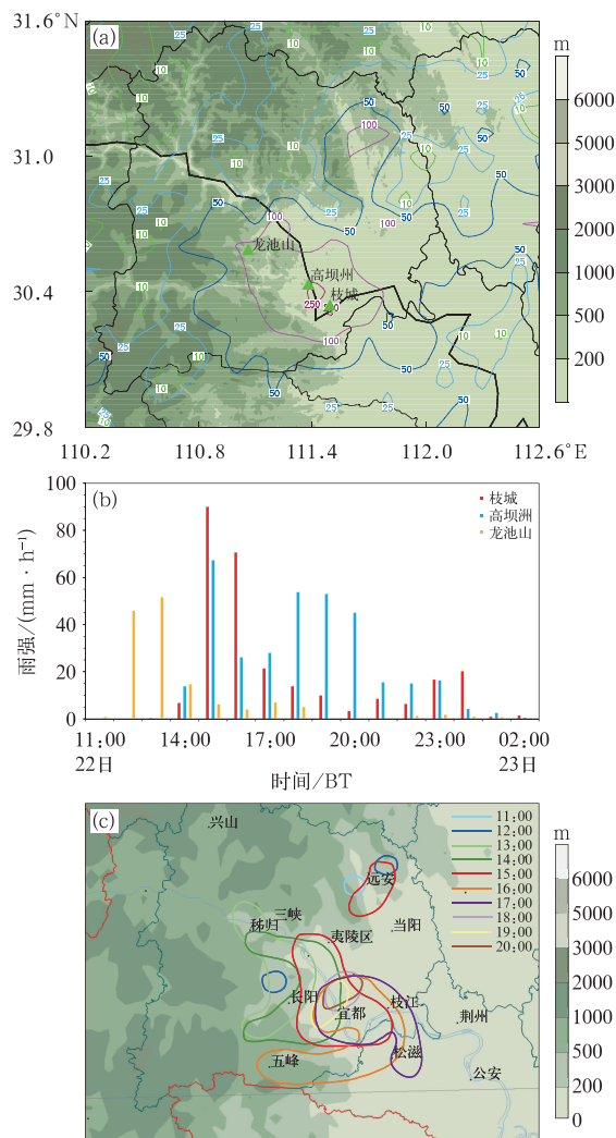
图 1 2018 年 4 月 22 日 08:00 至 23 日 08:00 宜昌地区(a)24 h 累计雨量(等值线,单位:mm)叠加地形(填色),(b)代表站小时雨强,(c)小时雨强超过 30 \text{ mm} \cdot \text{h}^{-1} 的雨团移动路径叠加地形(填色)
