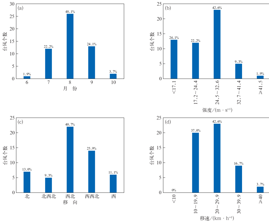
图 2 1950—2022 年登陆华东北部的台风统计特征
