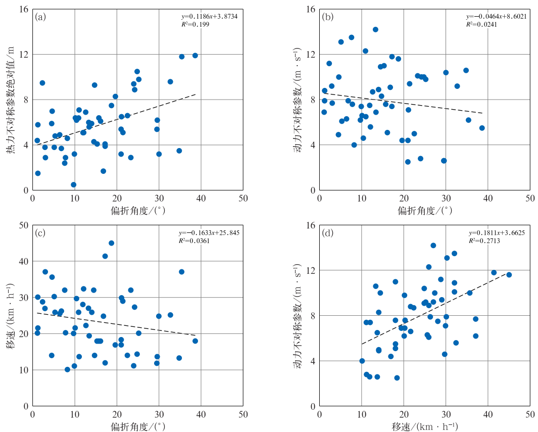
图 6 1950—2022 年登陆华东北部台风临近登陆时刻(a)热力不对称参数绝对值与偏折角度,(b)动力不对称参数与偏折角度,(c)移速与偏折角度,(d)动力不对称参数与移速的散点图
