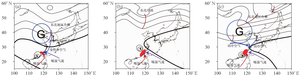
注:黑色等值线为 500 hPa 高度场(其中加粗为 5880 gpm 线),红色短线为 500 hPa 槽线,红色阴影为 6 h 降水量 \geq 100\text{ mm} 强降水落区,红色或紫色箭头分别为低层来自南海和西太平洋的暖湿气流,蓝色箭头为低层变性或弱冷空气。
