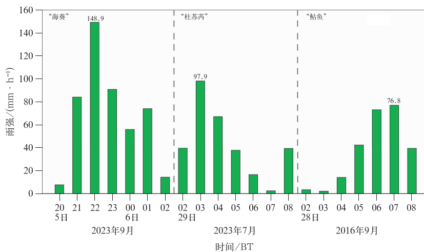
图 2 三个登闽台风极端降水期间的小时雨强演变
