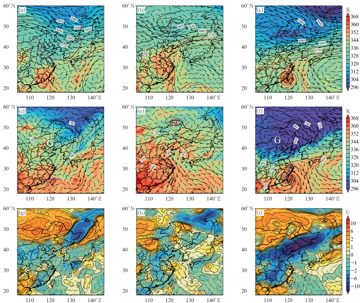
注:图 a~c 中,红棕色短线代表 500 hPa 槽线,红色加粗等值线为 5880 gpm 线;图 d~f 中,紫色短线代表 925 hPa 切变线, G 和 D 分别代表位势高度高、低值中心;台风符号代表对应时刻台风中心位置,下同。
