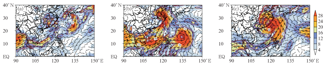
图 4 小时雨强最大时刻 925 hPa 水汽通量(填色,单位: 10^{-2} \text{ kg} \cdot \text{m}^{-1} \cdot \text{s}^{-1} )、风场(风羽)及风速(等值线, \geq 8 \text{ m} \cdot \text{s}^{-1} )分布 (a)“海葵”:2023 年 9 月 5 日 22:00,(b)“杜苏芮”:2023 年 7 月 29 日 03:00,(c)“鲇鱼”:2016 年 9 月 28 日 07:00
