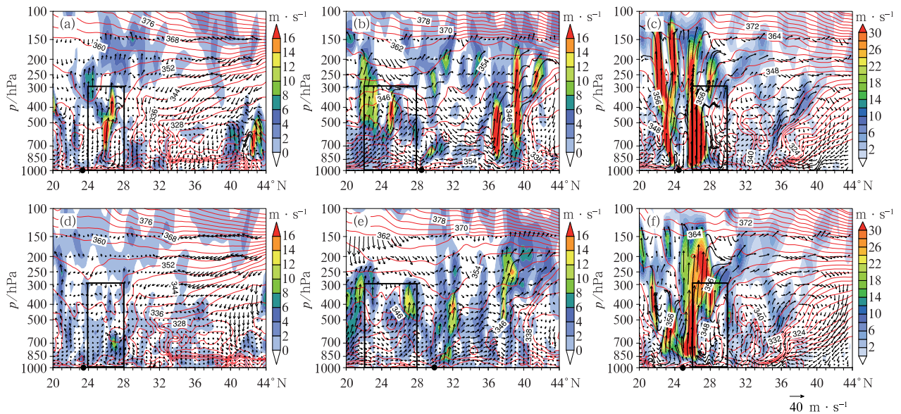
图 9 v (风矢)、假相当位温(等值线,单位:K)及垂直速度(填色)的经向垂直剖面
