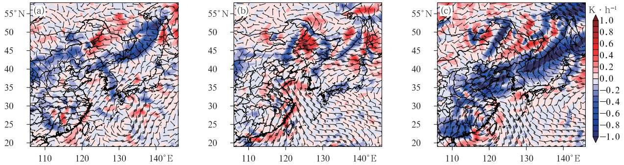
图 5 小时雨强最大时刻 925 hPa 水平温度平流(填色)和风场(风羽)分布
