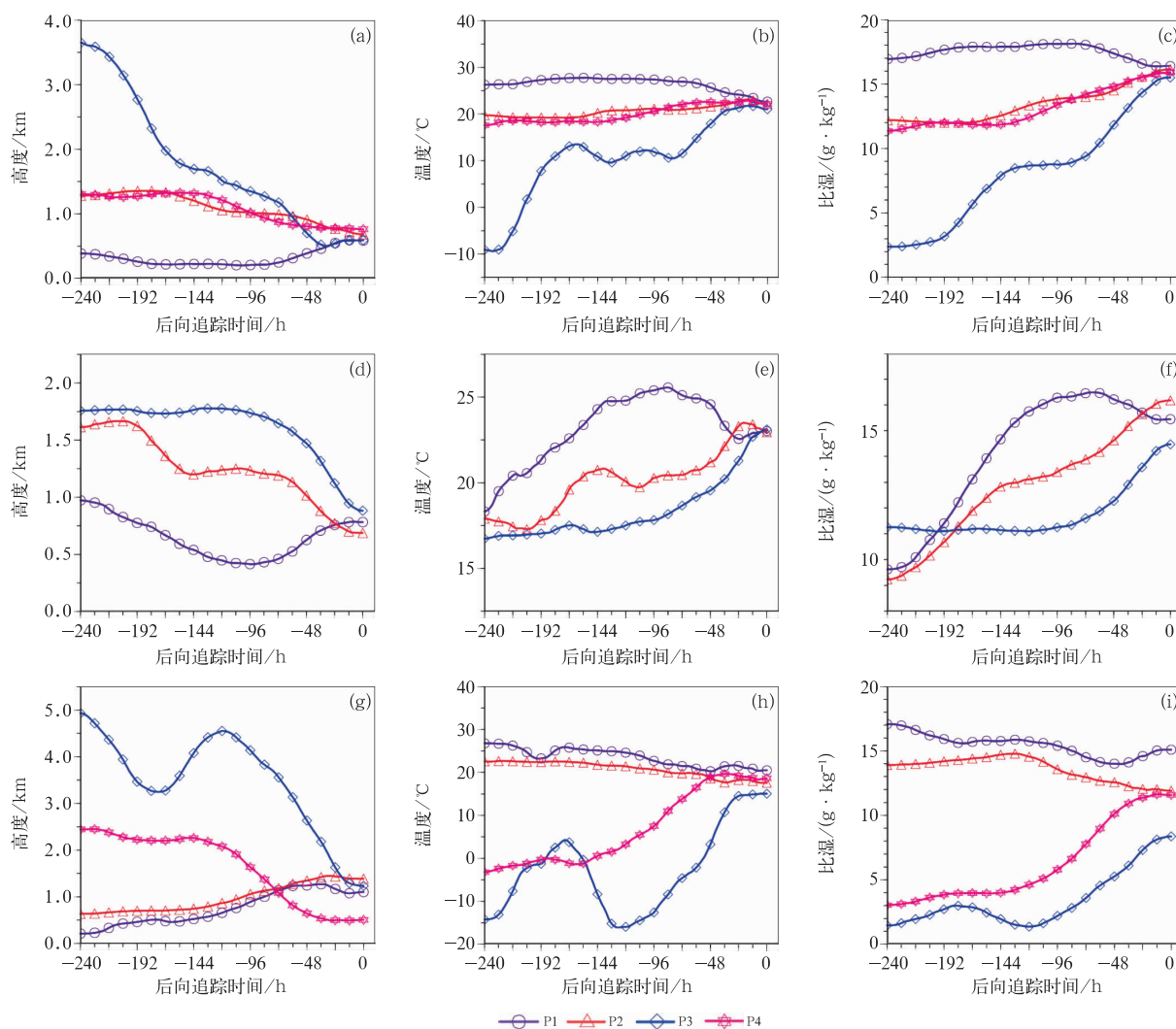
注:标记点间隔 12 h;P1~P4 为图 6 中 800 m 高度对应通道。
