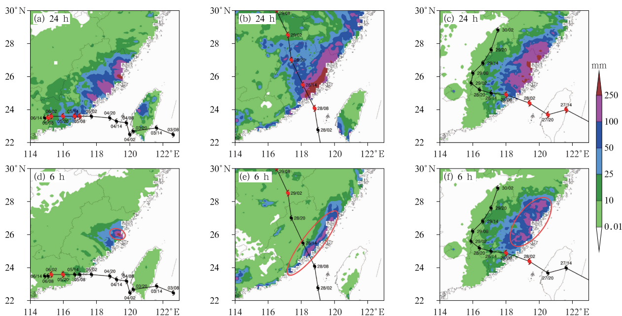
图 1 三个登闽台风最强 24 h、6 h 累计降水量(填色)与台风路径(黑色折线)
