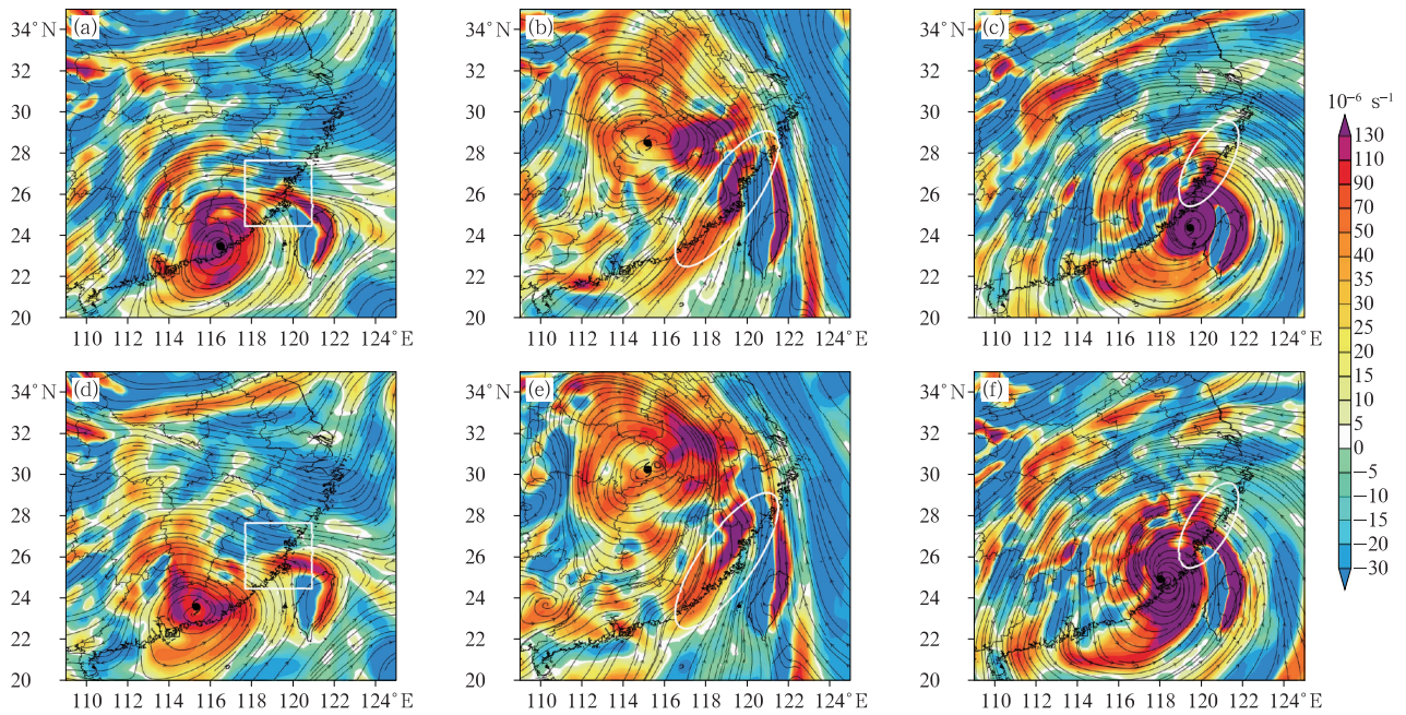
图 8 850 hPa 流场(流线)和相对涡度(填色)分布
