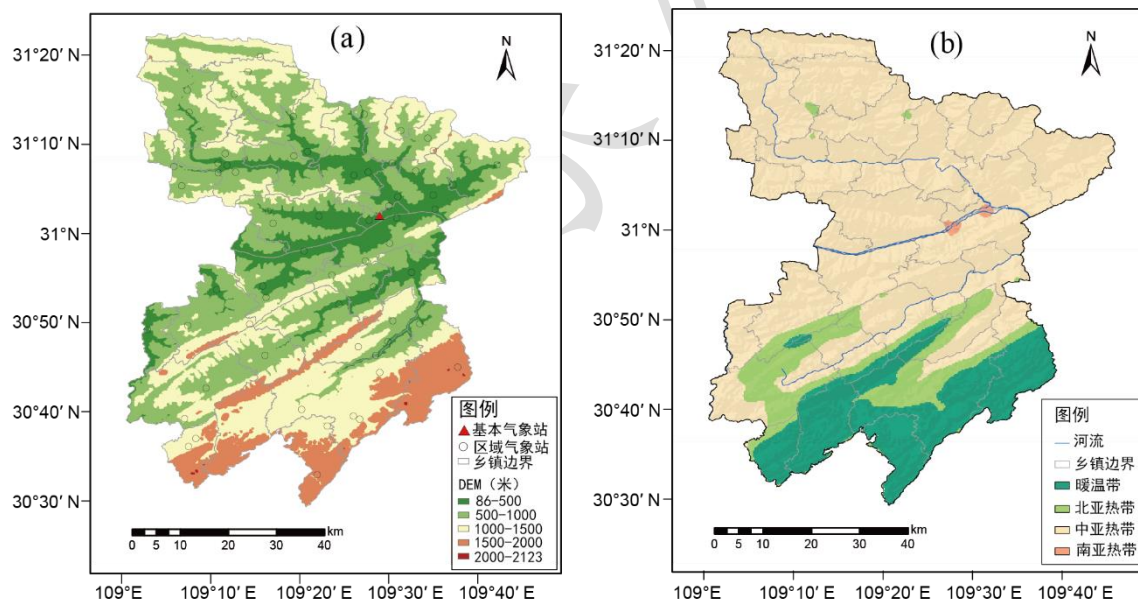
图 1 奉节县(a)高程及(b)气候带分布
