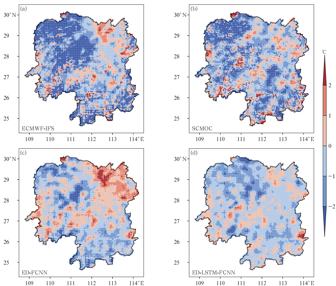
图 7 2022 年 8 月 19 日 14 时湖南不同预报产品气温预报值与观测值的偏差空间分布
