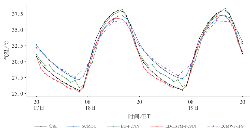
图 6 2022 年 8 月 17 日 20 时至 19 日 20 时湖南不同预报产品 平均气温预报与实况对比
