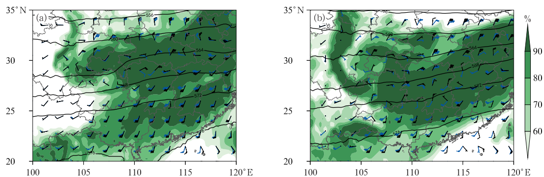
图9 2022年11月(a)28日14时,(b)29日02时500 hPa高度场(等值线,单位:dagpm)、850 hPa风场(蓝色风羽)、850 hPa相对湿度(填色)和925 hPa风场(黑色风羽)
