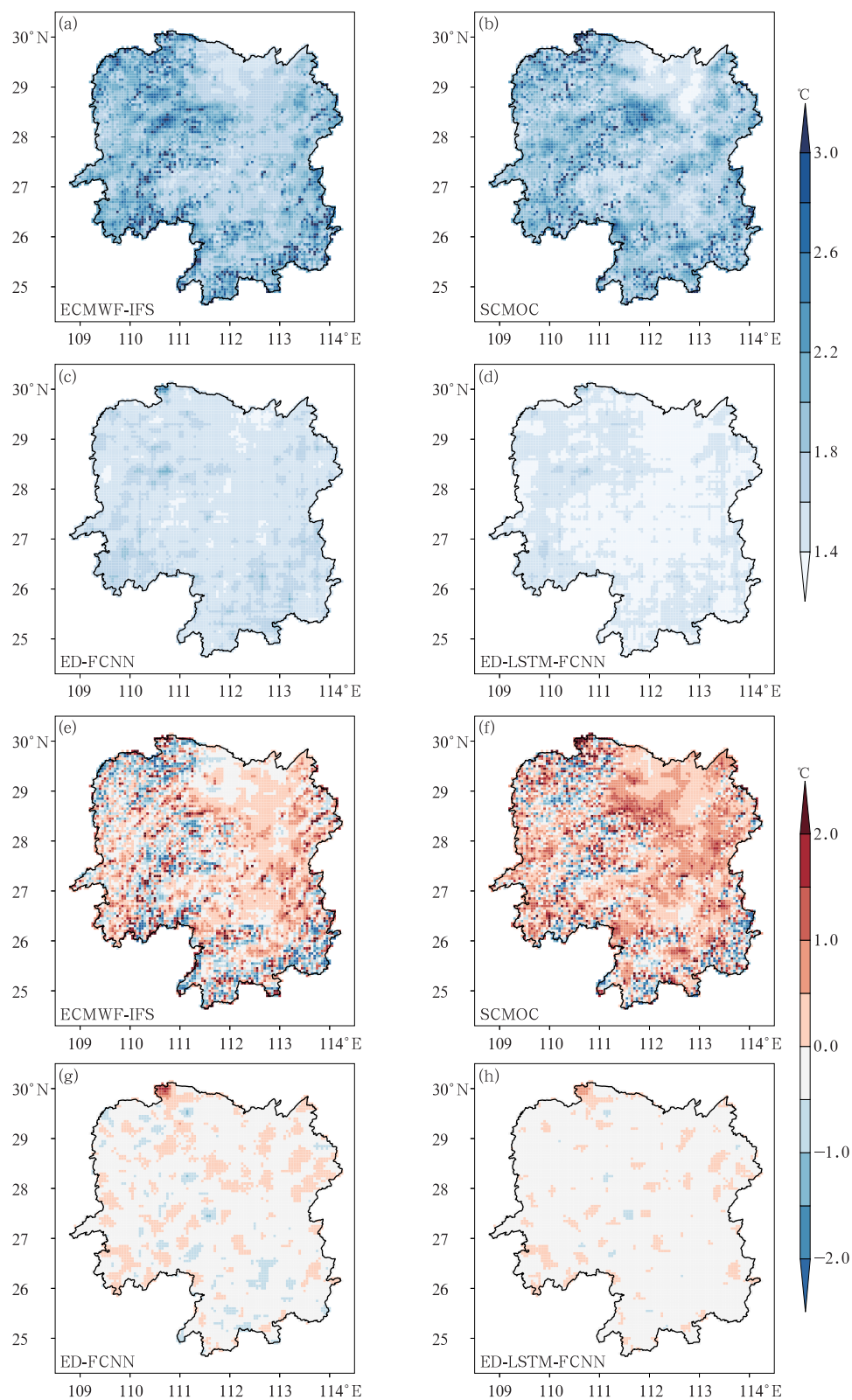
图 4 2022 年湖南不同预报产品气温预报的平均
