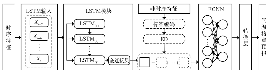
图2 ED-LSTM-FCNN 模型结构
