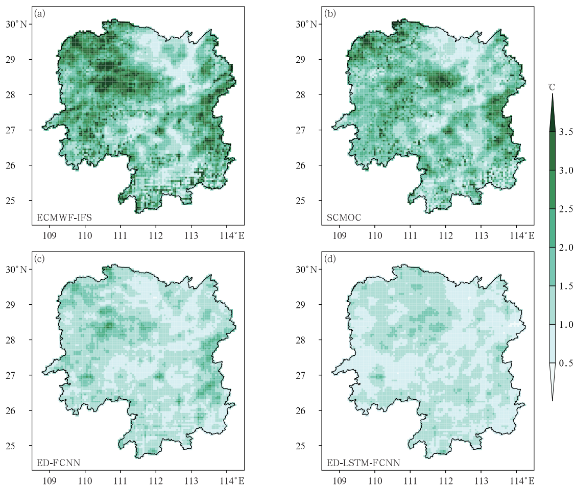
图8 2022年8月17—19日湖南不同预报产品气温预报的RMSE空间分布
