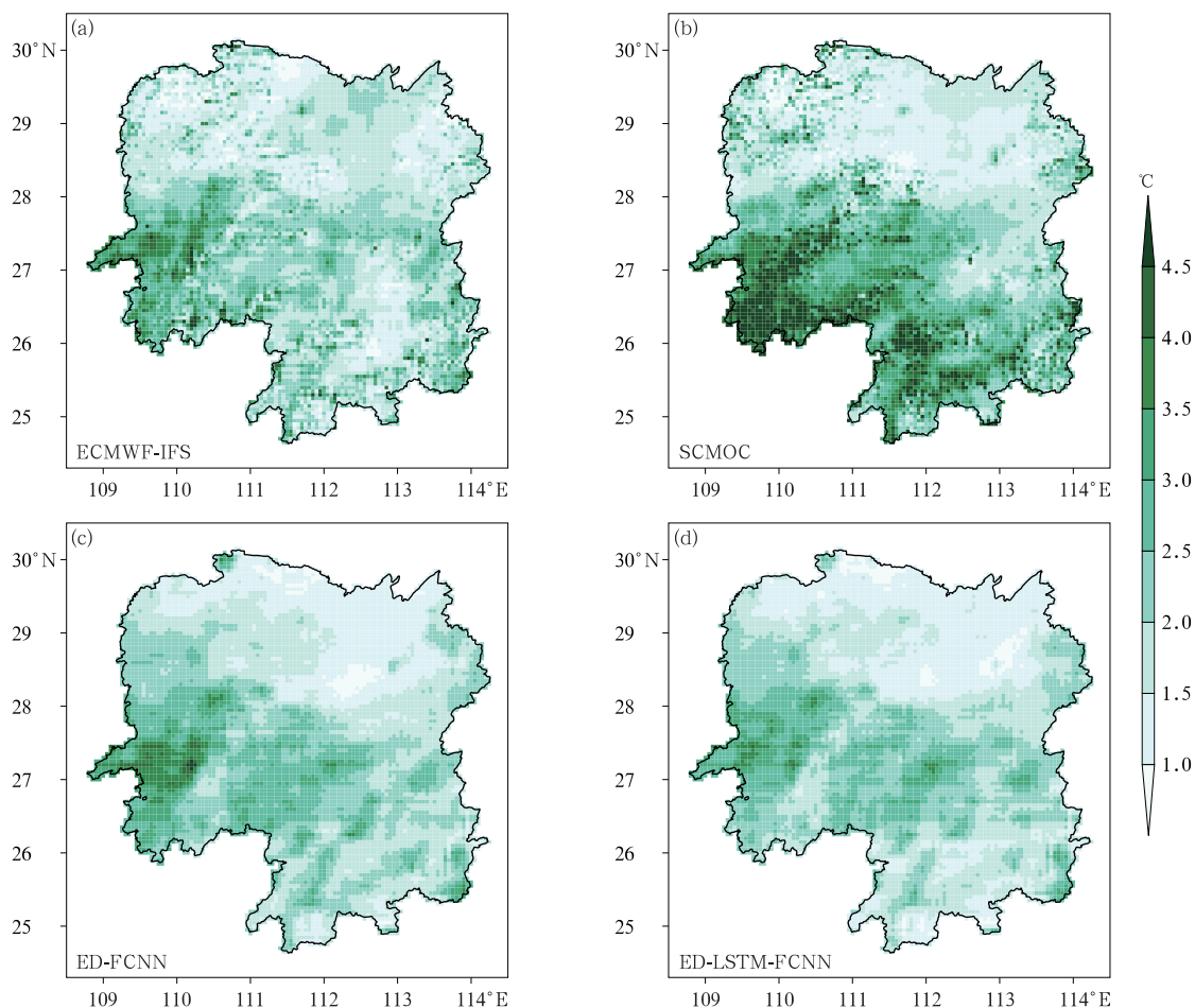
图 12 2022 年 11 月 27—29 日湖南不同预报产品气温预报的 RMSE 空间分布
