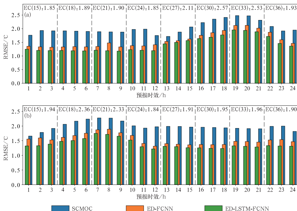
图 3 2022 年湖南不同预报产品(a)20 时、(b)08 时起报的各预报时效气温预报均方根误差
