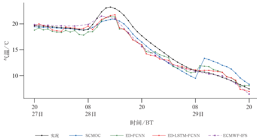
图 10 2022 年 11 月 27 日 20 时至 29 日 20 时湖南不同预报产品平均气温预报与实况对比 Fig. 10 Comparison between the average temperature forecast of different forecast products and observations in Hunan Province from 20:00 BT 27 to 20:00 BT 29 November 2022
