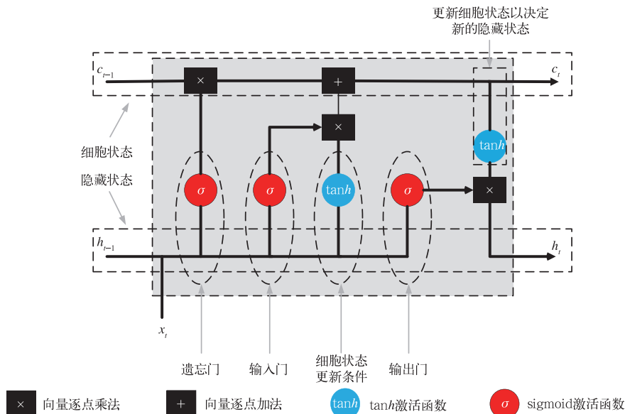
图 1 长短期记忆神经网络结构
