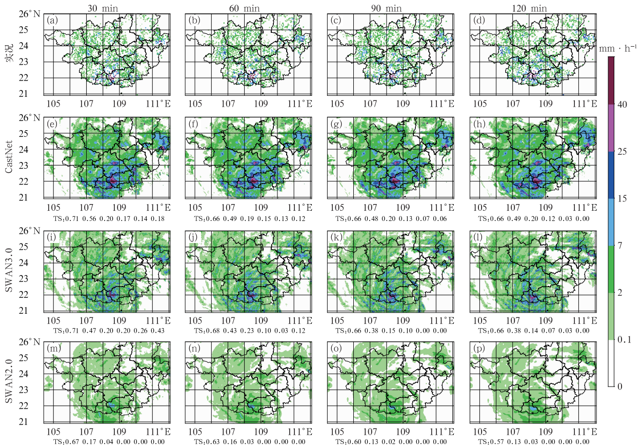
图 6 CastNet、SWAN 3.0、SWAN 2.0 不同预报时效的降水强度预报结果与实况:
