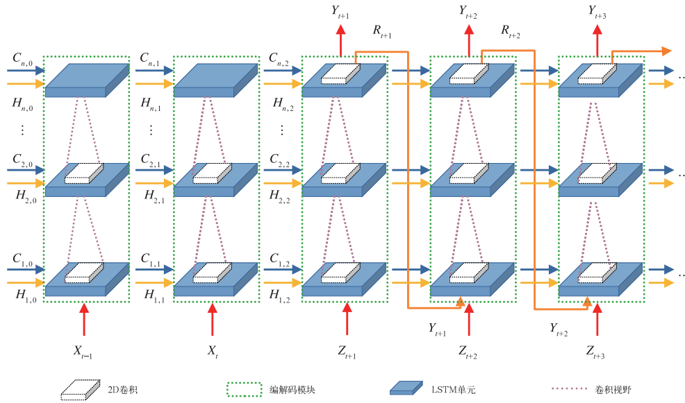
注: H : 隐藏层, C : 记忆单元, R : 残差连接路径, t : 时间序列; X_t, Z_{t+1}, Y_{t+1} 分别表示 t 或 t+1 时刻雷达数据输入、隐变量输入、模型输出。
