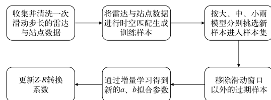
图3 滑动窗口 Z-R 参数动态更新流程图
