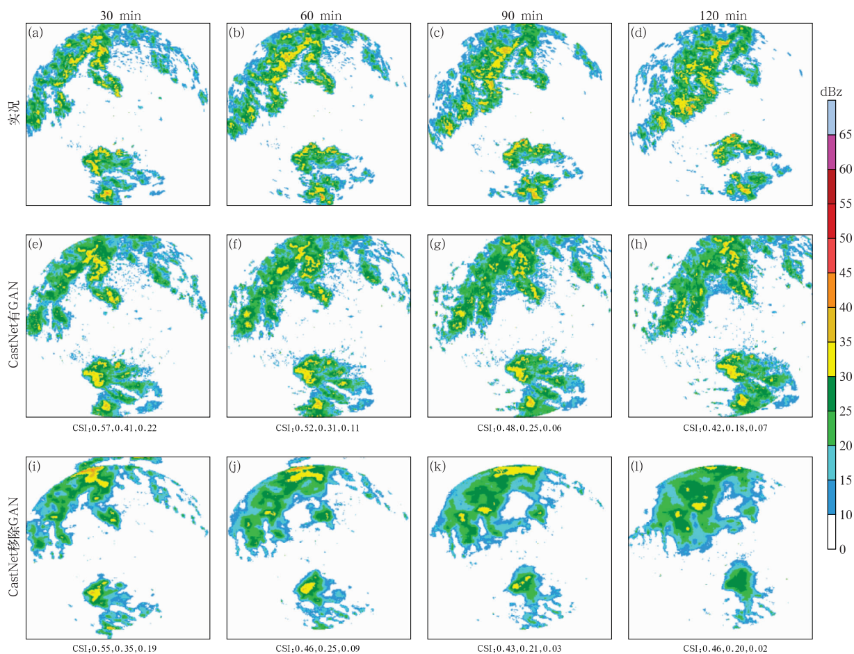
图 11 CastNet 移除 GAN 模块前后在 2023 年 5 月 24 日 08:00 起报的不同时效回波强度预报与实况对比
