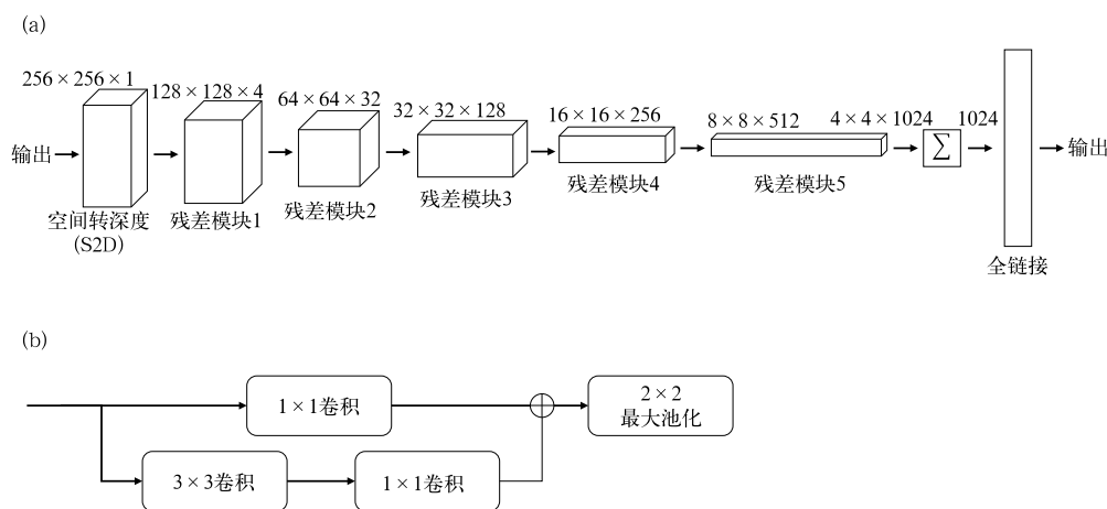
图 2 CastNet 架构示意图:GAN 判别网络部分
