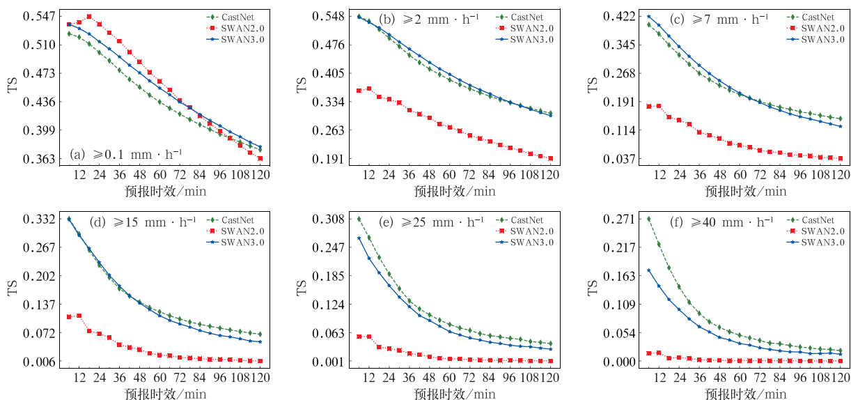
图 9 CastNet, SWAN 3.0, SWAN 2.0 对 2023 年 5—10 月广西主要降水过程在不同降水强度下的不同预报时效 TS 评分
