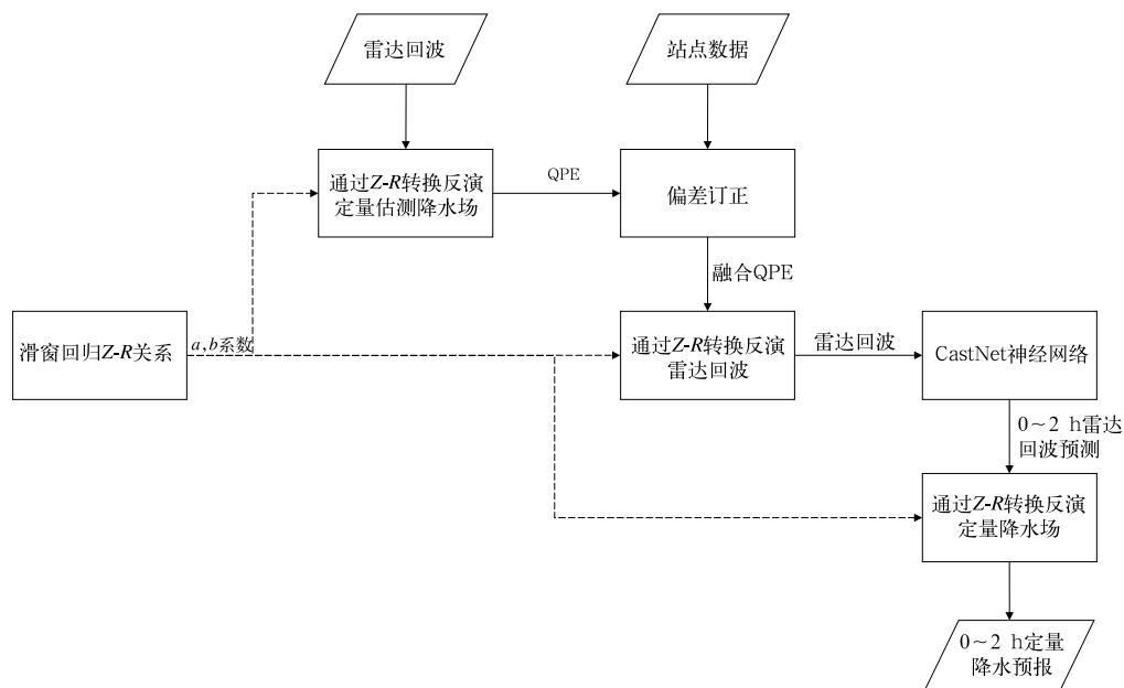
图 4 定量降水外推预报流程图
