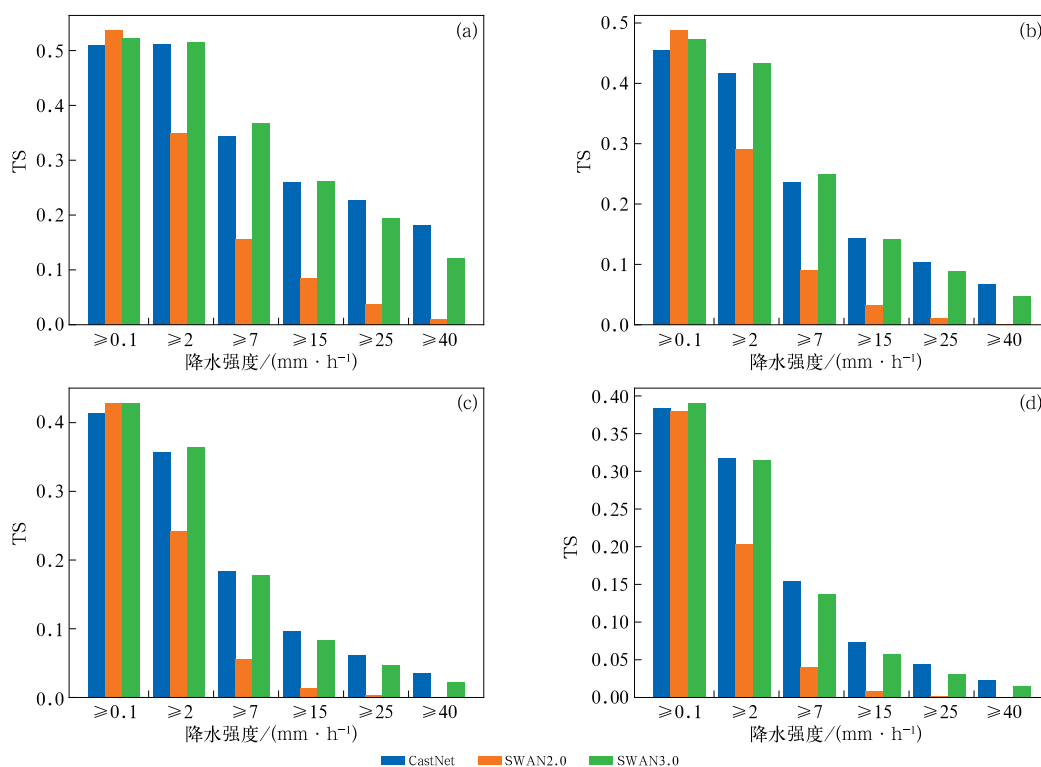
图8 CastNet,SWAN 3.0,SWAN 2.0对2023年5—10月广西主要降水过程在不同预报时效下的不同降水强度预报TS评分
