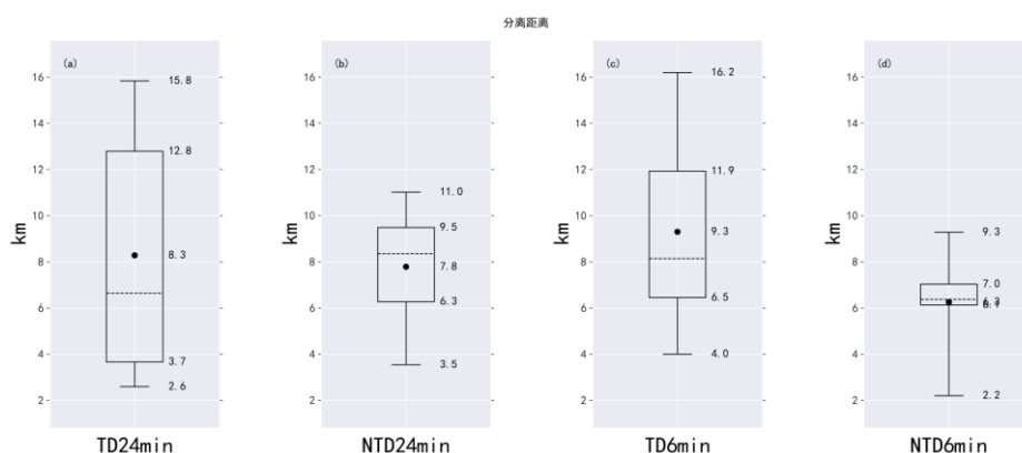
图 6 1km 等高平面上 K_{DP} 足质心和 Z_{DR} 弧质心的分离距离箱线图
