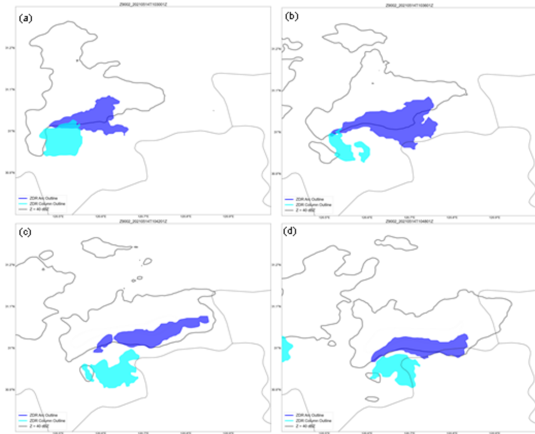
图 2 2021 年 5 月 14 日苏州强龙卷超级单体 1km 等高平面上 Z_{DR} 弧(深蓝色区域)和 Z_{DR} 柱(浅蓝色区域)演变
