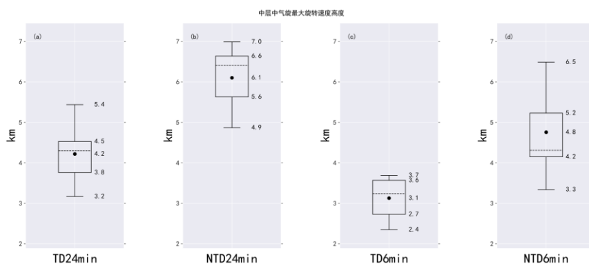
图 9 中层中气旋最大旋转速度高度箱线图
