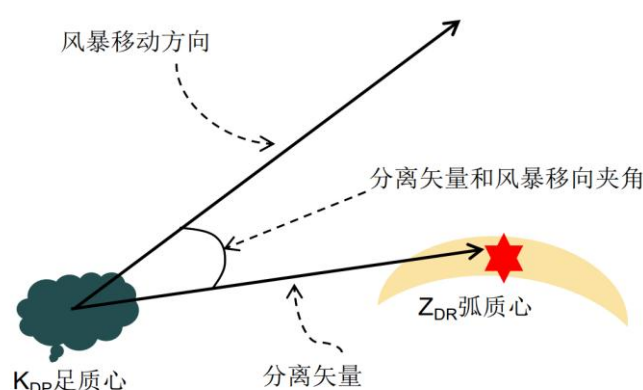
图 1 低层 K_{DP} 足和 Z_{DR} 弧的质心分离矢量与风暴运动方向夹角示意图(Loeffler and Kumjian, 2018)
