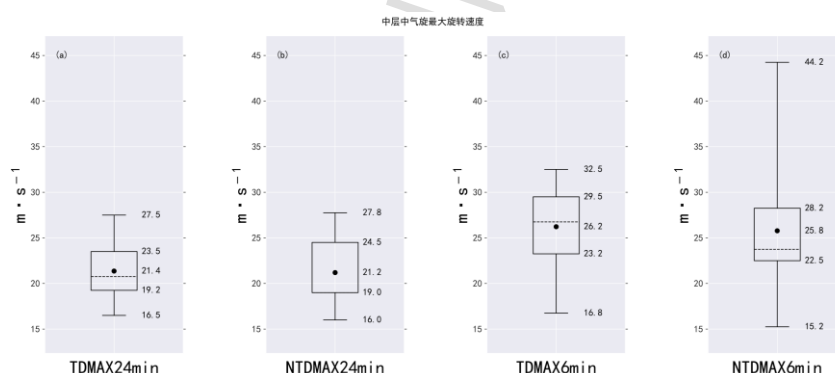
图 10 中层中气旋最大旋转速度箱线图
