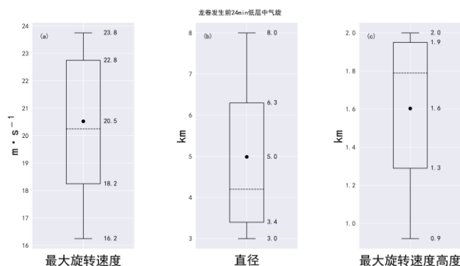
图 7 龙卷发生前 24min 低层中气旋箱线图
