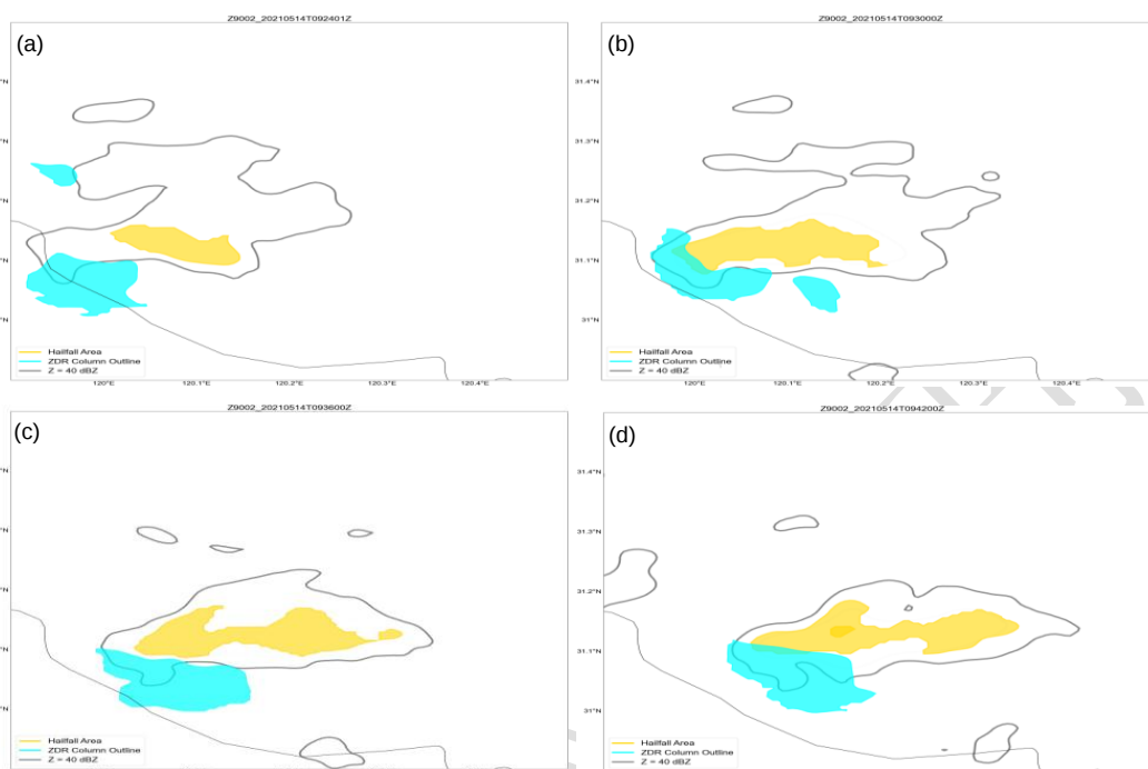
图 4 2021 年 5 月 14 日非龙卷超级单体 3.5km 等高平面上 Z_{DR} 柱（蓝色区域）和冰雹区域（黄色区域）演变 Fig.4 The evolution of the Z_{DR} column (blue area) and hail area (yellow area) for the non-tornadic supercell at 3.5 km AGL on 14 May 2021
