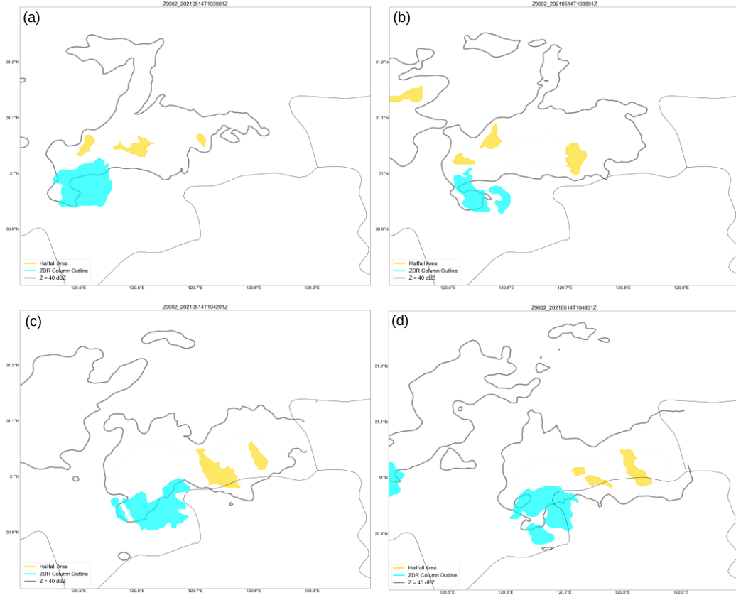
图 5 2021 年 5 月 14 日龙卷超级单体 3.5km 等高平面上 Z_{DR} 柱（蓝色区域）和冰雹区域（黄色区域）演变 Fig.5 The evolution of the Z_{DR} column (blue area) and hail area (yellow area) for the tornadic supercell at 3.5 km AGL on 14 May 2021
