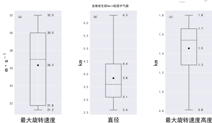
图 8 龙卷发生前 6min 低层中气旋箱线图
