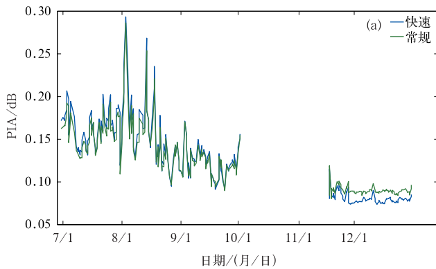
图 6 2022 年快速方法和常规方法计算的(a)Ku 波段,(b)Ka 波段总衰减对比
