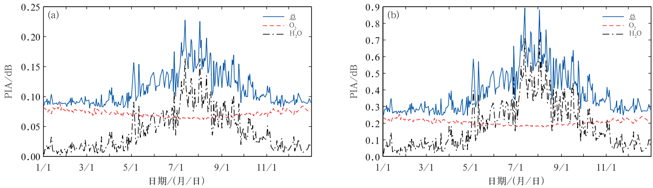
图 1 2023 年(a)Ku 波段和(b)Ka 波段的大气衰减变化
