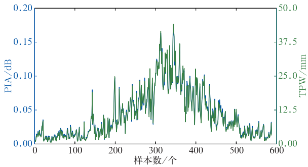
图 3 2023 年 Ku 波段水汽衰减(蓝线)和水汽总量(绿线)之间的关系
