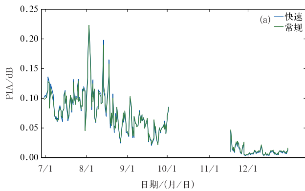
图 5 2022 年快速方法和常规方法计算的(a)Ku 波段,(b)Ka 波段水汽衰减对比
