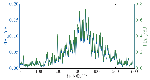
图 4 2023 年 Ku 波段水汽衰减(蓝线)和 Ka 波段水汽衰减(绿线)之间的关系
