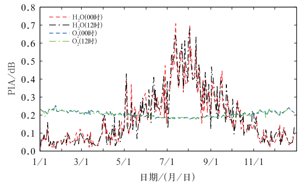
图 2 Ka 波段 2023 年 12 时和 00 时的大气衰减对比
