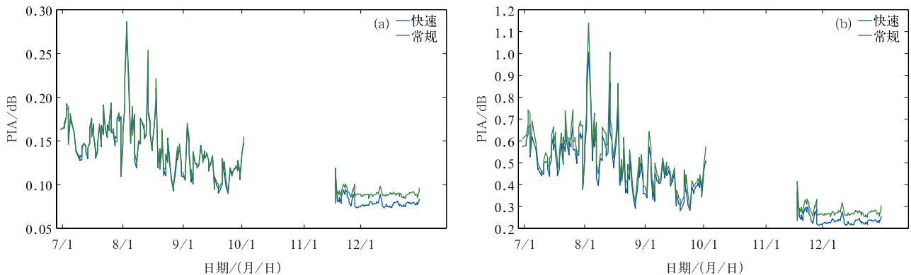
图 7 2022 年基于 IGRA 水汽总量利用快速方法和常规方法计算的 (a)Ku 波段,(b)Ka 波段总衰减对比
