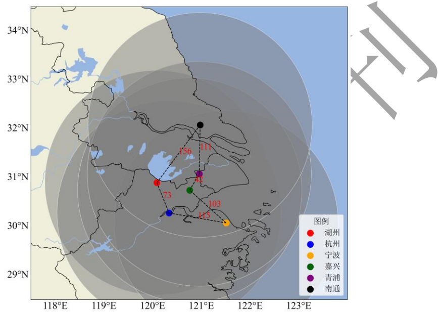
图 1 参与评估的 6 部 S 波段双偏振雷达位置（彩色圆点）与扫描范围（灰色阴影）
