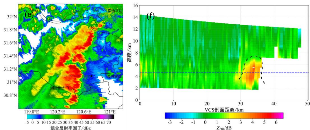
图4 2024年7月10日(a,b) 19:33青浦雷达(VCP11D)、(c,d) 19:33湖州雷达(VCP216D)、(e,f) 19:34南通雷达(VCP21D) (a,c,e) 组合反射率因子及(b,d,f) 对应差分反射率剖面
