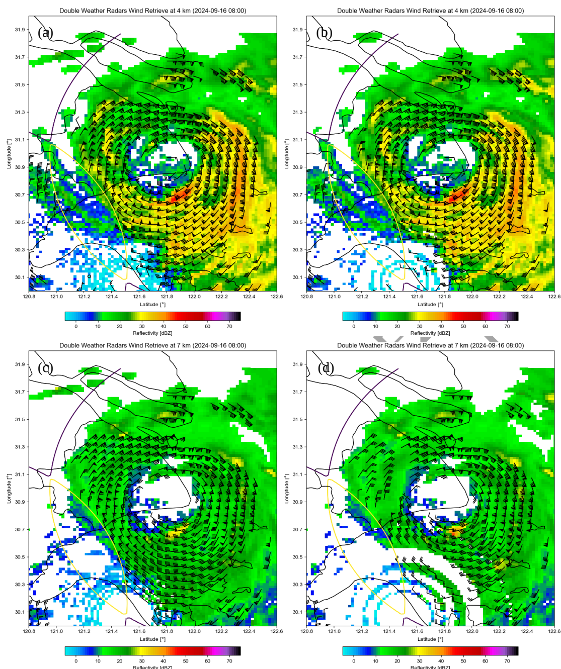
图9 2024 年台风“贝碧嘉”期间 9 月 16 日 08:00 基于青浦和宁波双雷达 (a, c) 对流模式 (VCP216D、VCP11D) 和 (b, d) 降水模式 (VCP21D) 在 (a, b) 4 km 和 (c, d) 7 km 高度的反射率因子 (填色) 和反演风场 (风羽)
