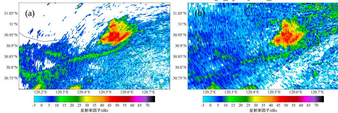
图6 2024年7月18日(a)14:06嘉兴雷达(VCP216D)1.0°、(b)14:09青浦雷达(VCP11D)0.5°反射率因子
