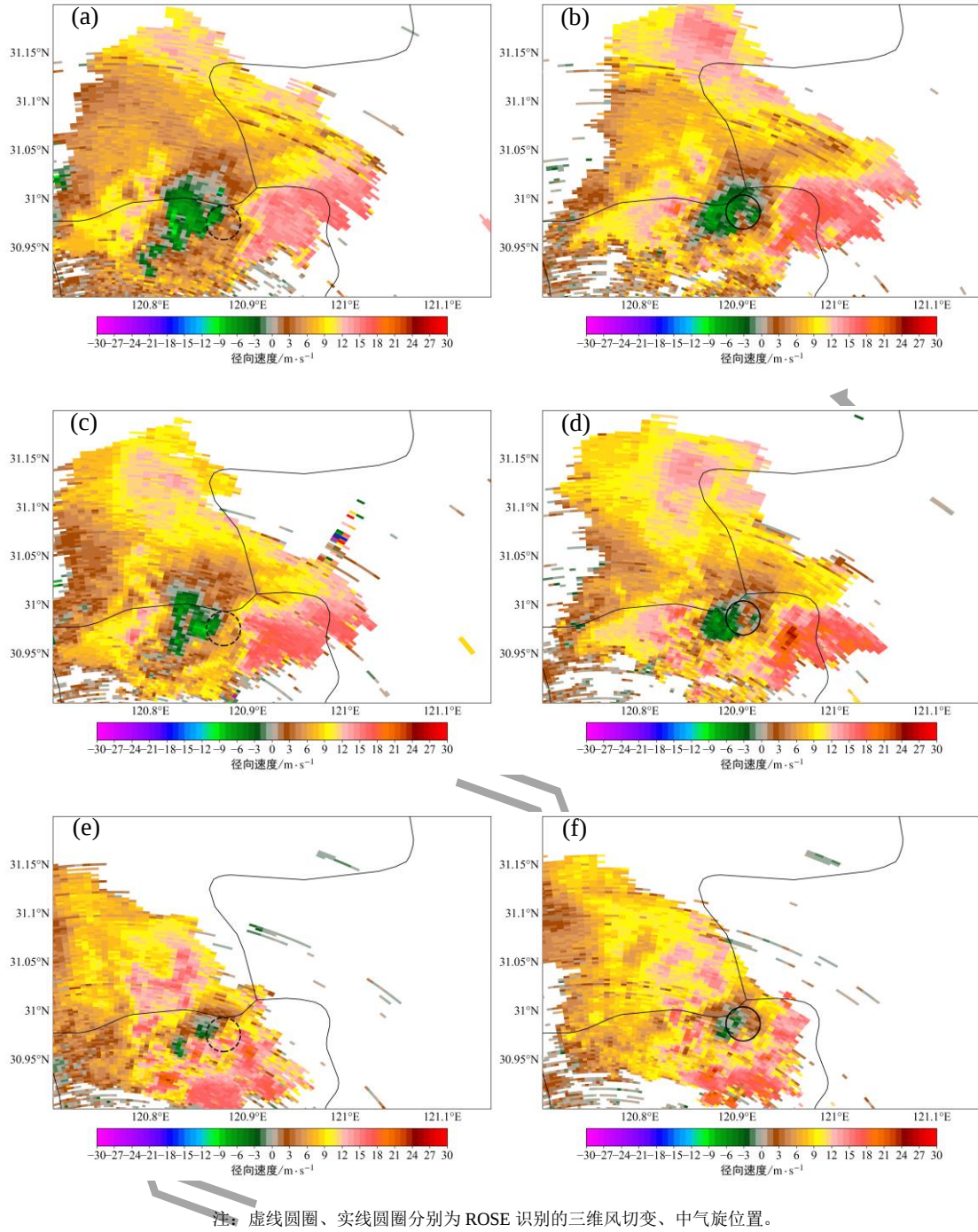
图 7 2024 年 7 月 18 日 (a, c, e) 14:36 和 (b, d, f) 14:42 嘉兴雷达 (VCP216D) (a, b) 7.5°、(c, d) 8.7°和 (e, f) 12°径向速度
