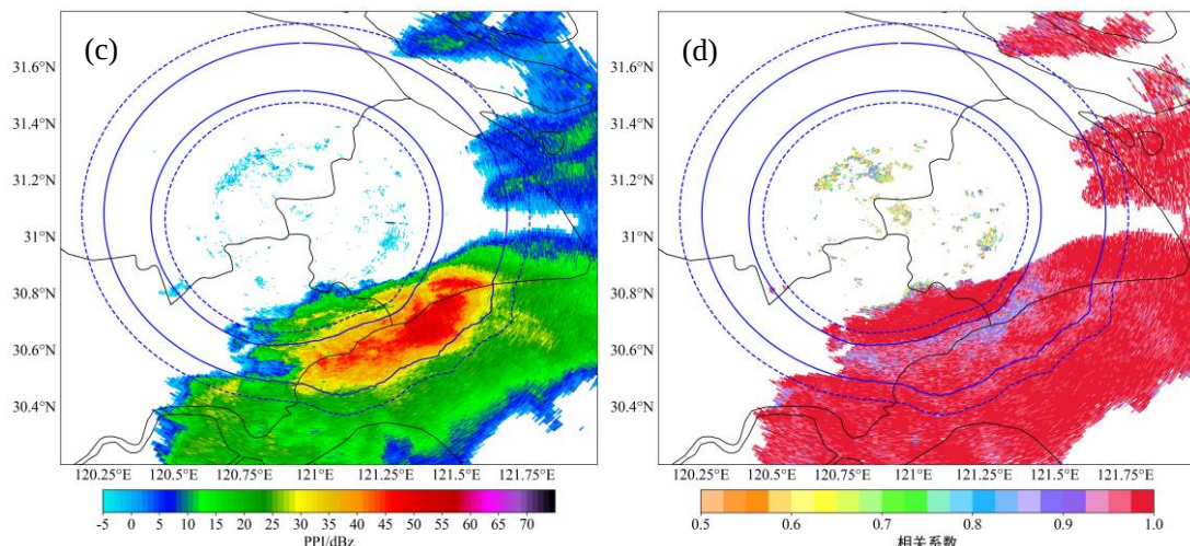
图2 2024年6月12日(a, b) 08:28 杭州雷达(VCP216D) 8.7°仰角和(c, d) 08:26 青浦雷达(VCP211D) 4.3°仰角的(a, c) 反射率因子叠加融化层产品及(b, d) 对应的相关系数
