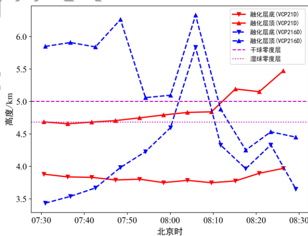
图3 2024年6月12日 07:30—08:30 杭州雷达(VCP216D) 和青浦雷达(VCP211D) 识别融化层高度的时间序列图
