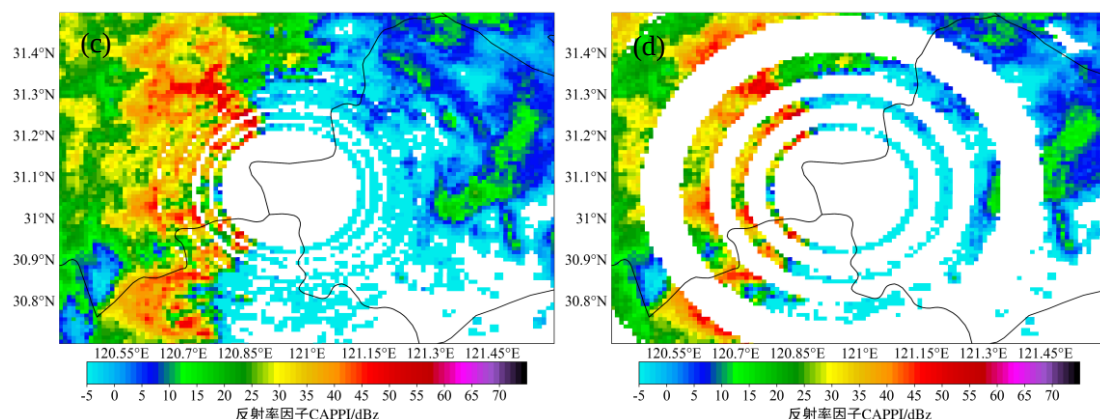
图 8 2024 年 7 月 10 日 20:03 青浦雷达 (a, c) VCP11D 和 (b, d) VCP21D 模式在 (a, b) 5 km 和 (c, d) 6km 高度的 CAPPI 产品
