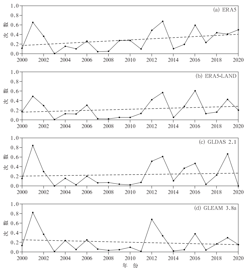
图 10 (a)ERA5,(b)ERA5-LAND,(c)GLDAS 2.1 和(d)GLEAM 3.8a 资料中淮河流域在 2000—2020 年作物生长季逐年骤旱发生次数
