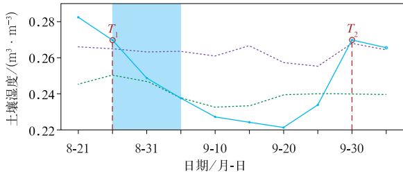
注:紫色虚线和绿色虚线分别为土壤湿度的 40%和 20%分位数阈值,蓝色实线为候平均的土壤湿度,蓝色区域表示骤旱爆发阶段,T 1 、T 2 分别为骤旱开始和结束时间。
