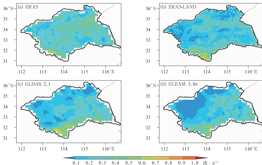
图 7 (a)ERA5,(b)ERA5-LAND,(c)GLDAS 2.1 和(d)GLEAM 3.8a 资料中淮河流域 2000—2020 年骤旱在作物生长季的年平均发生次数
