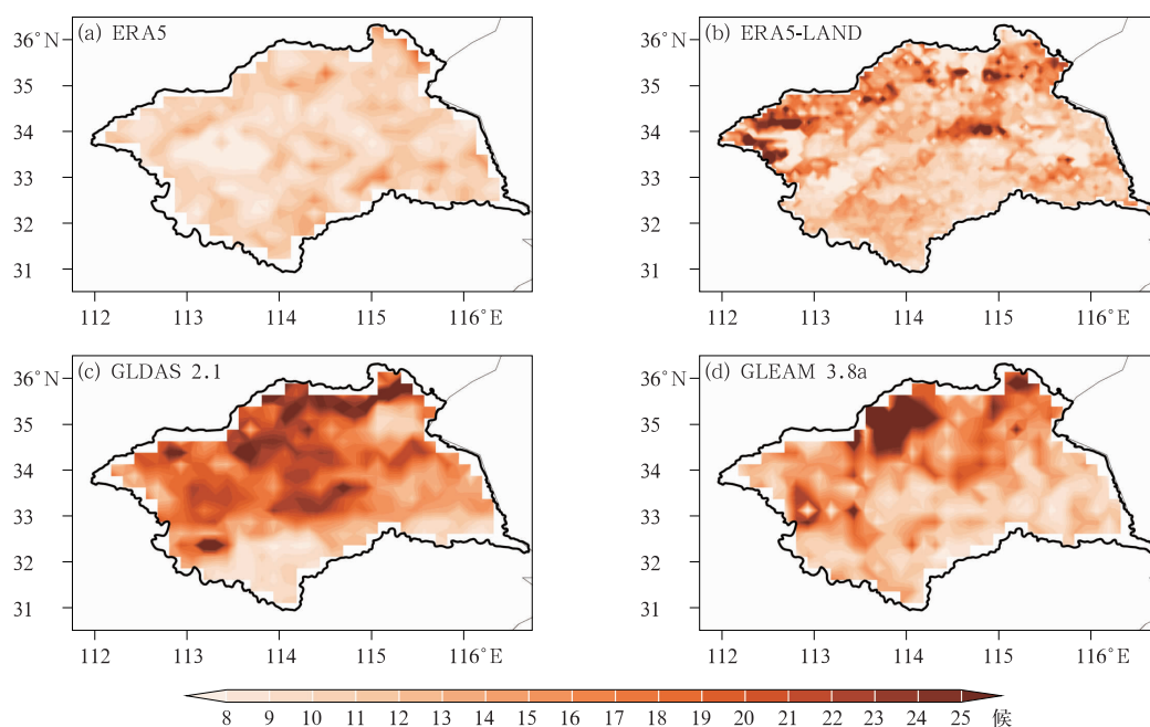
图 3 (a)ERA5, (b)ERA5-LAND, (c)GLDAS 2.1 和 (d)GLEAM 3.8a 资料中淮河流域 2000—2020 年骤旱的平均历时
