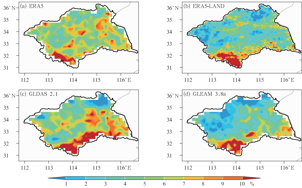
图 9 (a)ERA5,(b)ERA5-LAND,(c)GLDAS 2.1 和(d)GLEAM 3.8a 资料中淮河流域在 2000—2020 年作物生长季的骤旱发生率
