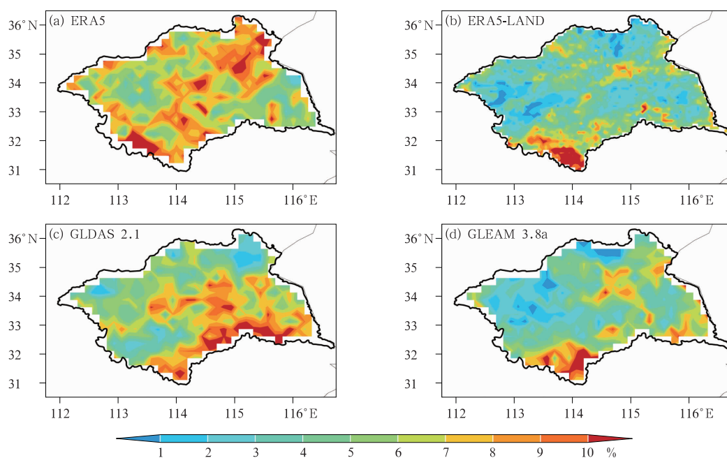
图 4 (a)ERA5, (b)ERA5-LAND, (c)GLDAS 2.1 和 (d)GLEAM 3.8a
