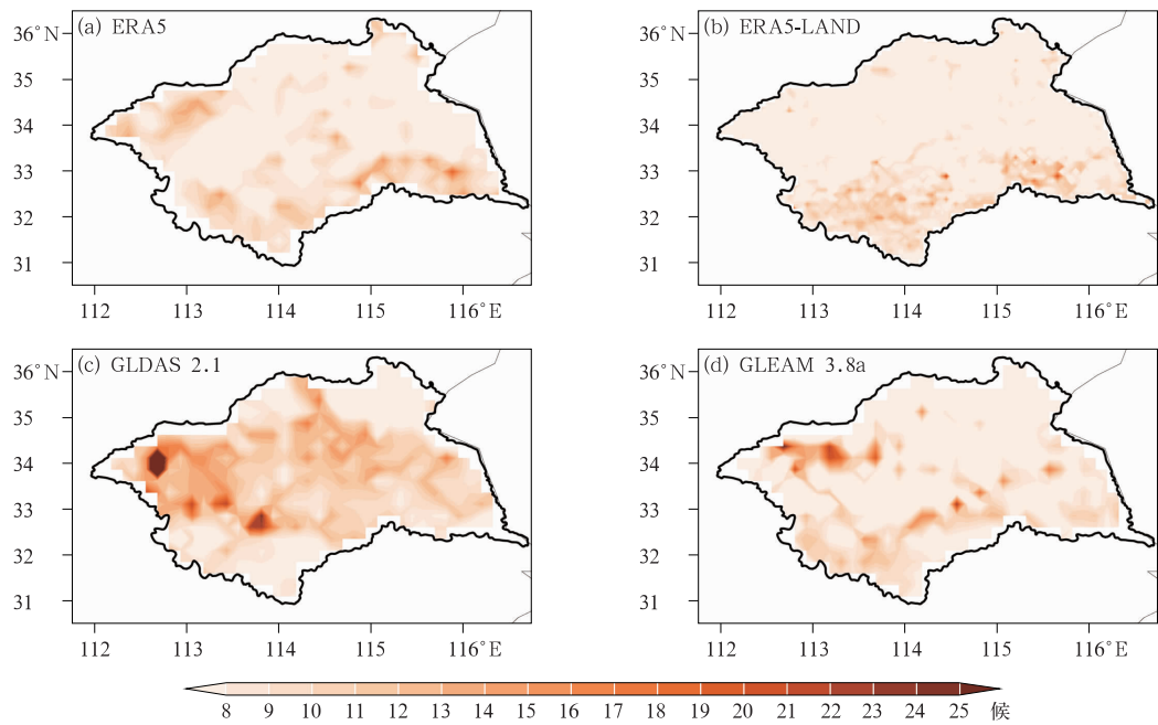
图 8 (a)ERA5,(b)ERA5-LAND,(c)GLDAS 2.1 和(d)GLEAM 3.8a 资料中淮河流域 2000—2020 年骤旱在作物生长季的平均历时
