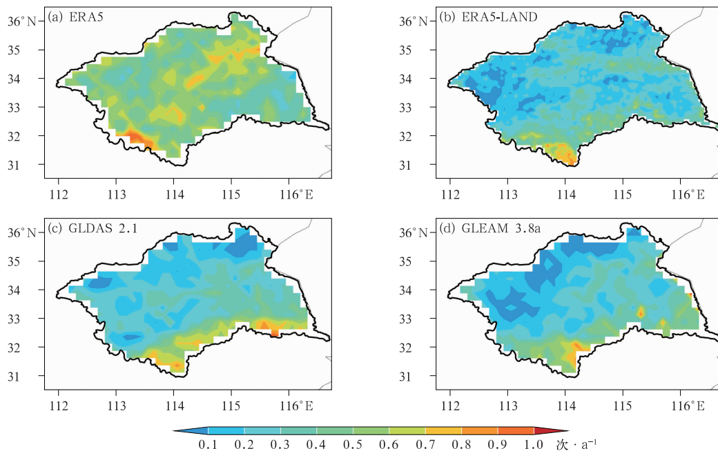
图 2 (a)ERA5,(b)ERA5-LAND,(c)GLDAS 2.1 和(d)GLEAM 3.8a
