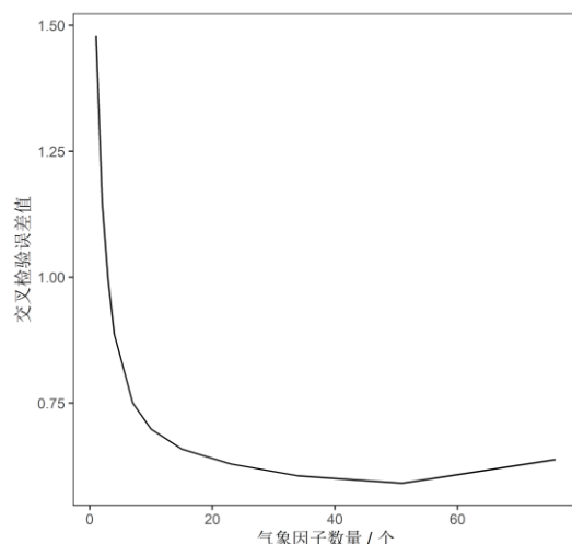
图 3. 溶氧量预测模型因子数量与误差曲线
