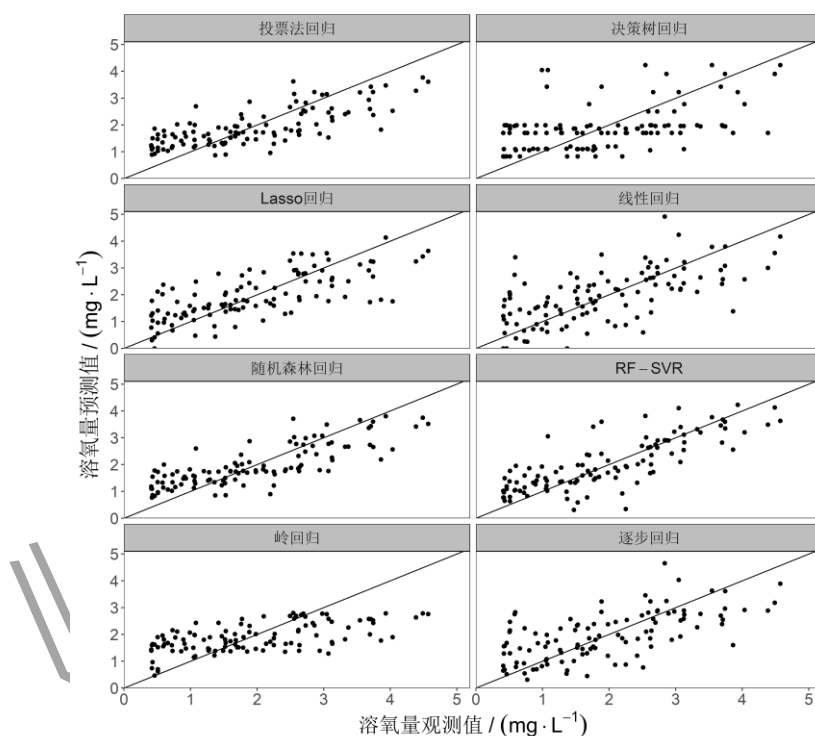
图 5. 8 种溶氧量预测模型预测值与观测值
