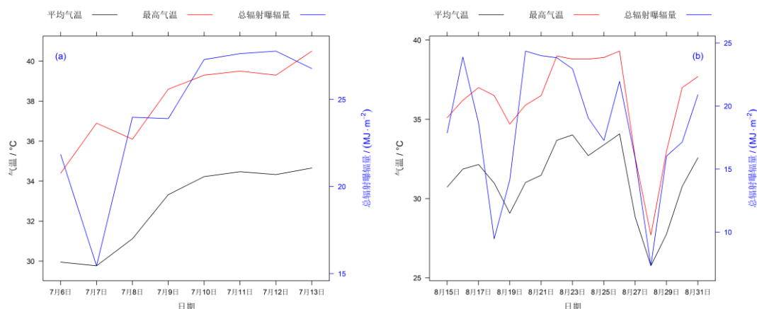
图 1. 洪湖市大同湖农场 (a) 2022 年 7 月 6—13 日, (b) 2025 年 8 月 15—31 日气温及太阳总辐射曝辐量
