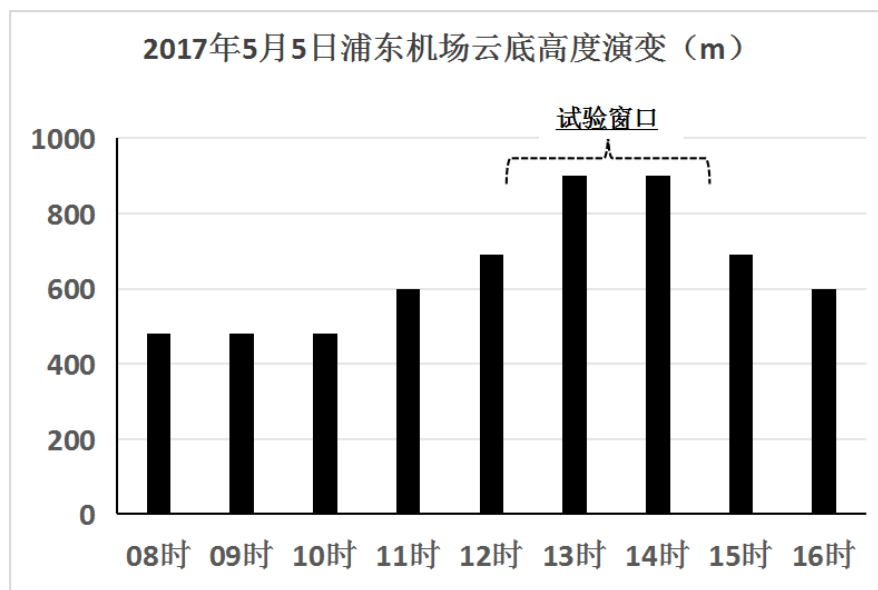
图 7 2017 年 5 月 5 日上海浦东国际机场云底高度时间序列
