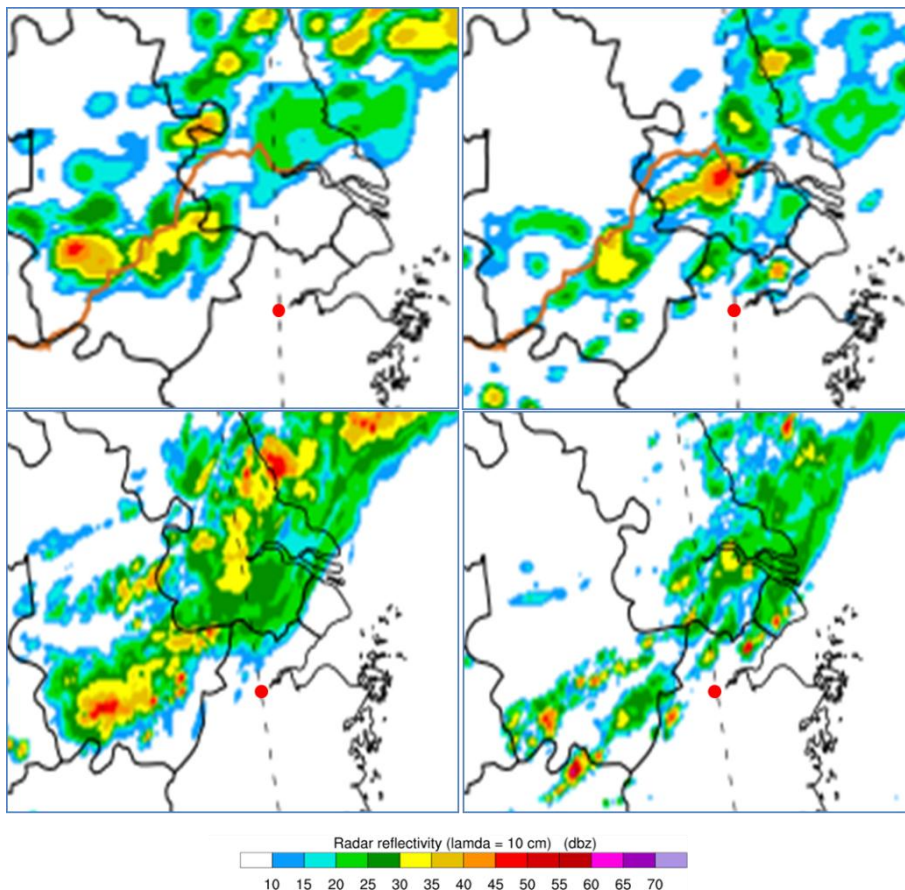
图3 2023年9月20日组合反射率预报
