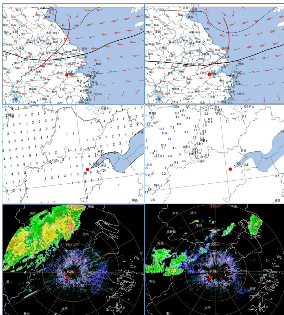
图 2 (a, b, c) EC 模式 2023 年 9 月 19 日 08:00 起报的 20 日 (a,b) 500hPa 高度场 (黑色等值线, 单位: dagpm) 和风场 (风羽), (c) 08:00—14:00 的 6 h 降水量 (数字, 单位: mm), (d) 9 月 20 日 08:00—14:00 的 6 h 降水量实况 (数字, 单位: mm), (e, f) 20 日杭州雷达 0.5°仰角反射率因子 Fig.2 (a, b) 500 hPa geopotential height (black contour, unit: dagpm) and wind (barb), (c) 6 h precipitation from 08:00 BT to 14:00 BT on 20 September initiated at 08:00 BT 19 September by EC model, (d) 0.5° elevation reflectivity factor at Hangzhou Radar on 20 September 2023
