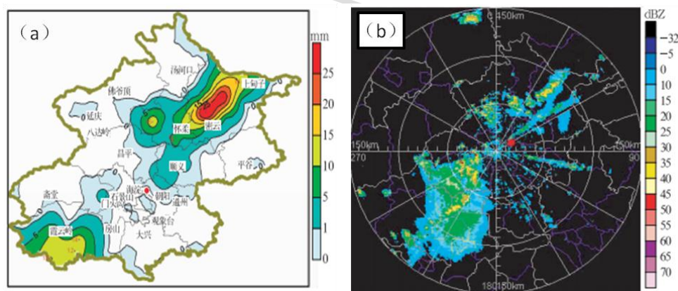
图 1 2008 年 8 月 (a) 8 日 19:00 至 9 日 01:00 北京累计降水量和 (b) 8 日 21:40 北京多普勒雷达组合反射率因子（引自杨波等，2010）
