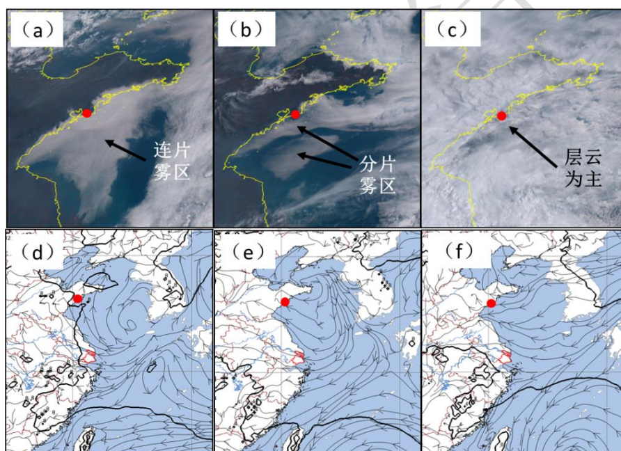
图 5 2018 年 6 月 7—9 日 (a~c) 可见光云图, (d~f) EC 模式 6 日 20:00 起报的 1000hPa 高度场 (等值线, 单位: hPa) 和地面流场 (流线) 零场
