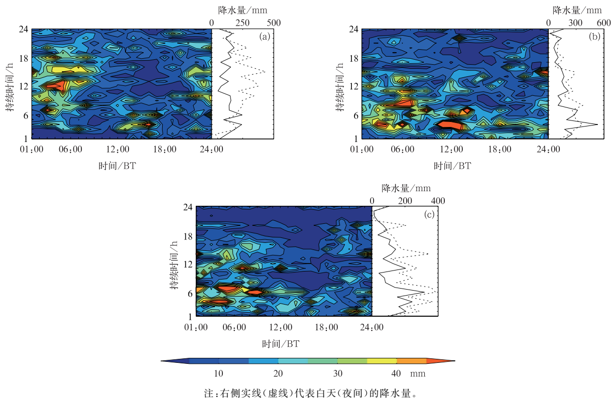
图 3 (a)山顶站、(b)山腰站、(c)坝区站不同持续时间的降水量变化
