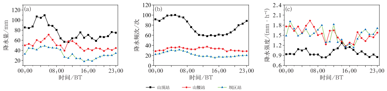
图 2 山顶站、山腰站和坝区站的(a)降水量、(b)降水频次和(c)降水强度日变化
