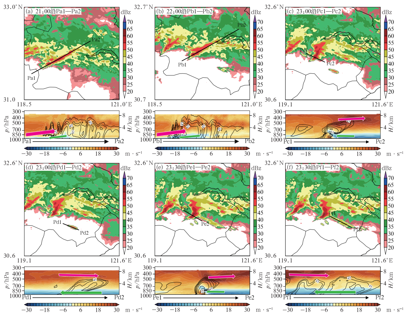
图 6 2017 年 9 月 24 日(上)模式模拟组合雷达反射率因子,(下)沿图中黑色直线的水平风速(填色,正值方向为起点指向终点)和雷达反射率因子的垂直剖面(黑色等值线,单位: dBZ)
