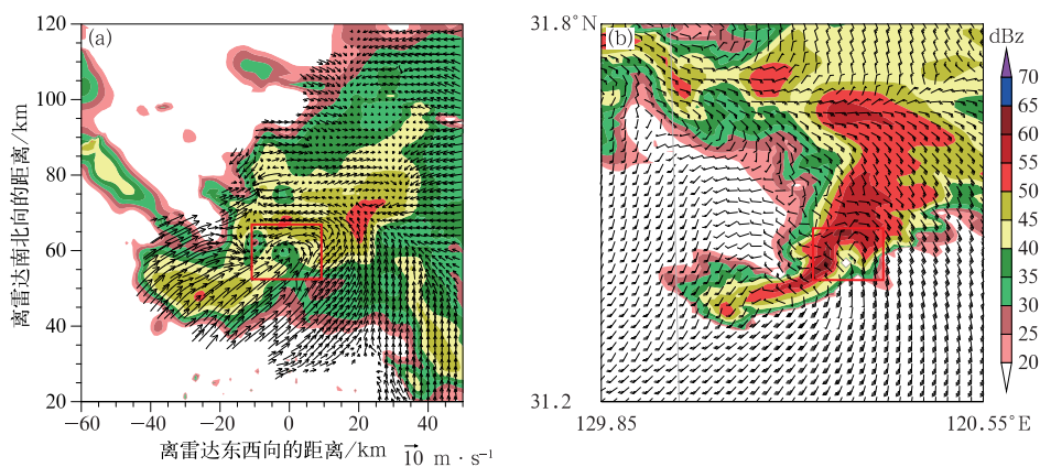
图 7 2017 年 9 月 25 日 (a) 00:30 利用青浦和南通双多普勒雷达风场反演和(b)00:00 模式模拟的 1 km 高度雷达反射率因子(填色)和水平风场(风矢,风羽)
