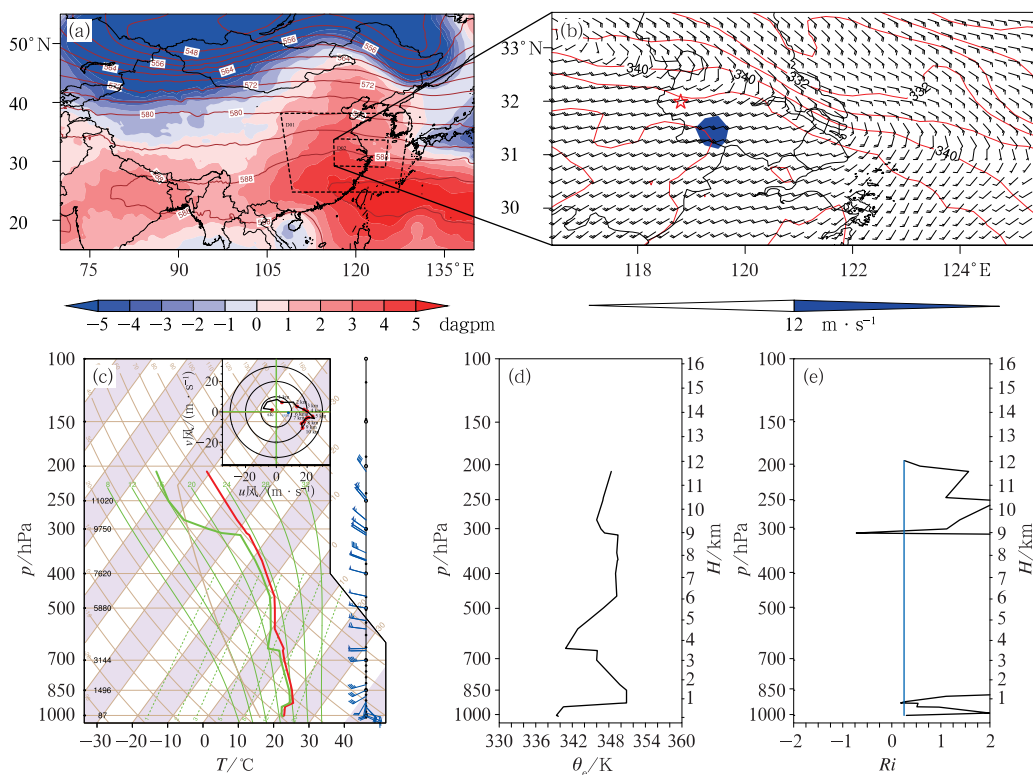
图 2 2017 年 9 月 24 日 20:00(ERA5 分析资料的 500 hPa 位势高度场(等值线,单位:dagpm)和其与 9 月气候平均(1979—2016 年)位势高度场偏差(填色),(b)图 a 中 D02 范围内 ERA5 分析资料的 850 hPa 风场(风羽)、相当位温(等值线,单位:K)和 \geq 12 \text{ m} \cdot \text{s}^{-1} 风速(填色),(c)南京站探空和速度矢端图,(d,e)南京站探空计算的(d)相当位温和(e)Ri 随高度的分布
