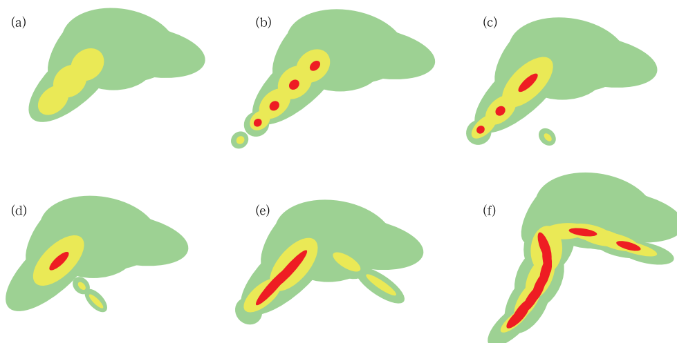
图 11 雷达组合反射率因子演变概念模型
