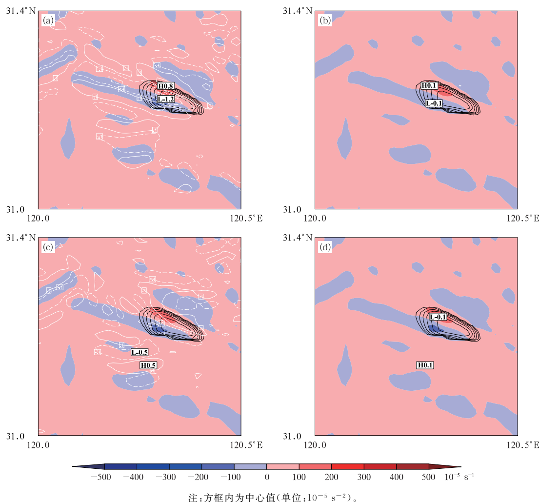
图 10 2017 年 9 月 24 日 23:00 模式模拟的回波 C 处 1 km 高度雷达反射率因子(黑色等值线,单位: dBZ)、 涡度(填色)、涡度方程各项(白色等值线)
