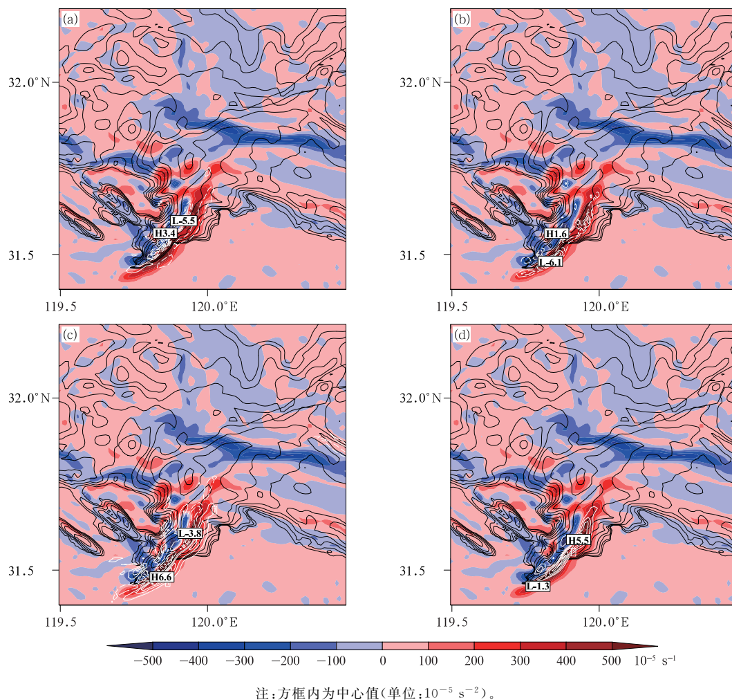
图 9 2017 年 9 月 24 日 23:00 模式模拟的回波 A 处 1 km 高度雷达反射率因子 (黑色等值线, 单位: dBz)、涡度 (填色)、涡度方程各项 (白色等值线)
