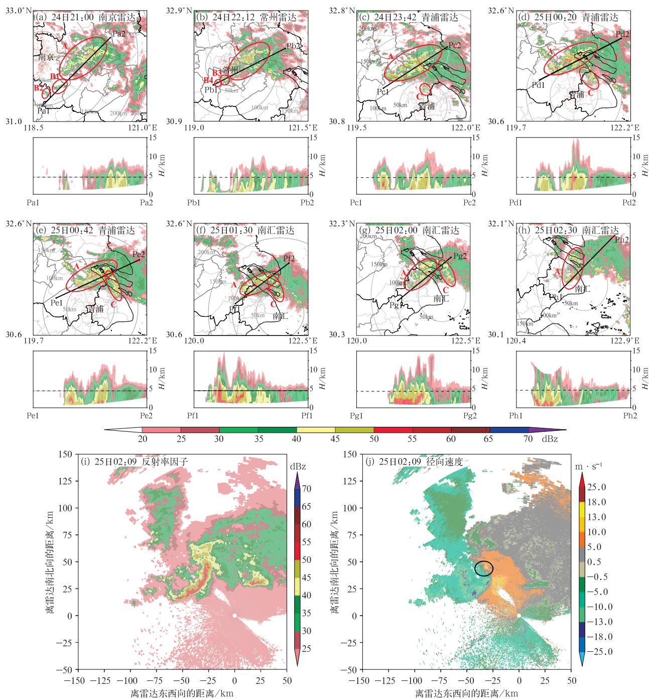
注:图 a~图 h 中,黑色虚线为融化层高度,红色椭圆及字母用于追踪主要对流系统的演变; 图 j 中,黑色椭圆为弓形回波北侧的气旋式涡旋。
