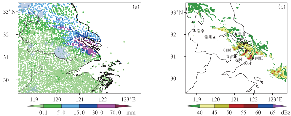
注:图b中黑色三角形为南京、常州、南通、青浦和南汇5部雷达所在位置。
