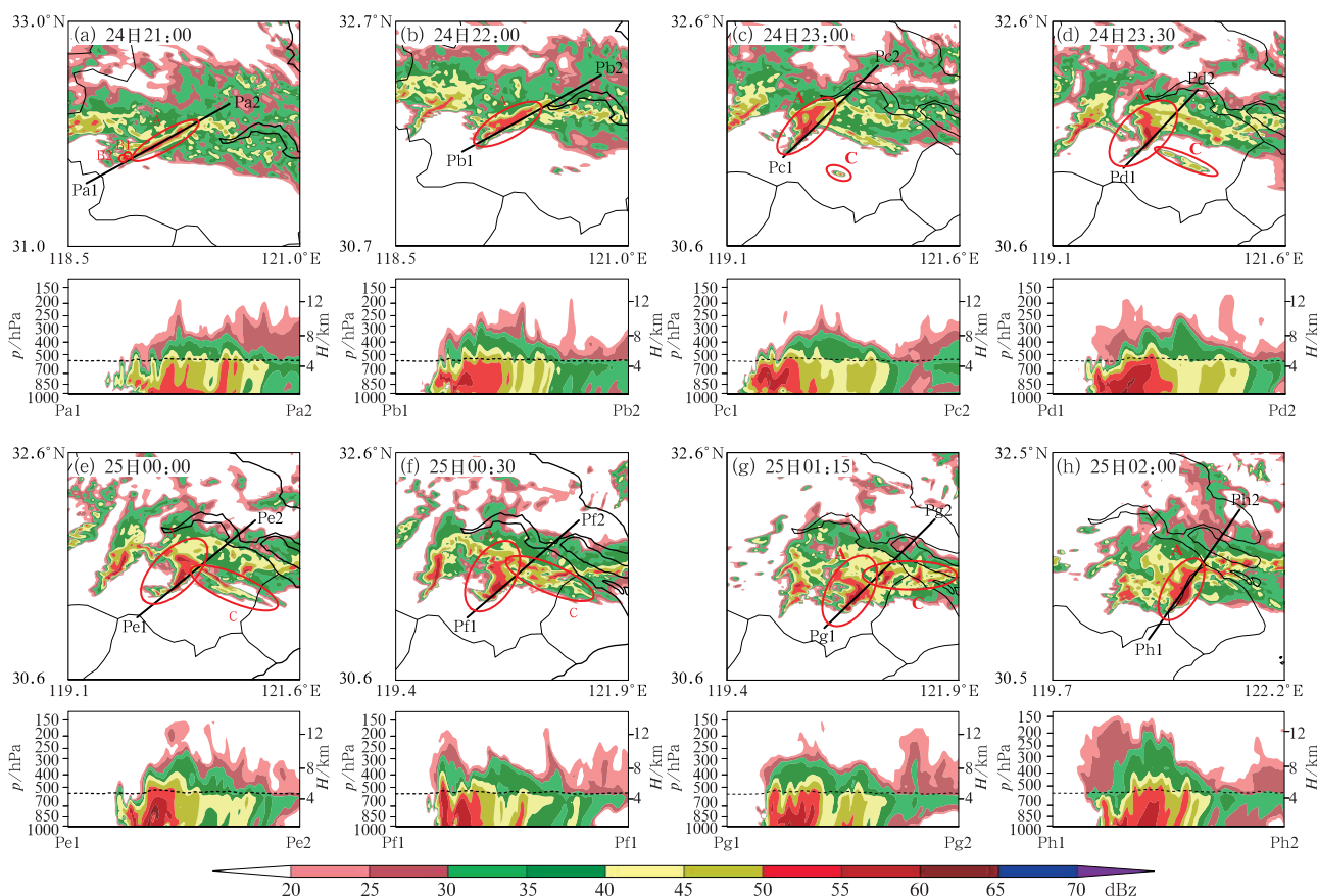
图 5 2017 年 9 月 24—25 日(上)模式模拟底层雷达反射率因子和 (下)沿图中黑色直线的雷达反射率因子垂直剖面
