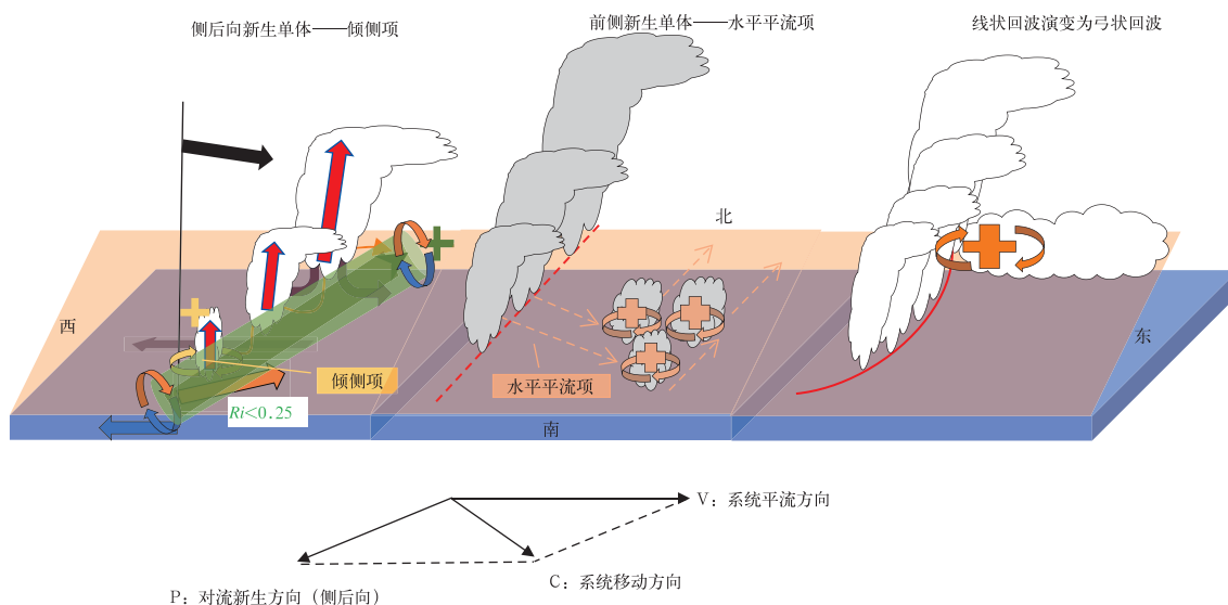
图 12 \beta 中尺度对流系统演变为弓形的立体概念模型和系统移动方向合成矢量图
