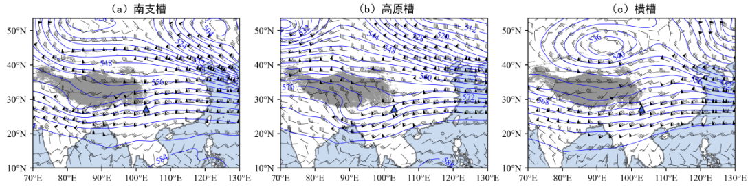
图 3 2018—2021 年白鹤滩水电站三类大风环流形势的 500 hPa 位势高度场（等值线）和风场（风羽）
