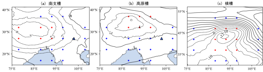
图 6 白鹤滩水电站 (a) 2018 年 1 月 25 日南支槽型、(b) 2019 年 1 月 14 日高原槽型和 (c) 2018 年 1 月 6 日横槽型大风时 500 hPa 与 1 月平均位势高度距平分布 (等值线, 单位: dagpm, )
