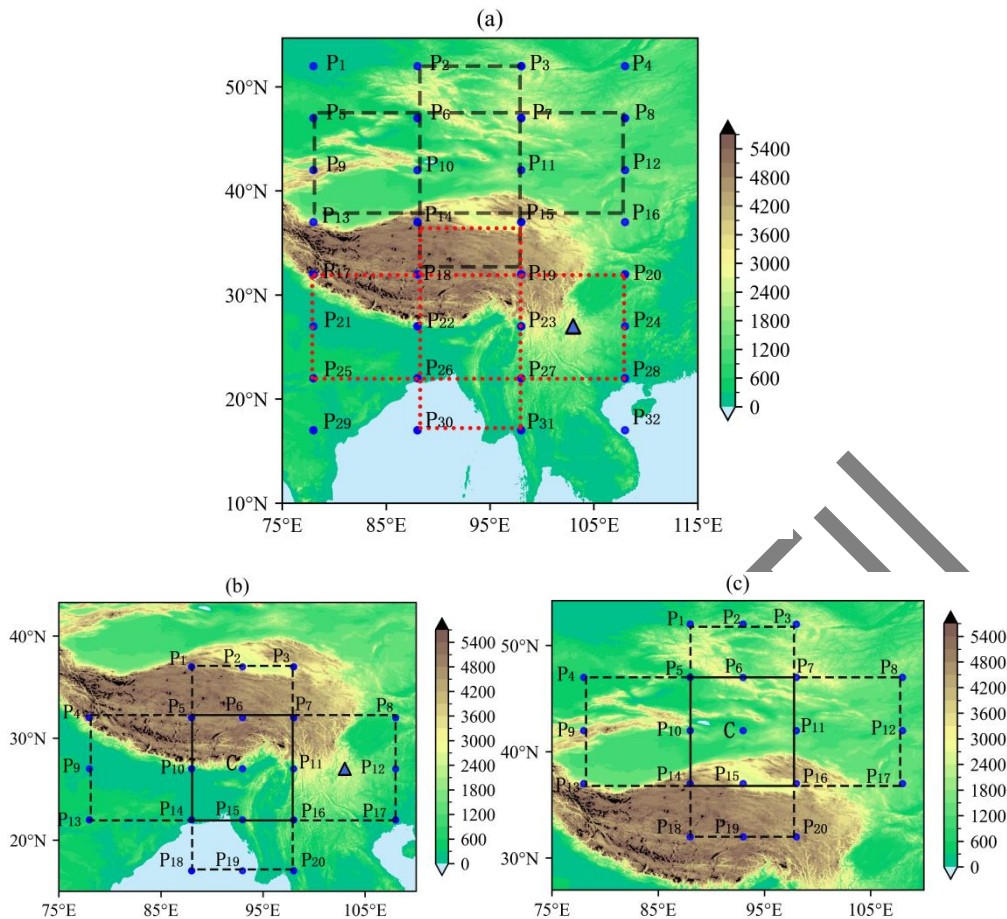
注：填色为海拔，单位：m；蓝点为选取的计算环流指数格点； P_x 为格点序号；三角形为白鹤滩水电站位置。图 a 中黑色十字型框为北部区域，红色十字型框为南部区域。图 b, c 中 C 为选取的中心点。
