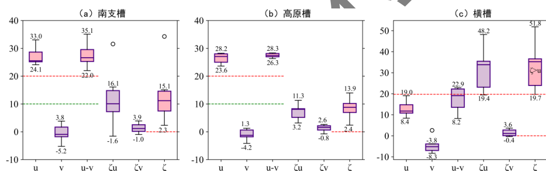
注：箱型图上、下横线分别为环流指数最大值和最小值，圆圈为极端值，中间线为中位数，箱体上、下线分别为上四分位数和下四分位数，粉色和紫色箱体分别为判识所用和未用环流指数；红线和绿线分别为调整前和调整后环流指数条件。
