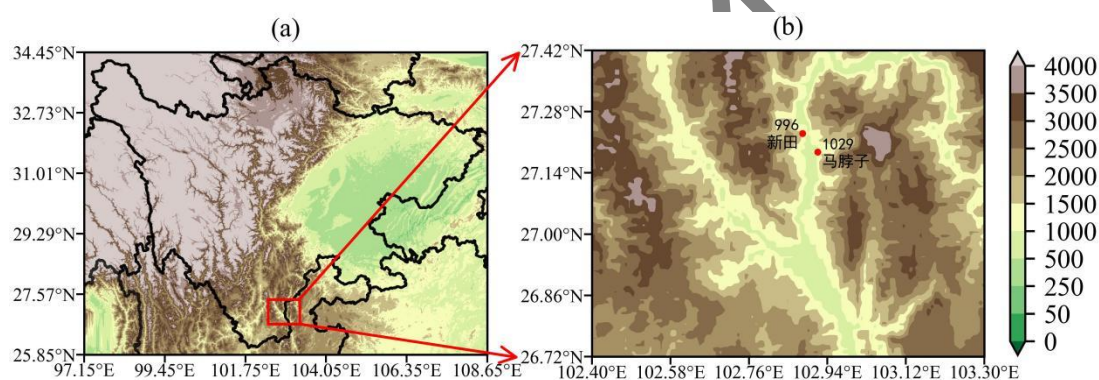
注: 填色为海拔, 单位: m。图 a 中方框为水电站位置。图 b 为图 a 方框放大; 红点为观测站; 数值为观测站海拔, 单位: m。
