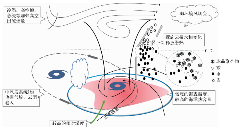
图 3 TC 近海加强影响因子模型
