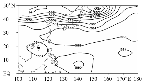
图1 副高与近海加强 TC 的相对位置(引自胡春梅等,2005)
