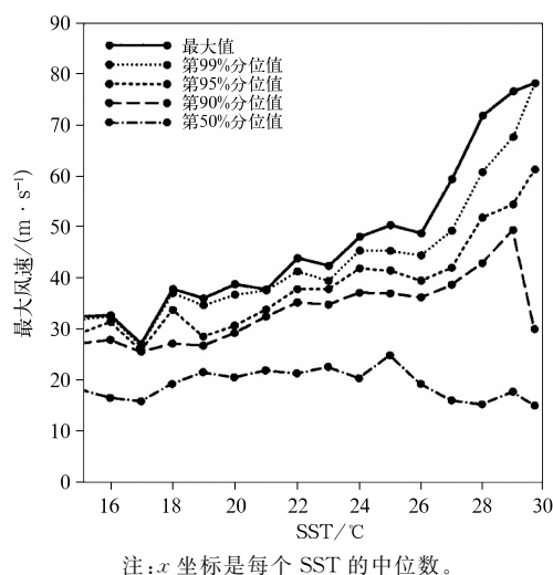
图2 1^{\circ}\text{C} 海温组的最大风暴强度和第 99%、95%、90% 和 50% 分位值强度随 SST 的变化(引自 DeMaria and Kaplan, 1994)
