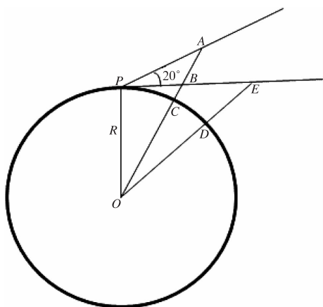
图2 理想条件下天气雷达顶部 盲区半径和覆盖半径
