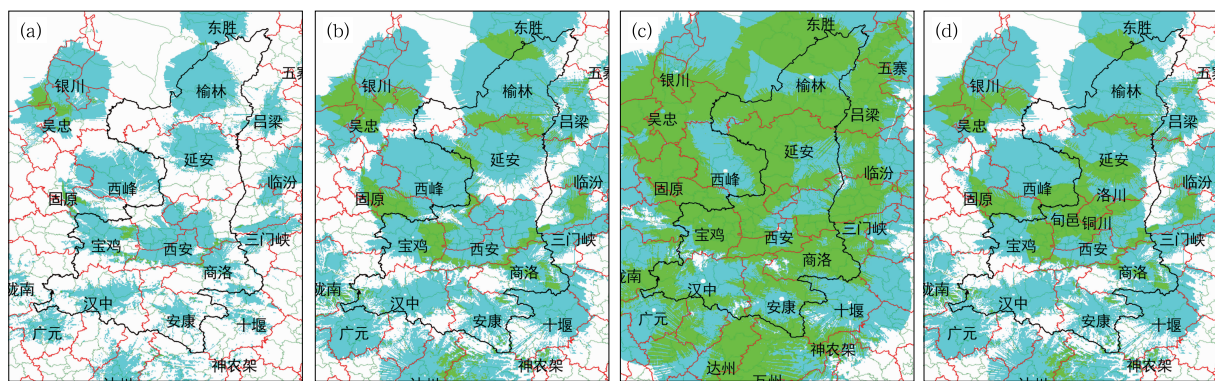
图 6 陕西新一代天气雷达在(a)0.5 km,(b)1 km,(c)2 km 高度和(d)增加 3 部 X 波段雷达后 1 km 高度的覆盖范围
