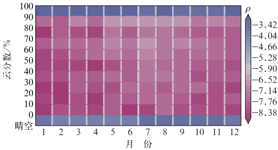
图 7 2016 年 1 月 1 日至 2020 年 12 月 31 日 观测期间每月不同云分数分布特征 Fig. 7 Different distribution characteristics of cloud fraction each month during the observation period from 1 January 2016 to 31 December 2020
