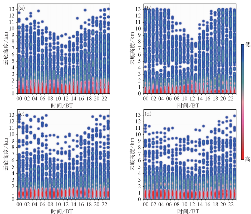
图 4 2016 年 1 月 1 日至 2020 年 12 月 31 日 (a) 春季, (b) 夏季, (c) 秋季, (d) 冬季各时段的云底高度频次分布
