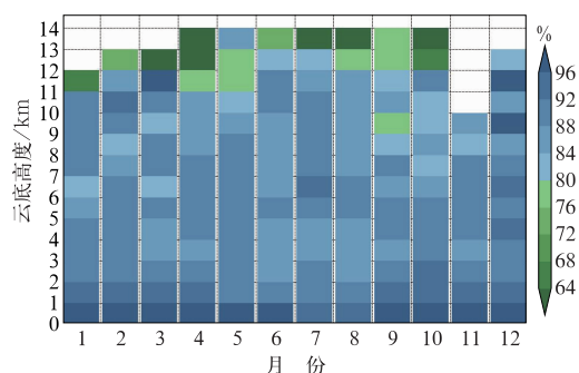
图 10 2016—2020 年各月云分数时空分布
