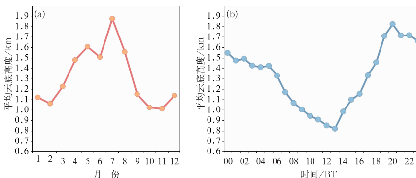
图3 2016年1月1日至2020年12月31日(a)月份和(b)小时的平均云底高度变化
