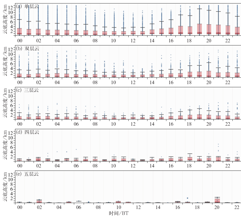
图 5 2016 年 1 月 1 日至 2020 年 12 月 31 日单层至五层云的云底高度盒须图
