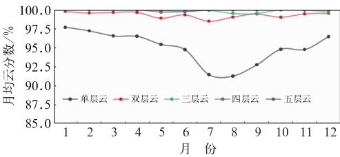
图 8 2016 年 1 月 1 日至 2020 年 12 月 31 日 不同云层月均云分数变化 Fig. 8 Variation of monthly average cloud fraction in each layer from 1 January 2016 to 31 December 2020
