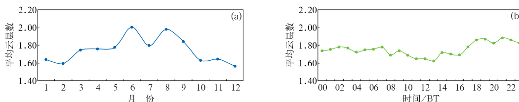
图2 2016年1月1日至2020年12月31日(a)月份和(b)小时的平均云层数变化
