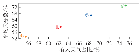
图 9 2016 年 1 月 1 日至 2020 年 12 月 31 日 各季节有云天气占比及平均云分数
