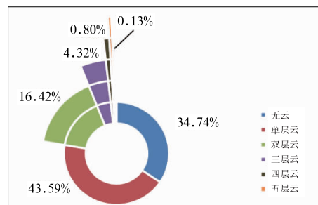
图1 2016年1月1日至2020年12月31日无云及单层、双层、三层、四层、五层云的概率分布
