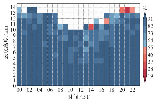
图 11 2016 年 1 月 1 日至 2020 年 12 月 31 日 云分数时空分布(时段)
