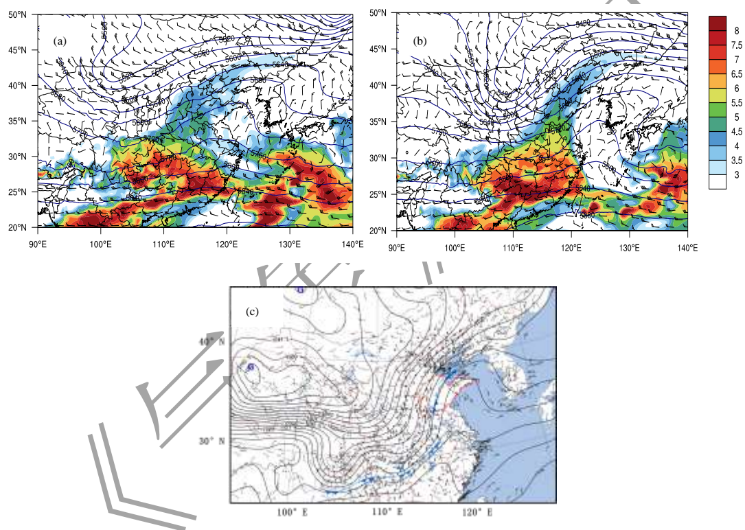
图2 2021年11月(a)6日20时和(b)7日08时500 hPa高度场(等值线, 单位: gpm)、700 hPa风场(单位: \text{m} \cdot \text{s}^{-1} )和比湿(填色, 单位: \text{g} \cdot \text{kg}^{-1} ), (c)7日08时地面气压场(单位: hPa)、风场(单位: \text{m} \cdot \text{s}^{-1} )和天气现象(填图符号)
