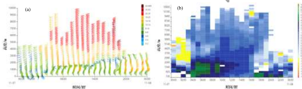
图 3 2021 年 11 月 7 日 00 时至 8 日 00 时章丘风廓线雷达的 (a) 风羽图和 (b) 垂直速度(单位: \text{m}\cdot\text{s}^{-1} )
