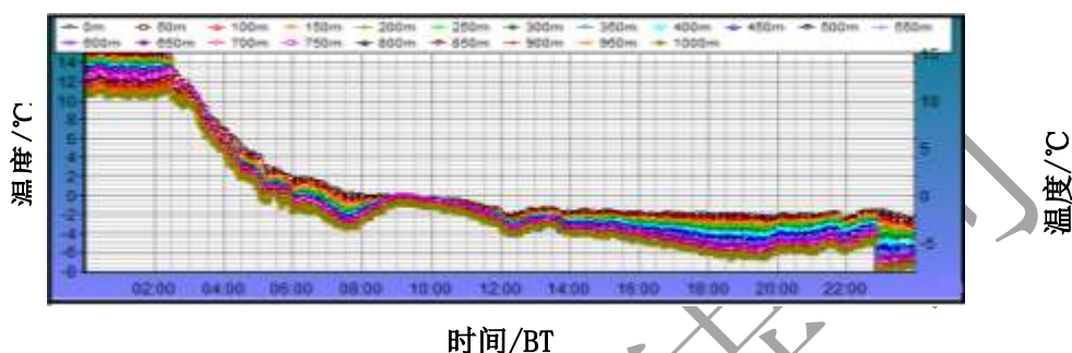
图7 2021年11月7日00—23时济南边界层温度(单位:℃)垂直分布随时间变化
