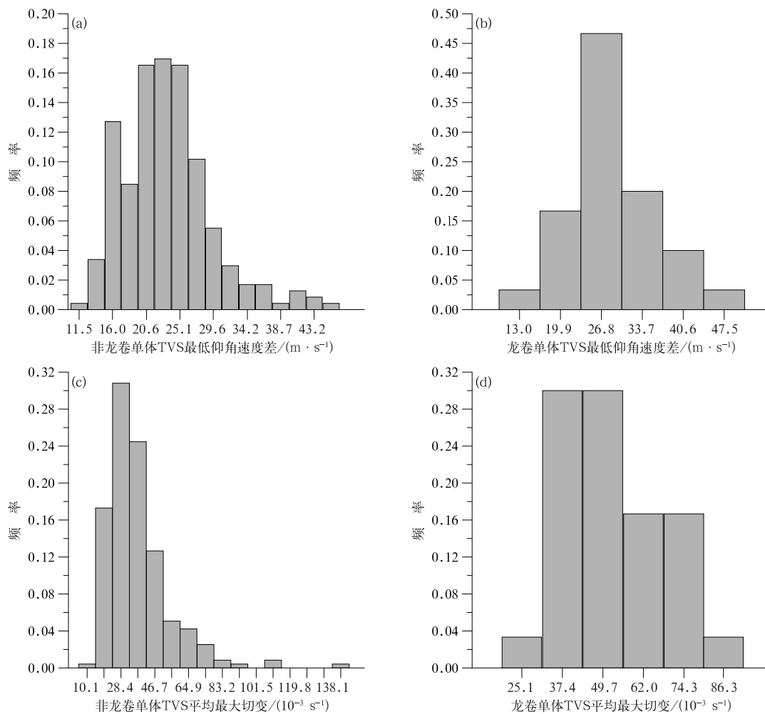
图8 2007—2018年江苏台风龙卷天气中龙卷与非龙卷单体TVS关键特征分布
