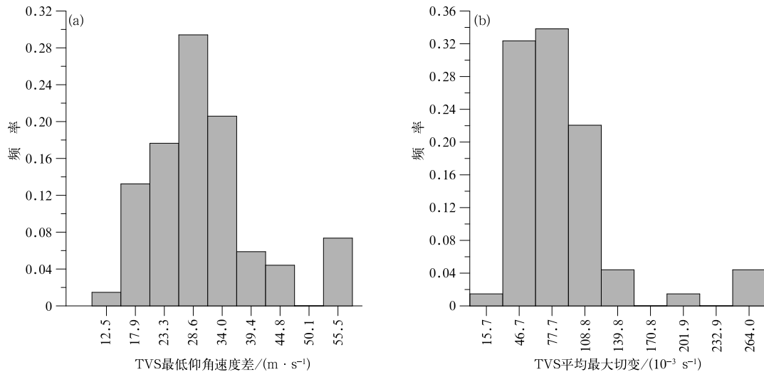
图 9 广东台风龙卷 TVS 关键特征分布
