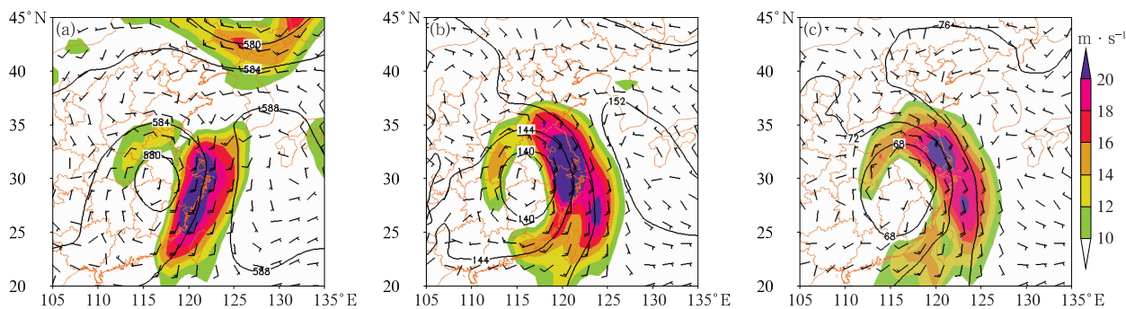
图 5 江苏 9 次台风龙卷过程环流形势合成(实线:等高线,单位:dagpm;填色和风羽:风速) (a)500 hPa,(b)850 hPa,(c)925 hPa
