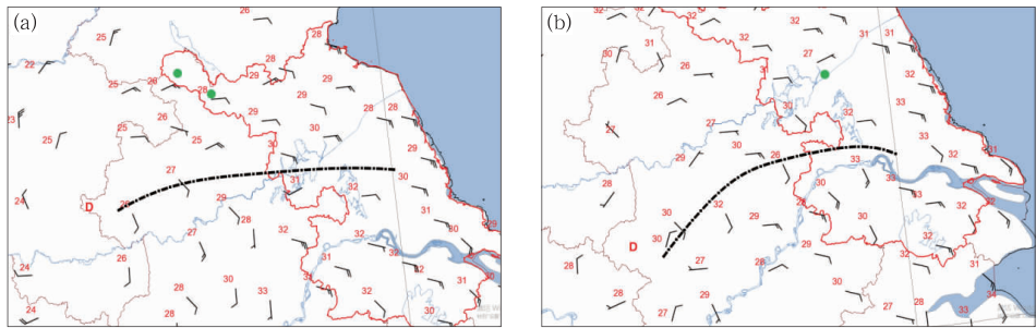
图 7 (a)2018 年 8 月 18 日 17 时和(b)2017 年 8 月 1 日 17 时地面填图 (绿色圆点为龙卷发生地)
