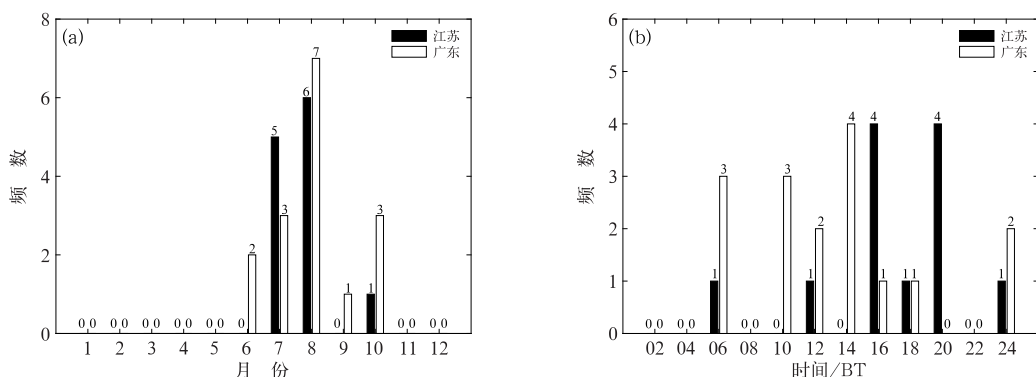
图1 2007—2018年江苏和广东台风龙卷的(a)月分布特征和(b)日变化分布对比
