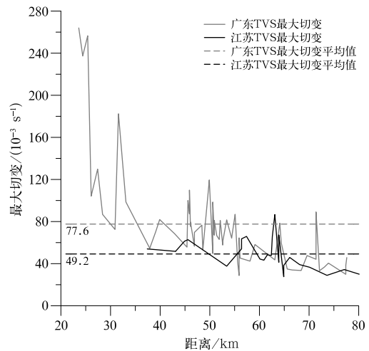
图 10 江苏、广东两地台风龙卷 TVS 最大切变与距离分布
