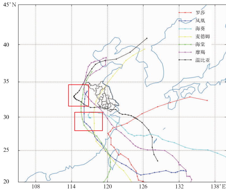
图 3 2007—2018 年引发江苏龙卷的台风路径 (红框表示出现龙卷时台风中心位置)
