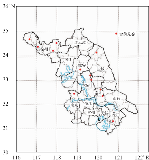
图2 2007—2018年江苏台风龙卷地域分布特征
