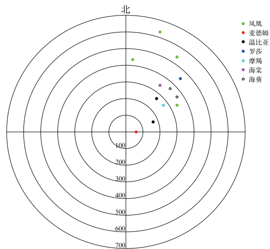
图 4 2007—2018 年江苏龙卷发生地与台风中心的位置关系 (单位: km)
