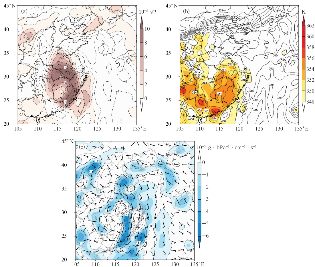
图 6 江苏 9 次台风龙卷过程的(a)850 hPa 涡度、(b)假相当位温( \theta_{se} )及(c)水汽通量散度与风场的合成
