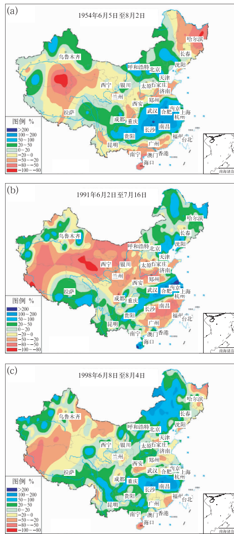
图 9 1954 年(a), 1991 年(b)和 1998 年(c) 梅雨期降水距平百分率的空间分布 Fig. 9 Distribution of the rainfall anomaly percentage rate in the Meiyu season (a) 1954, (b) 1991, (c) 1998
