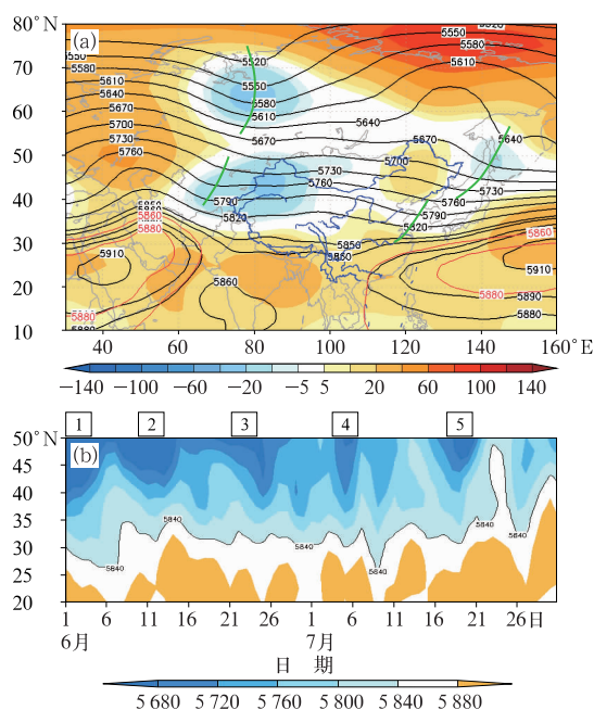
图8 2020年梅雨期(a)平均500 hPa位势高度场的空间分布和(b)110°~122.5°E
