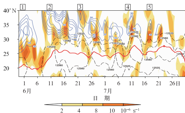
图 6 2020 年梅雨期 110^{\circ}\sim 122.5^{\circ}\text{E} 平均的 200 hPa 位势高度场(黑色虚线,单位:gpm), 纬向风(蓝色细实线,单位: \text{m}\cdot\text{s}^{-1} )和水平散度(填色)的时间-纬度剖面图(红色粗实线代表南亚高压脊线,图片上方的数字表示 5 次东亚高空西风急流的加强过程)
