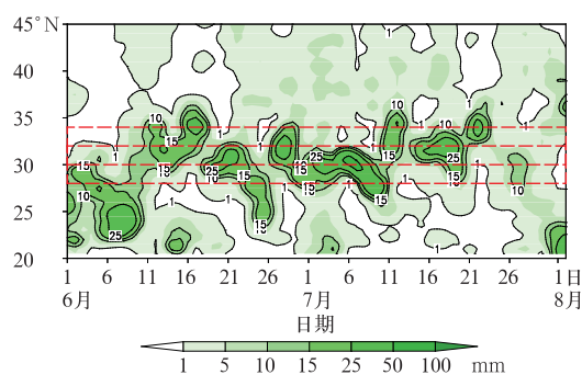
图 3 2020 年梅雨期沿 110^{\circ}\sim 122.5^{\circ}\text{E} 平均的逐日降水量的时间-纬度剖面 [红色虚线代表梅雨监测区,从南至北分别代表江南区( 28^{\circ}\sim 30^{\circ}\text{N} ),长江中下游区( 30^{\circ}\sim 32^{\circ}\text{N} )和江淮区( 32^{\circ}\sim 34^{\circ}\text{N} )]
