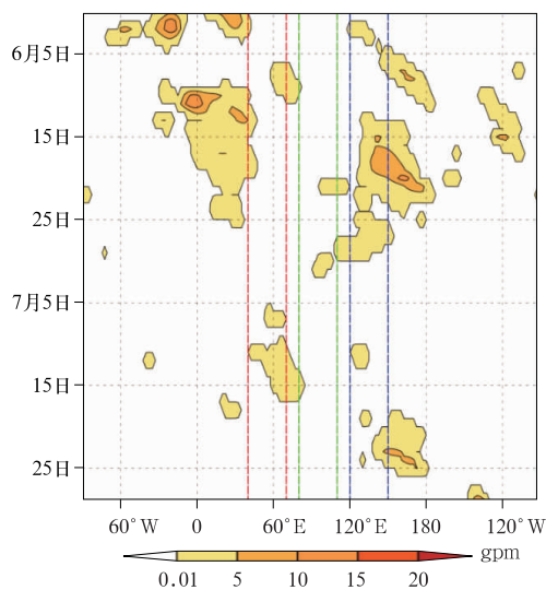
图 7 2020 年梅雨期北半球中高纬度阻塞高压强度的时间-经度剖面
