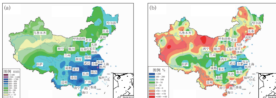
图 2 2020 年 6 月 1 日至 8 月 2 日梅雨期(a)累计降水量和(b)降水距平百分率的空间分布
