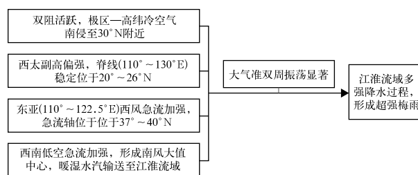
图 10 超强梅雨形成的大气环流条件框图
