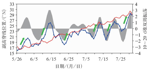
图 4 2020 年梅雨期 110^{\circ}\sim 130^{\circ}\text{E} 副高脊线位置的逐日演变 (红线为气候平均值,绿色箭头代表副高的北抬过程,灰色阴影代表经 10\sim 20\text{ d} 滤波后的准双周振荡分量)
