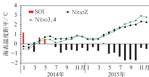
图 5 2014—2015 年 NinoZ 和 Nino3.4 海温指数(单位: ^{\circ}\text{C} )及南方涛动指数(SOI)逐月演变 Fig. 5 Monthly variation of sea surface temperature index (unit: ^{\circ}\text{C} ) and southern oscillation index (SOI) of NinoZ and Nino3.4 during 2014–2015
