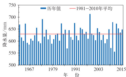
图 3 1961—2015 年全国平均年降水量历年变化
