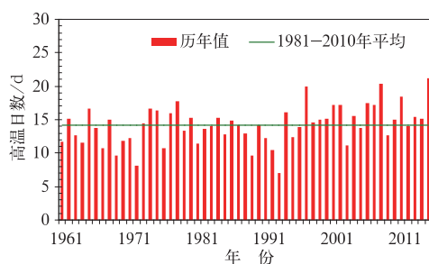
图9 1961—2015年新疆夏季高温 日数历年变化
