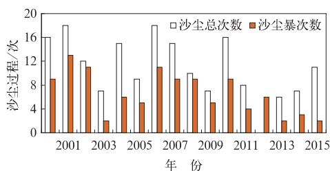
图10 2000—2015年春季北方沙尘天气过程历年变化
