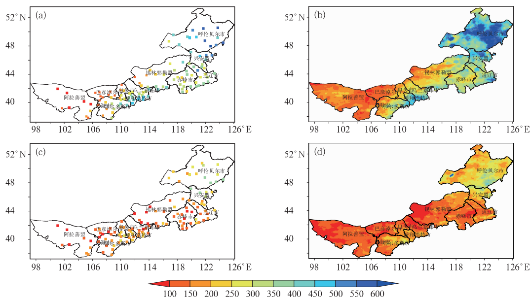
图 1 2013 和 2014 年夏季内蒙古地区站点观测降水(a, c)与 CLDAS 资料降水(b, d)空间分布(单位: mm)
