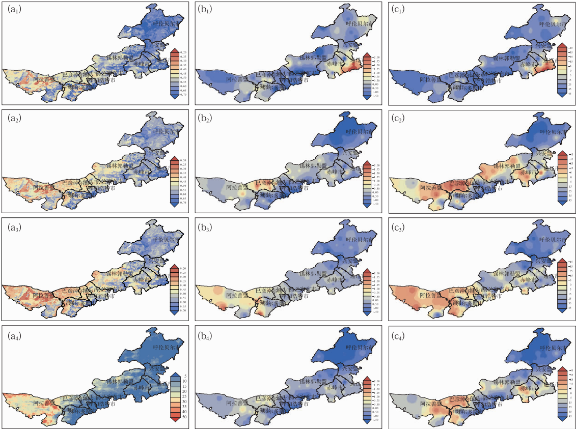
图 5 2013 年内蒙古地区 RSM 、 DNP 、 SPI 、 PDECI 干旱指数分布 (说明同图 4)
