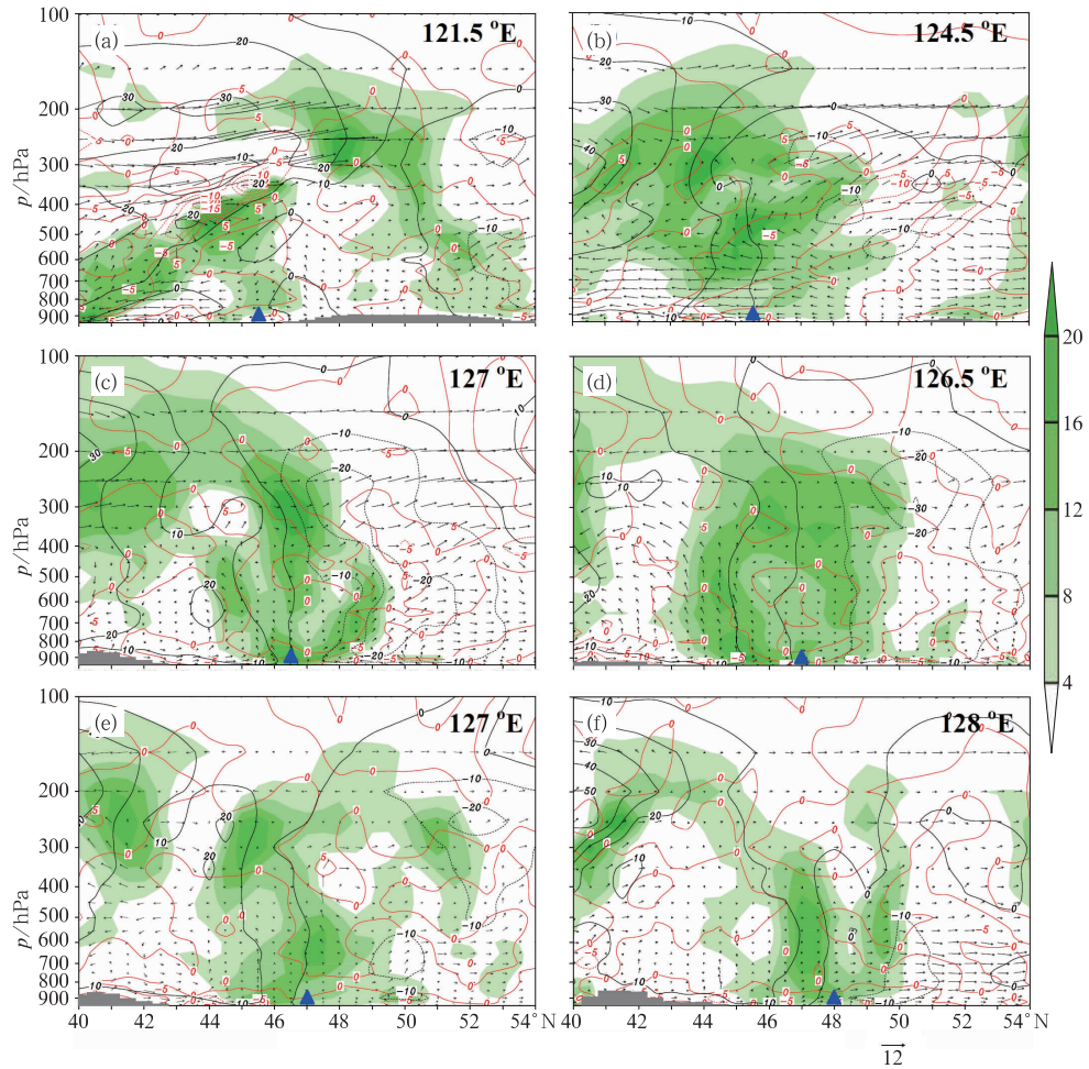
图 6 2013 年 7 月 2—4 日沿涡旋中心经度(图右上角)的涡度(阴影,单位: 10^{-5} \text{ s}^{-1} ) 散度(红色实线和虚线,单位: 10^{-5} \text{ s}^{-1} )、纬向风(黑色实线和虚线,单位: \text{m} \cdot \text{s}^{-1} ) 以及经向风和 50 \times 垂直速度(箭头,单位: \text{m} \cdot \text{s}^{-1} )的剖面 (底部灰色填色代表地形)
