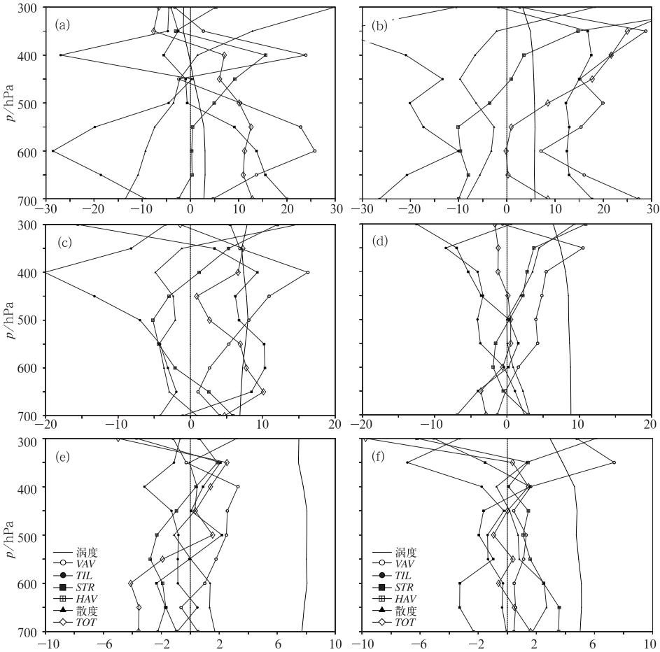
图 7 2013 年 7 月 1—4 日关键区区域平均的涡度收支项(单位: 10^{-10} \text{ s}^{-2} )、 涡度(单位: 10^{-5} \text{ s}^{-1} )和散度(单位: 10^{-6} \text{ s}^{-1} )
