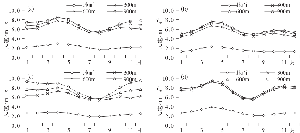
图 1 边界层内不同高度风速月际变化图 (a) 3 站平均; (b) 邢台; (c) 张家口; (d) 乐亭
