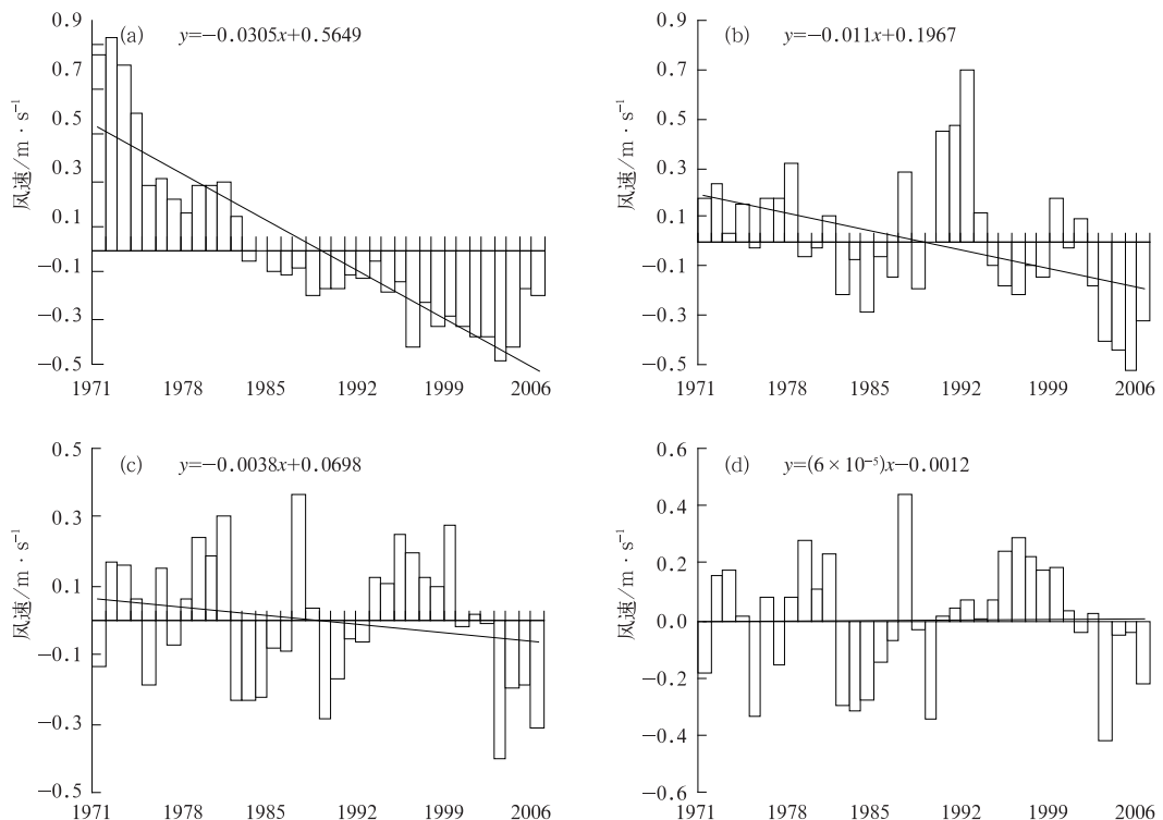
图 2 河北地区边界层内不同高度年平均风速距平变化 (a) 10m; (b) 300m; (c) 600m; (d) 900m。直线表示线性趋势
