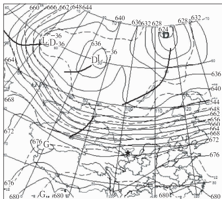
图3 2008年5月2日08时500hPa高空图 ★为沙尘暴区域
