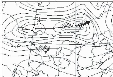
图4 2008年5月2日08时500hPa T213全风速数值预报产品图
