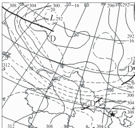
图5 2008年5月2日08时700hPa高空图 ★为沙尘暴区域
