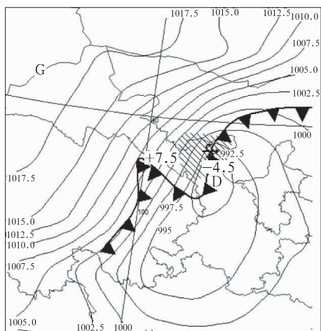
图6 2008年5月2日17时地面图
