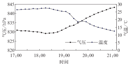
图 2 2008 年 5 月 2 日 17—21 时凉州地面自动站气压和气温变化曲线
