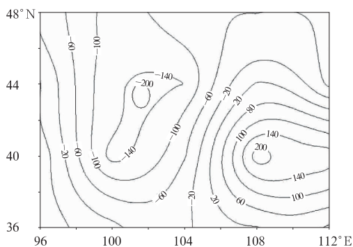
图 8 2008 年 5 月 2 日 14 时垂直螺旋度 单位: \text{m}^2 \cdot \text{s}^{-2}
