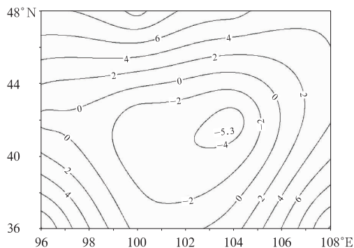
图 9 2008 年 5 月 2 日 08 时 \theta_{500-700} 分布图(单位: ^{\circ}\text{C} \cdot \text{m}^{-1} )
