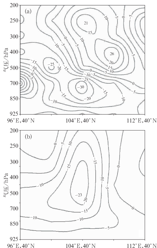
图7 2008年5月2日20时散度(a)和垂直速度(b)垂直剖面图 散度单位: 10^{-5}\text{s}^{-1} ,垂直速度单位: 10^{-3}\text{hPa}\cdot\text{s}^{-1}
