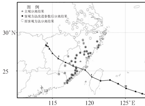
图 2 2005 年 08 月 31 日降水主客观分离结果对照图
