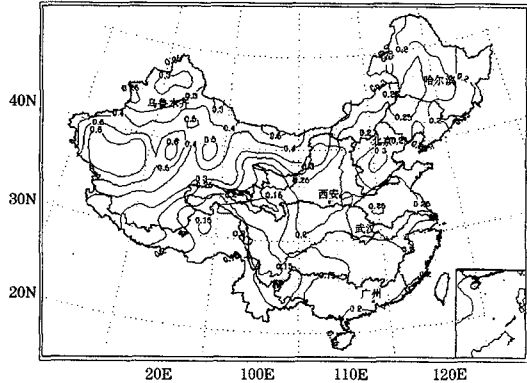
图2 中国年降水量变差系数分布(1971~2000年)
