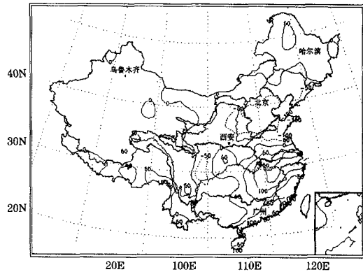
图3 中国年降水量变化趋势空间特征 (1980~2000年与1956~1979年年降水量之差)
