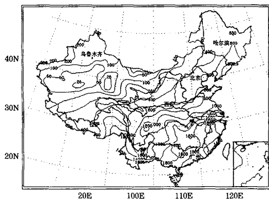
图1 中国年降水量分布(mm) (1971~2000年平均)
