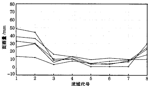
图2 2001年6月16日海河流域面雨量实况(无标记实线)与24小时指导预报(带叉实线)、T106(带空心圆)、HLAFS(带实心圆)及集成(带空心方框)
