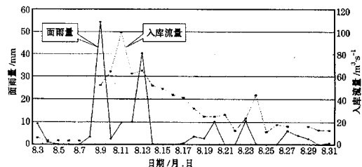
图4 2000年8月滦河流域面雨量与潘家口水库入库流量
