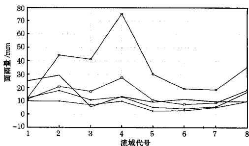
图3 2001年6月16日海河流域面雨量实况(无标记实线)与48小时指导预报(带叉实线)、T106(带空心圆)、HLAFS(带实心圆)及集成(带空心方框)
