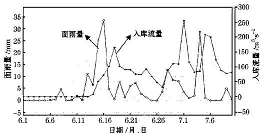
图5 2001年6~7月滦河流域面雨量与潘家口水库入库流量
