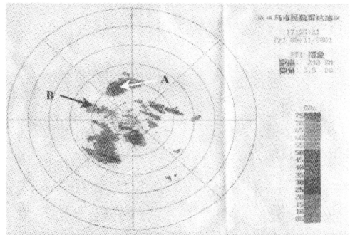
图 5a 2001 年 5 月 11 日 09 时 55 分仰角 2.5° 距离 240km 平显
