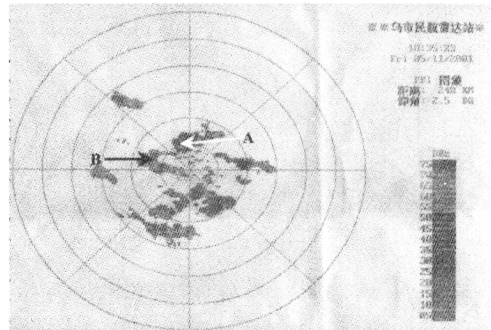
图 5b 2001 年 5 月 11 日 10 时 35 分仰角 2.5° 距离 240km 平显
