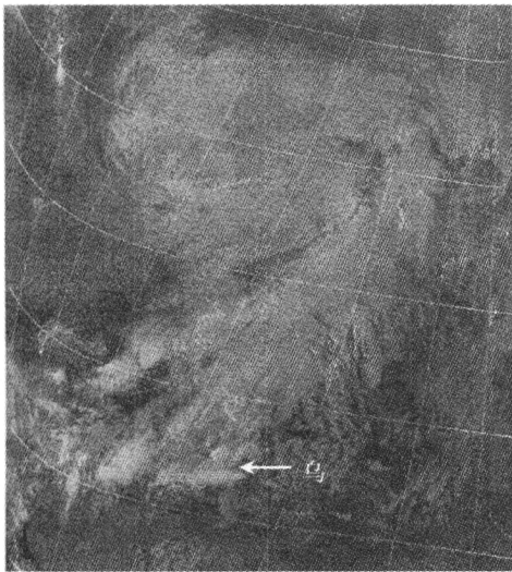
图 4 2001 年 5 月 11 日 NOAA-14 10:31 云图
