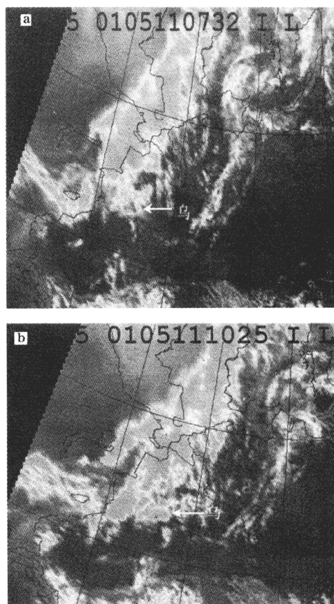
图3 2001年5月11日GMS-5卫星云图 (a)07:32,(b)10:25
