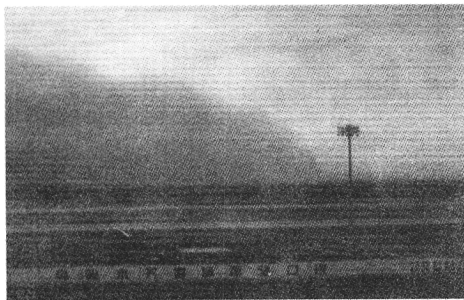
图 1 沙尘暴袭击乌鲁木齐机场
