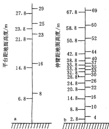
附图 西双版纳热带森林生态系统观测铁塔平台与伸臂距地面垂直高度/m 位置的示意图
