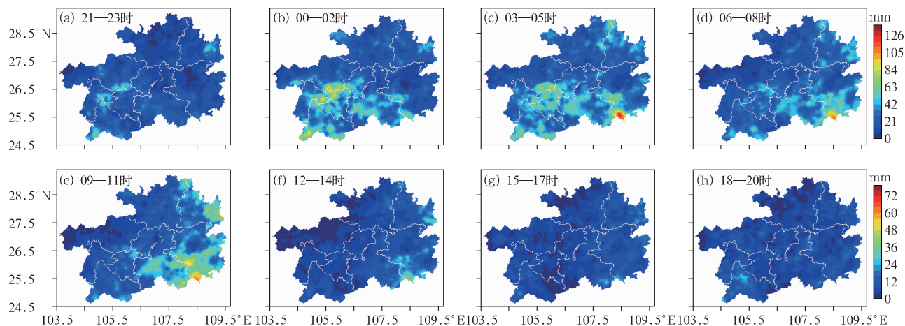
图 7 2010—2023 年汛期贵州年平均暴雨的逐 3 h 累计降水量空间分布
