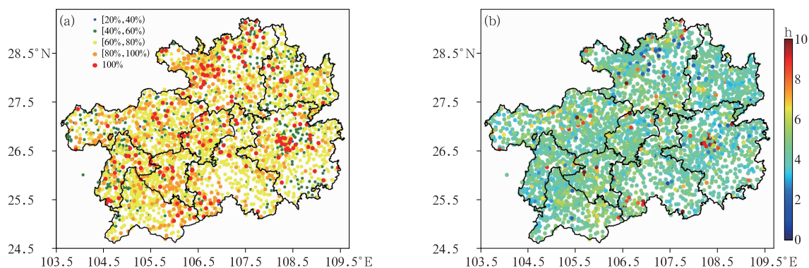
图 5 2010—2023 年汛期贵州暴雨(a)伴随短时强降水的占比和(b)降水持续时间空间分布
