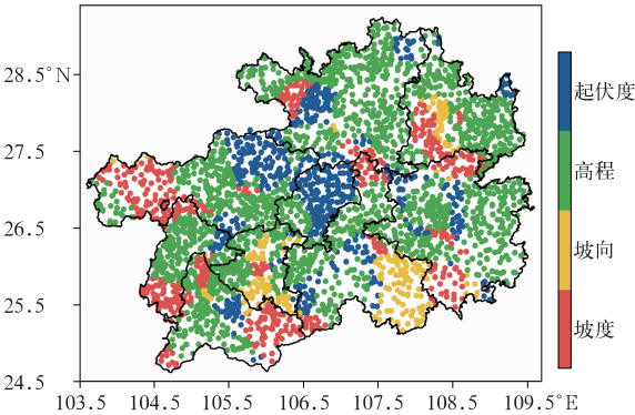
图 11 2010—2023 年汛期贵州各站点暴雨频次主导地形因子空间分布
