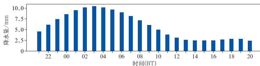
图 6 2010—2023 年汛期贵州暴雨平均小时降水量日变化
