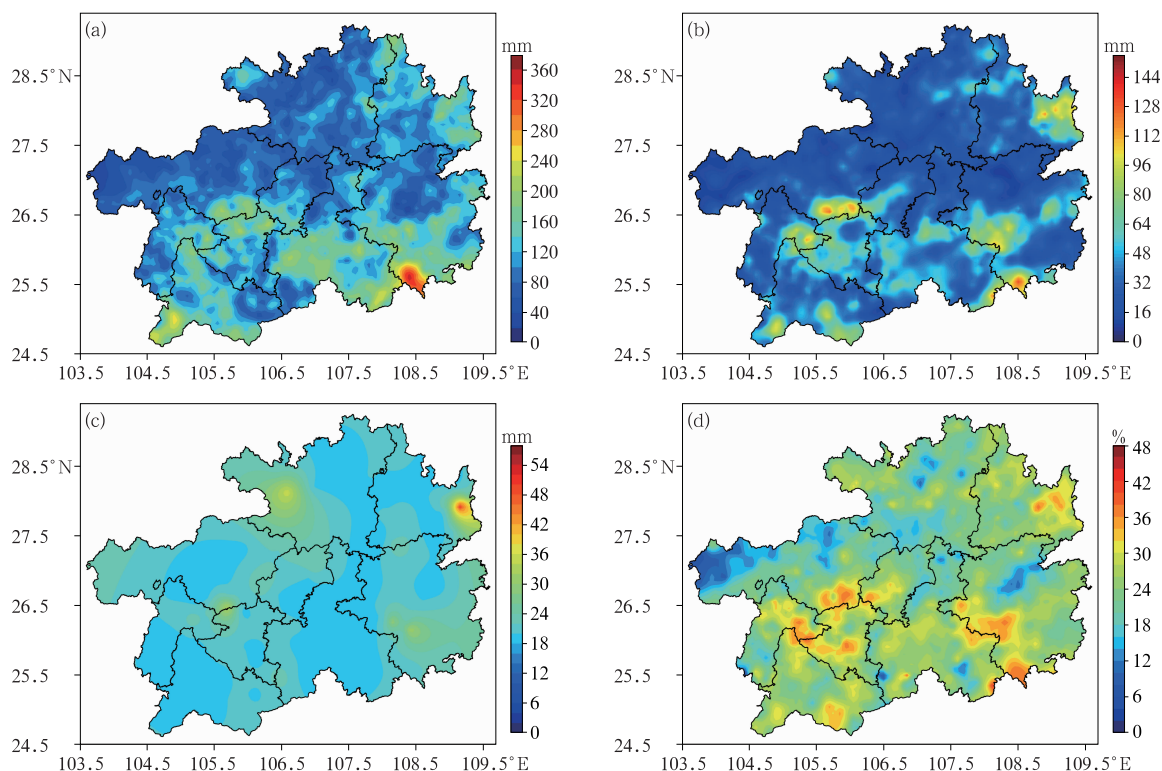
图 2 2010—2023 年汛期贵州年平均(a)暴雨,(b)大暴雨,(c)特大暴雨累计降水量和 (d)暴雨及以上降水占汛期总降水量比例的空间分布
