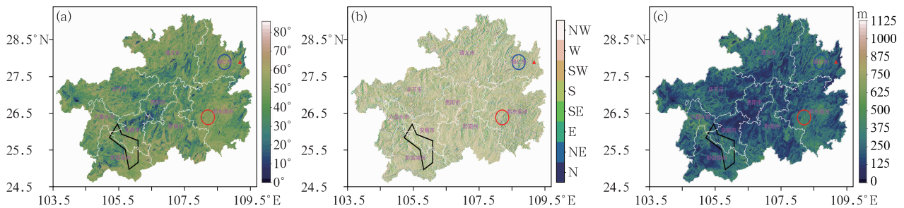
图1 贵州境内(a)坡度,(b)坡向及(c)地形起伏度空间分布
