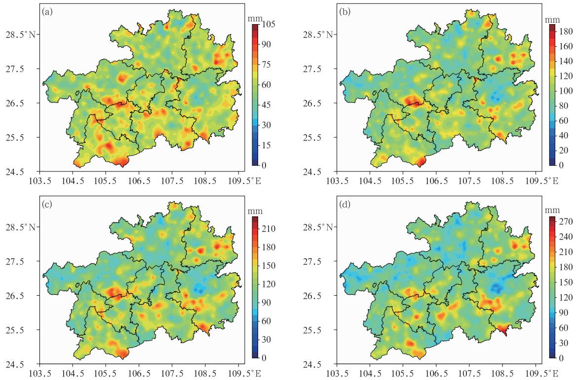
图3 2010—2023年汛期贵州年平均暴雨最大(a)1 h,(b)3 h,(c)6 h和(d)12 h降水量空间分布
