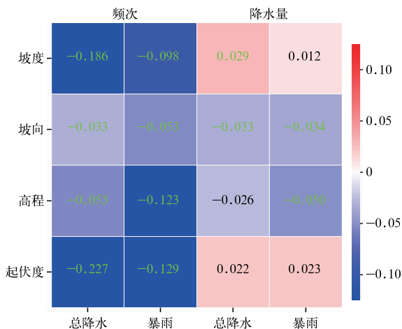
图 10 2010—2023 年汛期贵州总降水、暴雨的降水频次、降水量与各地形因子的相关系数
