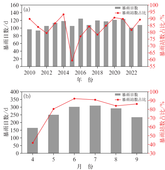
图4 2010—2023年汛期贵州暴雨日数、暴雨站数占比的(a)年变化及(b)月变化分布
