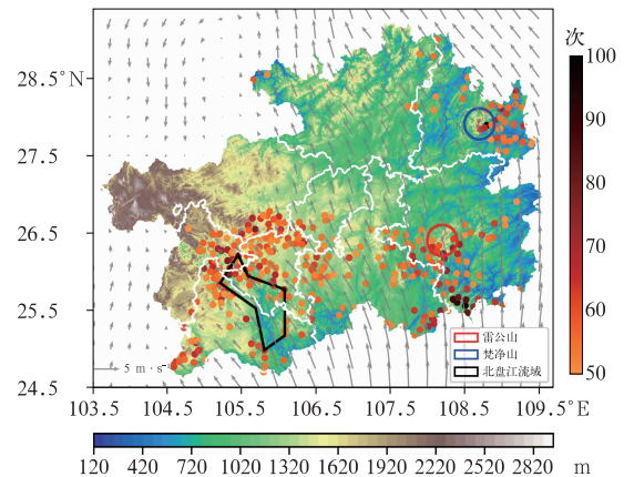
图9 2010—2023年汛期贵州暴雨量级降水频次(彩色圆点),850 hPa气候平均风场(风矢)以及地形高程(填色)分布
