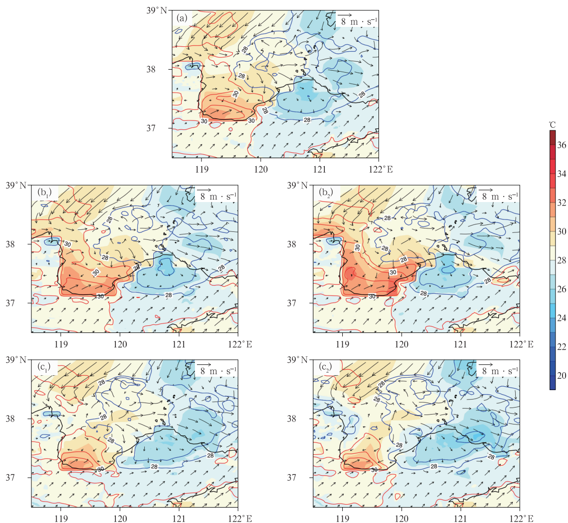
图7 2022年8月8日04时莱州湾地区(a)CTRL,(b 1 )SST+1,(b 2 )SST+2,(c 1 )SST-1,(c 2 )SST-2试验的地表温度(填色)、2 m气温(等值线,间隔1℃)和10 m风场(风矢)的分布
