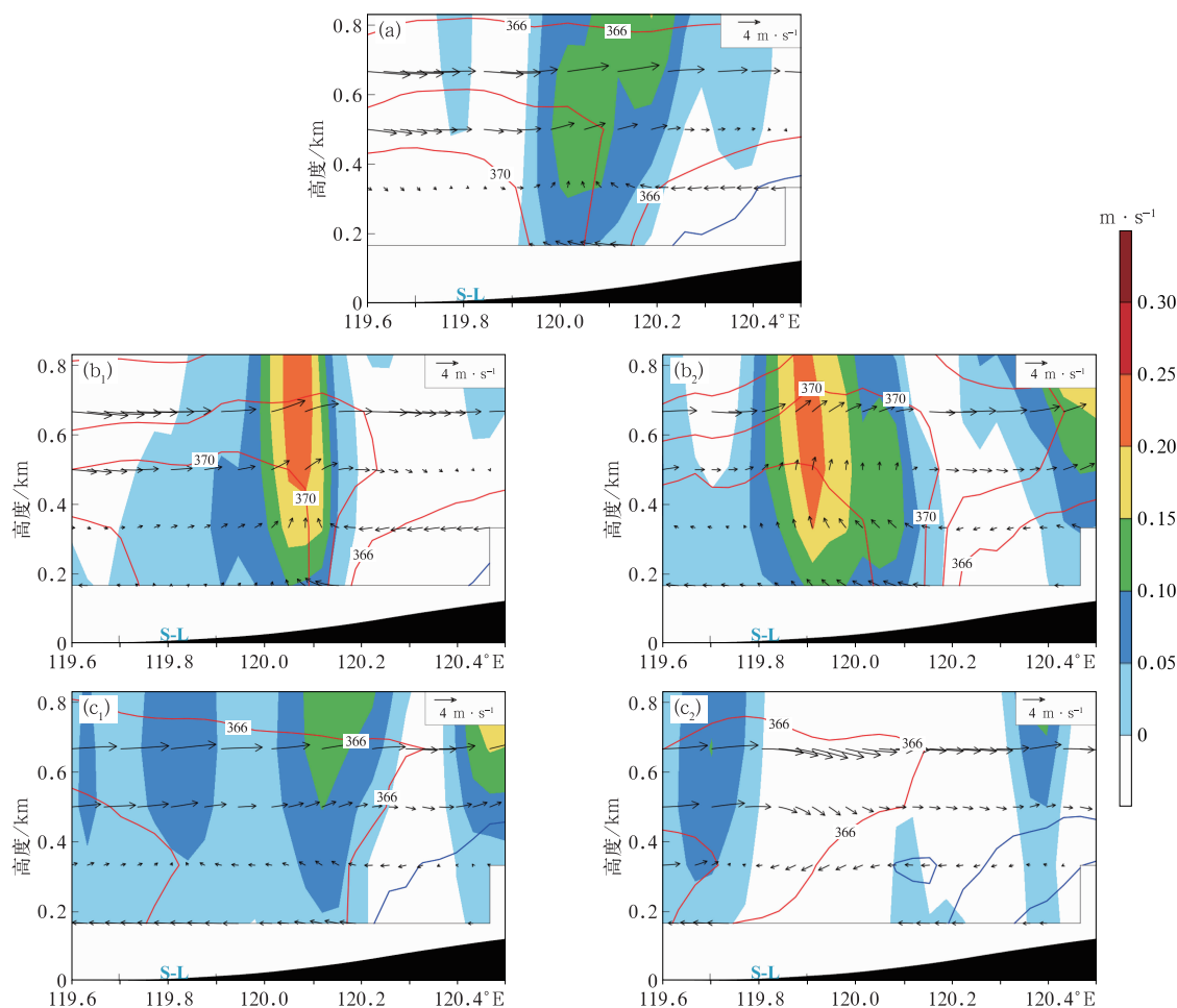
图 8 2022 年 8 月 8 日 05 时(a)CTRL, (b 1 )SST+1, (b 2 )SST+2, (c 1 )SST-1, (c 2 )SST-2 试验 u-w 风场(风矢,垂直速度扩大 10 倍)、相当位温(等值线,单位:K)和垂直速度(填色)沿 37.4°N 的垂直剖面
