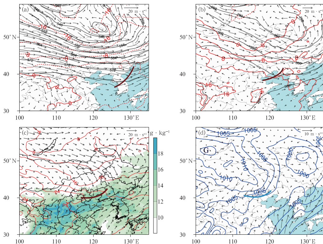
注:图 a 中棕色线代表槽线, b、c 中棕色线代表切变线,图 d 中粗蓝色线代表冷锋。
