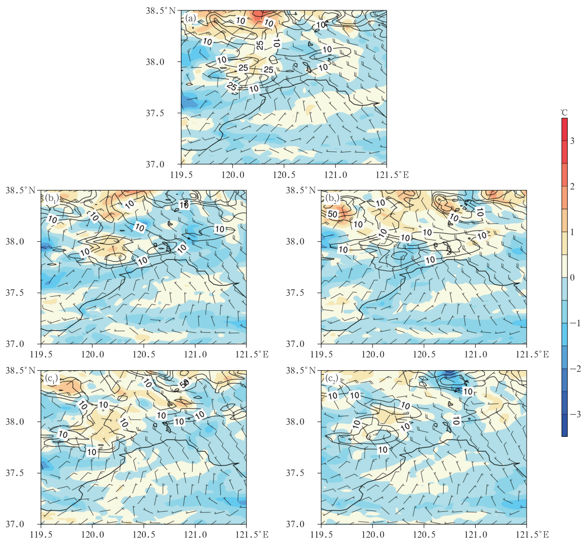
图9 2022年8月8日05时莱州湾东侧沿岸附近(a)CTRL, (b 1 )SST+1, (b 2 )SST+2, (c 1 )SST-1, (c 2 )SST-2试验风场(风羽)、2 m变温(填色)和1 h累计降水量(等值线,取值10、25、50 mm)的分布
