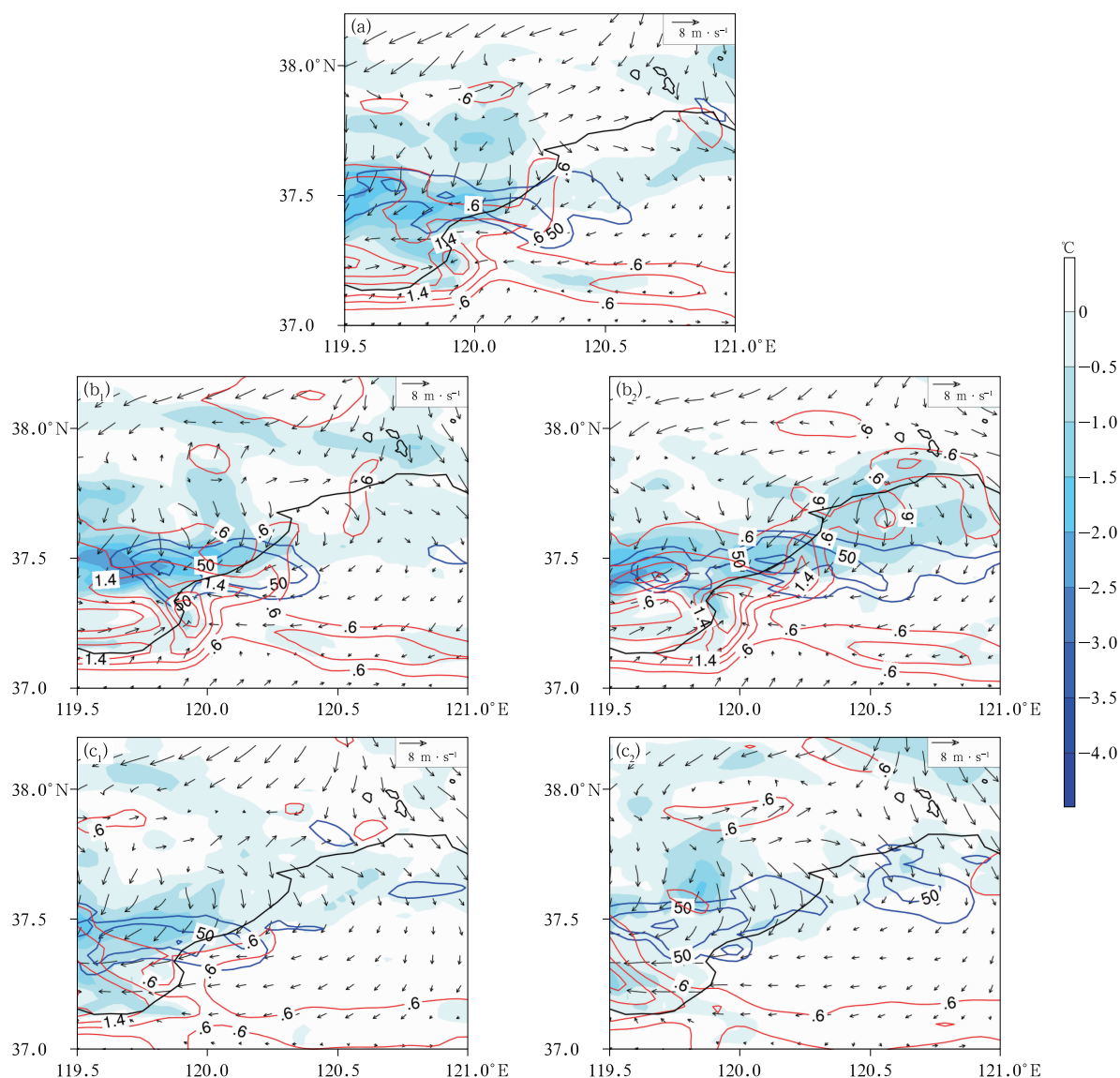
图 10 2022 年 8 月 8 日 06—07 时莱州湾东侧沿岸附近平均温度梯度(红色等值线,单位: 10^{-4} \text{ }^{\circ}\text{C} \cdot \text{m}^{-1} )、风场(风矢)、2 m 变温(填色)和 07—08 时累计降水量(蓝色等值线,取值 25、50、100 mm)的分布 (a)CTRL, (b 1 ) SST+1, (b 2 ) SST+2, (c 1 ) SST-1, (c 2 ) SST-2
