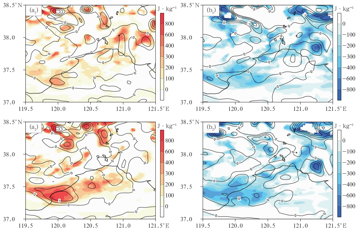
图 6 2022 年 8 月 8 日 04 时莱州湾东侧沿岸附近 (a 1 )SST+1, (a 2 )SST+2, (b 1 )SST-1, (b 2 )SST-2 试验与 CTRL 试验的 CAPE(填色)
