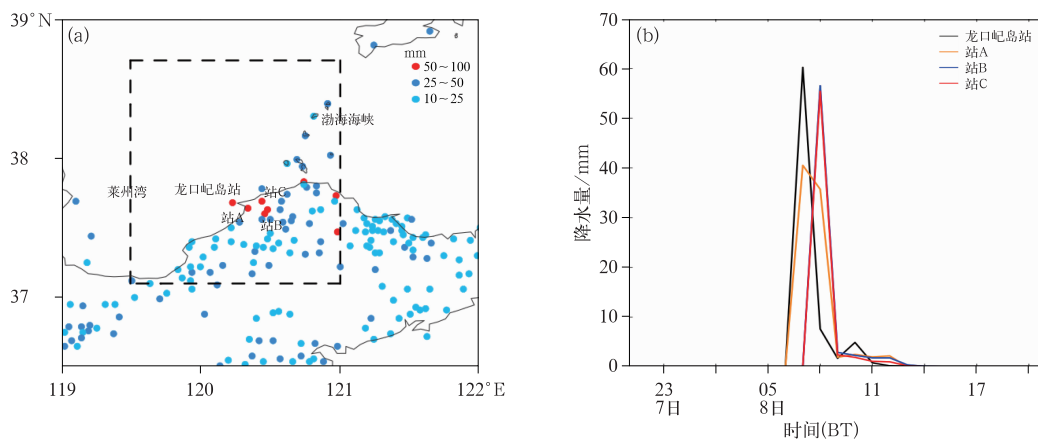
图1 2022年8月7日20时至8日20时莱州湾东侧沿岸附近(a)累计降水量分布及(b)代表站逐小时降水量时间序列
