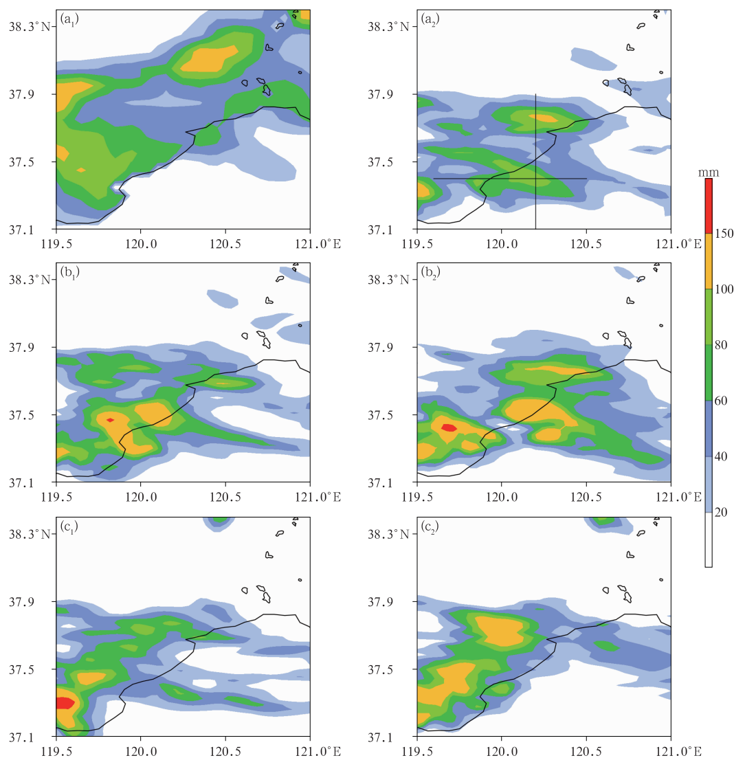
注:图 a_2 中横、竖黑色实线(分别对应 37.4^\circ\text{N} 和 120.2^\circ\text{E} )分别为图 8、图 11 垂直剖面所在位置。
