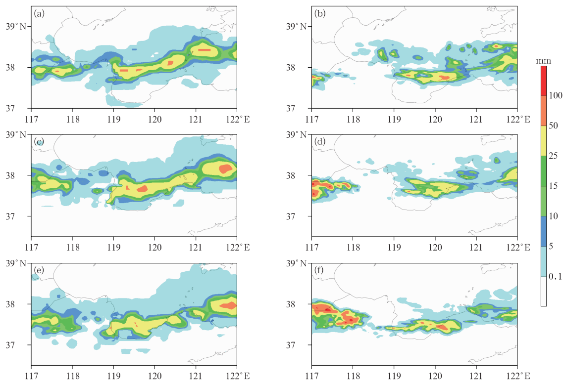
图 4 莱州湾地区 2022 年 8 月 8 日 (a,b)06 时,(c,d)07 时,(e,f)08 时
