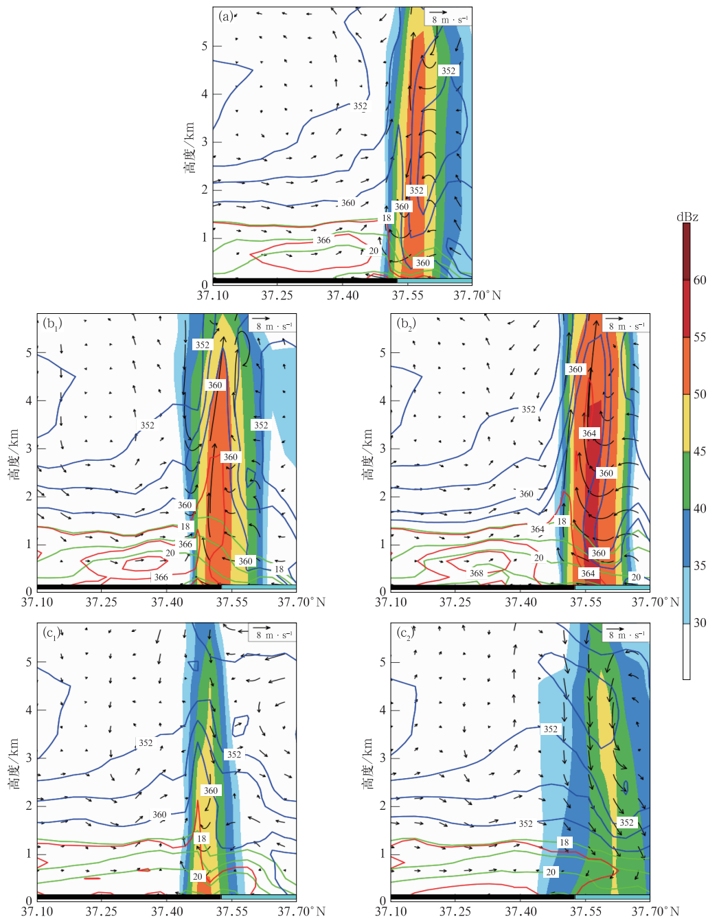
图 11 2022 年 8 月 8 日 07 时相当位温(红色、蓝色等值线,单位:K)、比湿(绿色等值线,单位: \text{g} \cdot \text{kg}^{-1} )、反射率因子(填色)、 v-w 风场(箭头,垂直速度扩大 10 倍)沿 120.2^\circ\text{E} 的垂直剖面 (a)CTRL, (b 1 )SST+1, (b 2 )SST+2, (c 1 )SST-1, (c 2 )SST-2
