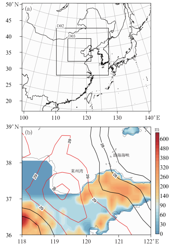
图 3 (a)模拟区域示意图,(b)莱州湾地区地形(填色)及基于 ERA5 资料的 2022 年 8 月 7 日 20 时的地表温度(等值线,单位: ^{\circ}\text{C} )
