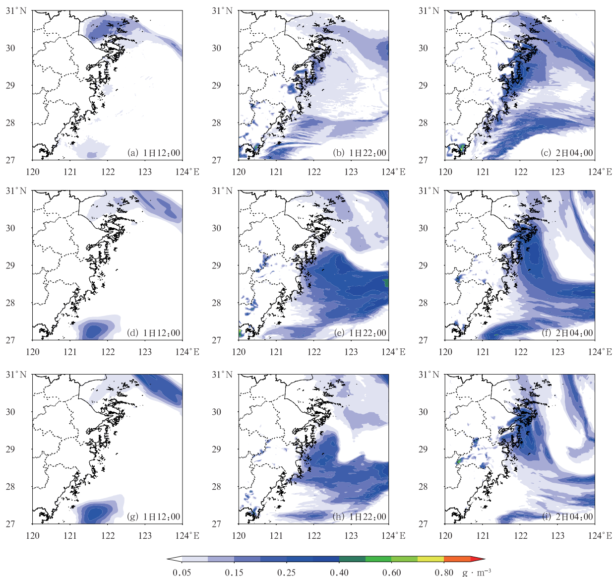
图7 浙江东部沿海及海面 2021 年 4 月 1 日 12:00、22:00 和 2 日 04:00(a~c)IAP-LACS, (d~f)Morrison05, (g~i)Thompson08 模拟的云水含量
