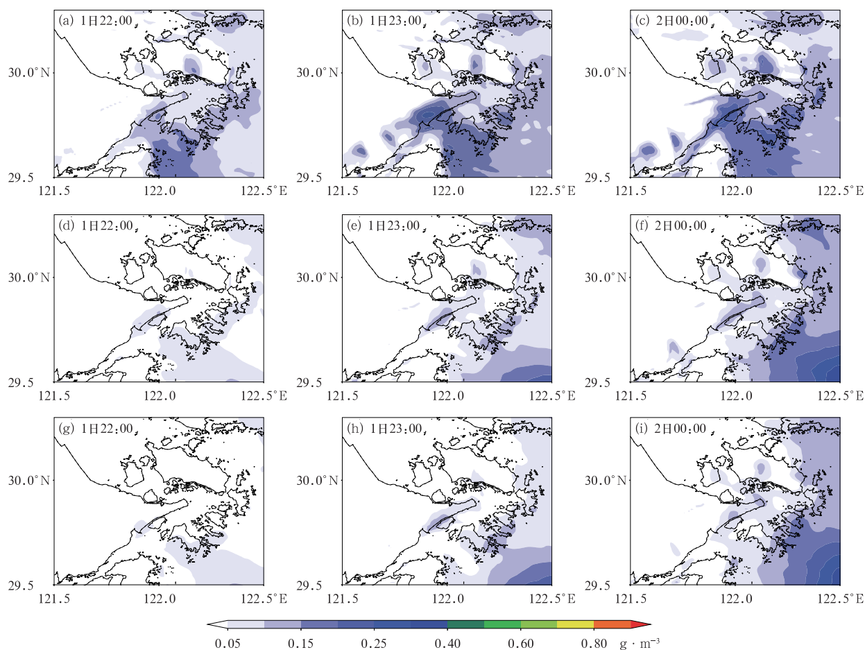
图9 2021年4月1日22:00、23:00和2日00:00(a~c)IAP-LACS, (d~f)Morrison05,(g~i)Thompson08 模拟的北仑舟山港附近云水含量
