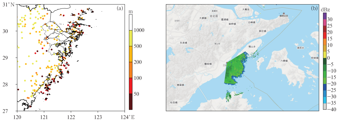
图 2 2021 年 4 月(a)1 日 08:00 至 2 日 08:00 自动站观测的最小能见度和 (b)2 日 00:00 毫米波雷达观测回波强度 Fig. 2 (a) Minimum visibility observations of automatic weather stations from 08:00 BT 1 to 08:00 BT 2 and (b) echo intensity observation of millimeter-wave radar at 00:00 BT 2 April 2021
