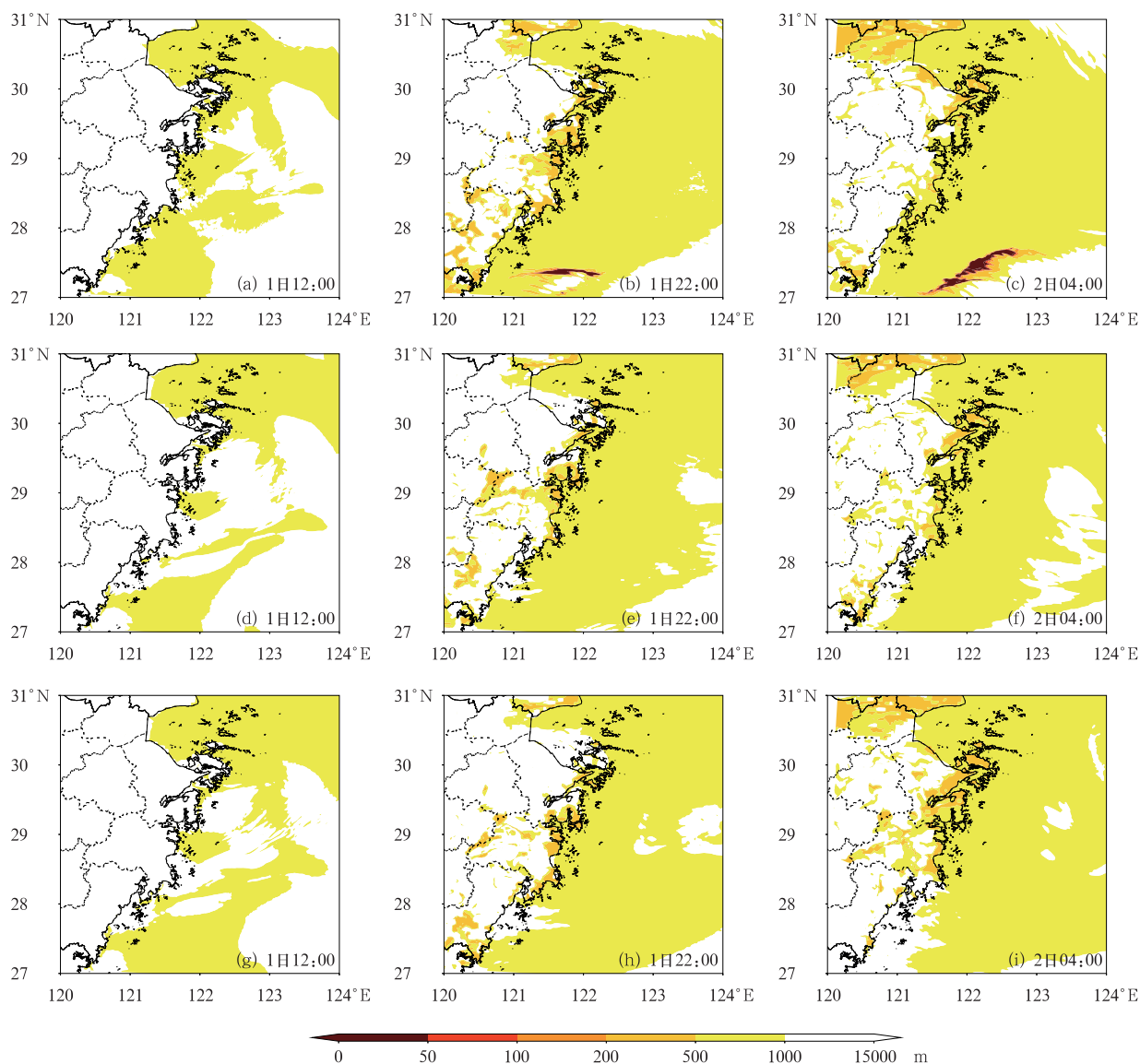
图 6 基于 FSL 诊断的浙江东部沿海及海面 2021 年 4 月 1 日 12:00、22:00 和 2 日 04:00
