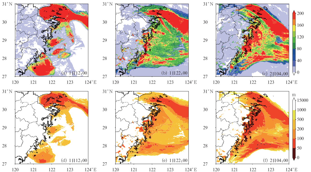
图 11 浙江东部沿海及海面 2021 年 4 月 (a, d) 1 日 12:00、(b, e) 1 日 22:00 和 (c, f) 2 日 04:00 (a~c) IAP-LACS 试验模式近地层云滴数浓度 (单位: \text{cm}^{-3} ) 和 (d~f) IAP-LACS 试验基于 Gultepe 方法的能见度诊断结果
