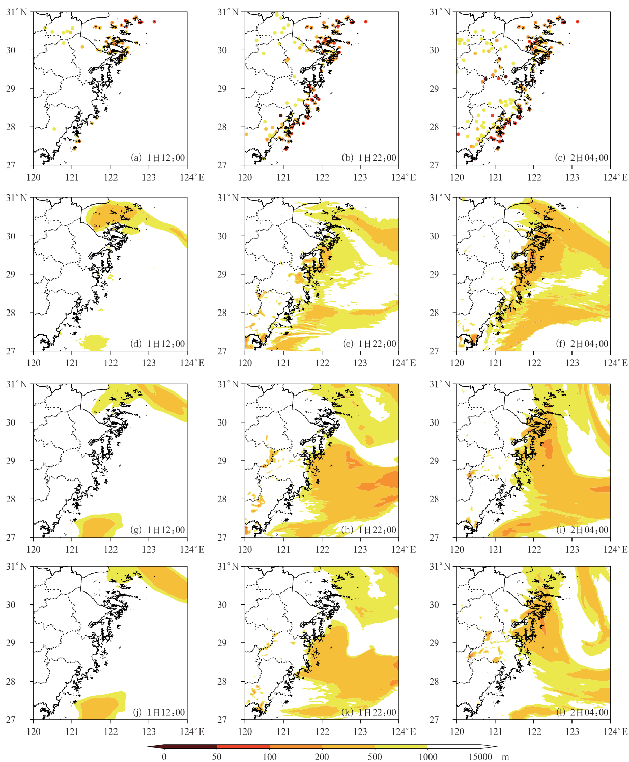
图 5 基于 SW99 诊断的浙江东部沿海及海面 2021 年 4 月 1 日 12:00、22:00 和 2 日 04:00(a~c)自动站能见度观测,及(d~f)IAP-LACS、(g~i)Morrison05、(j~l)Thompson08 能见度模拟
