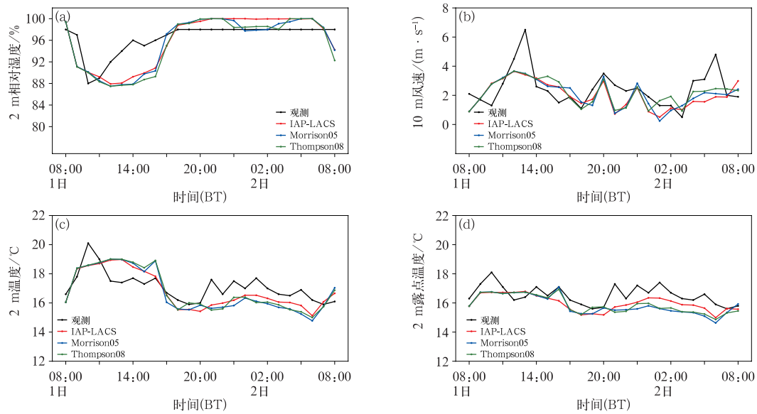
图 10 2021 年 4 月 1 日 08:00 至 2 日 08:00 玉环站观测和各组试验模拟的 (a) 2 m 相对湿度, (b) 10 m 风速, (c) 2 m 温度, (d) 2 m 露点温度对比
