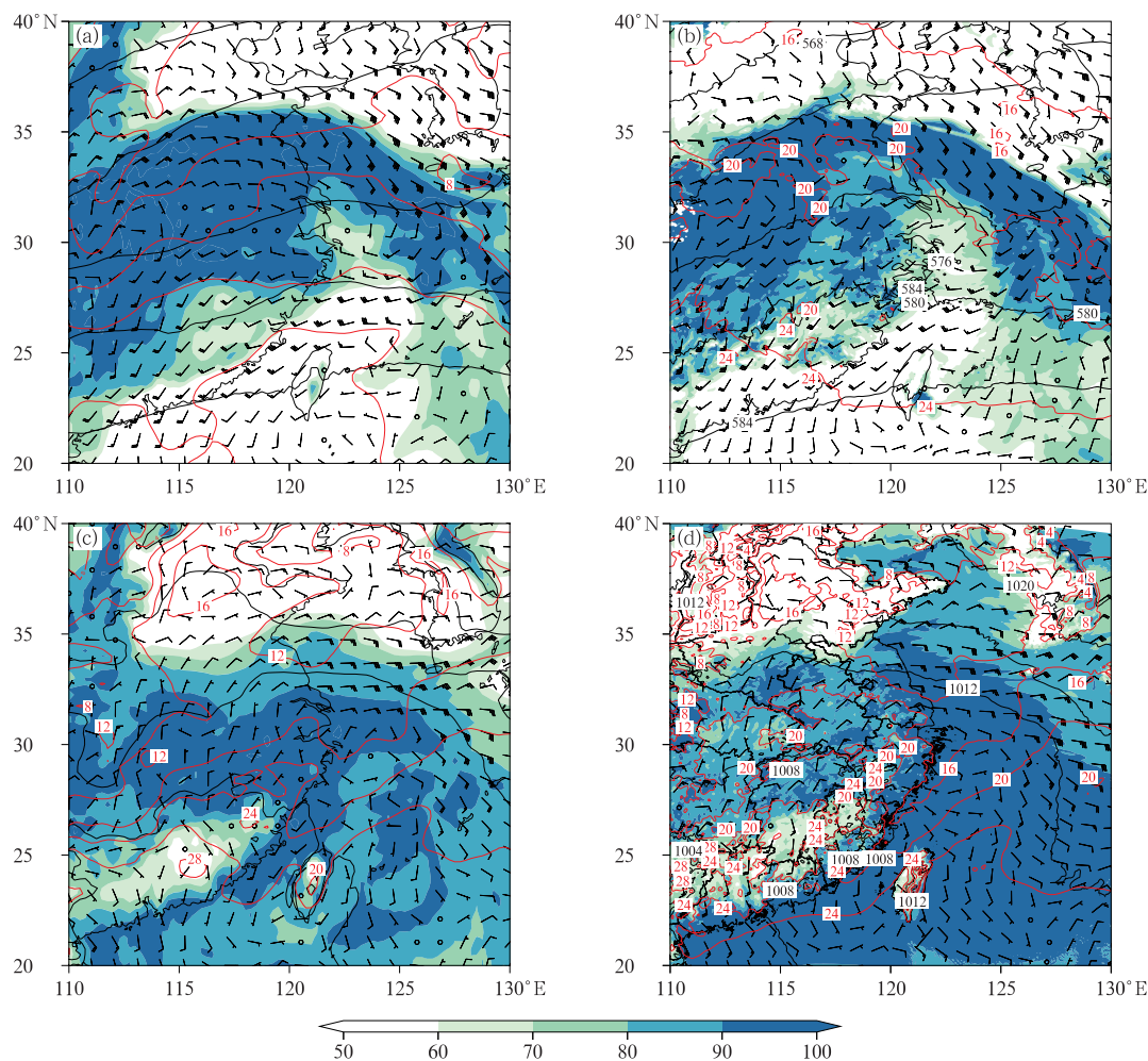
图3 2021年4月1日20:00基于(a,c)ERA5再分析资料和(b,d)IAP-LACS模拟的(a,b)500 hPa位势高度(黑色等值线,单位:dagpm),850 hPa气温(红色等值线,单位: ^{\circ}\text{C} )、相对湿度(填色,单位:%)和风场(风羽)与(c,d)地面气压(黑色等值线,单位:hPa)、2 m气温(红色等值线, ^{\circ}\text{C} )、2 m相对湿度(填色,单位:%)和风场(风羽)
